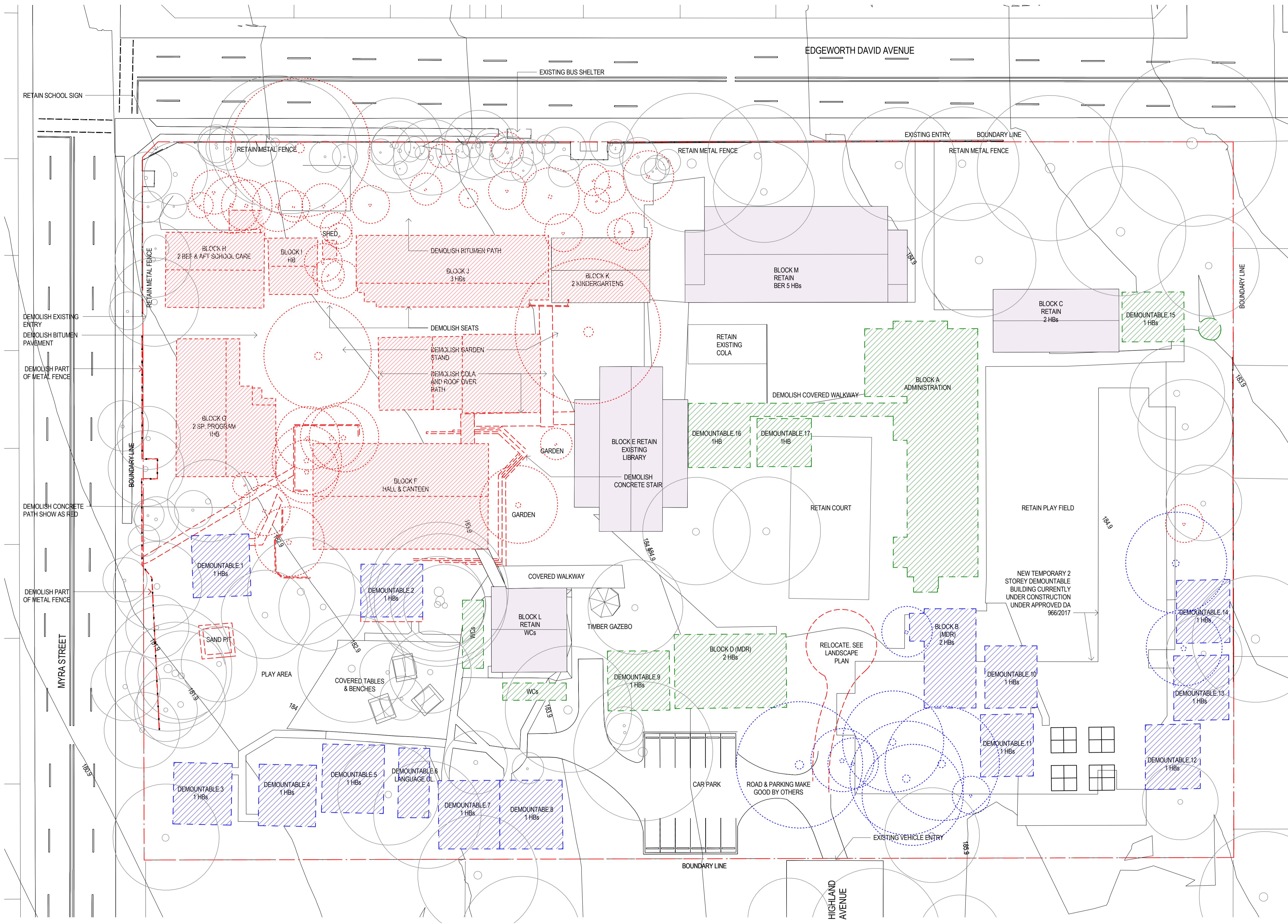
1 Site Demolition Plan 1 : 300
