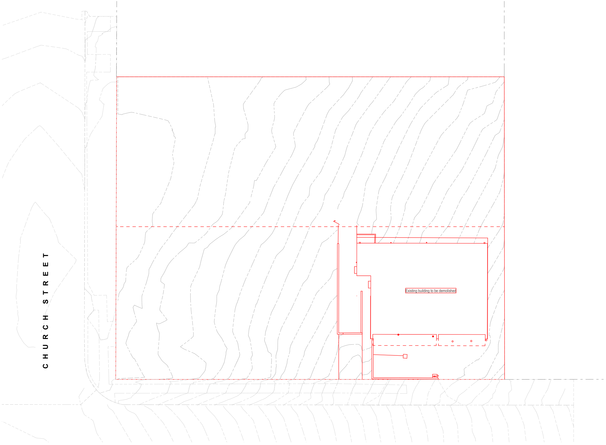
200 Demoliton Plan 1:250
