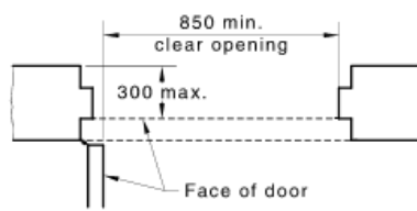
(a) Swing door
