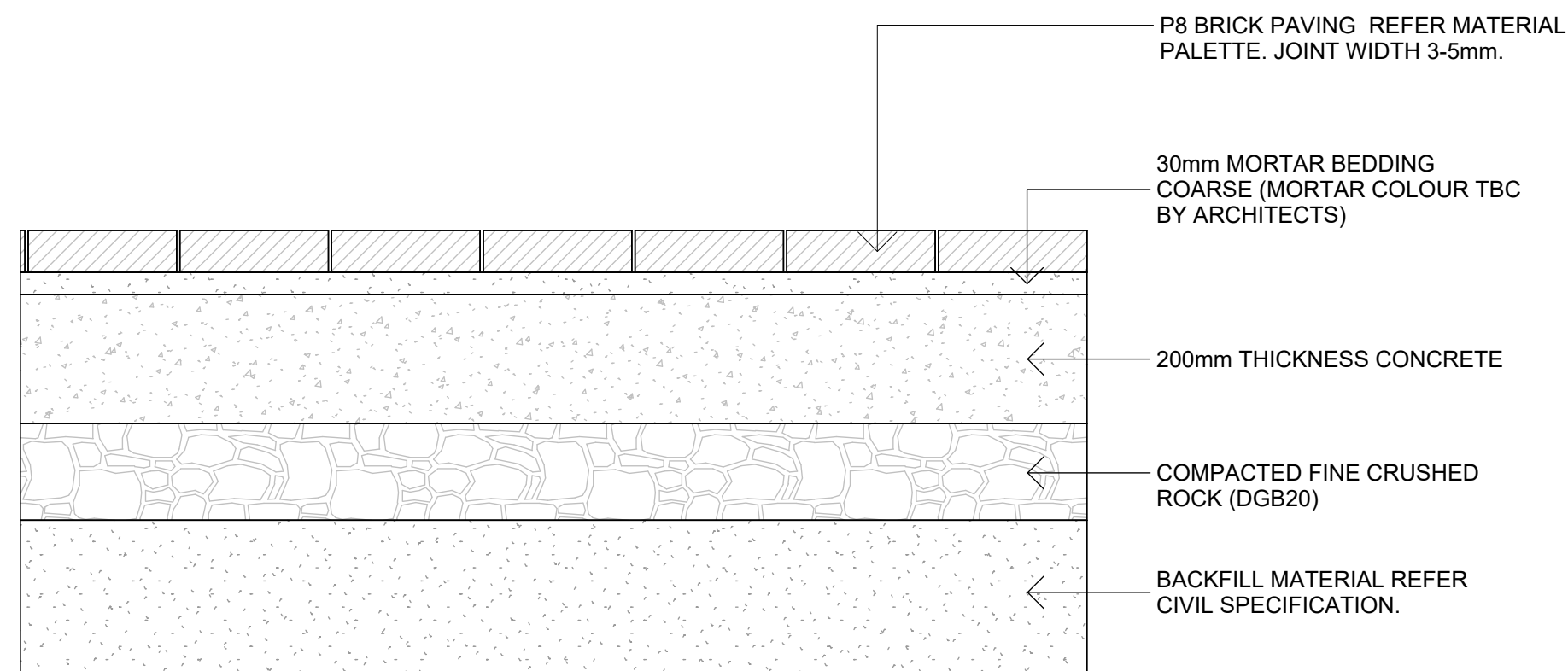
6 P8 - BRICK PAVER 1 : 10
