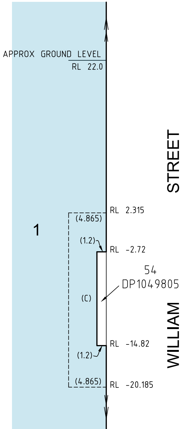
SECTION A-A 1:300
