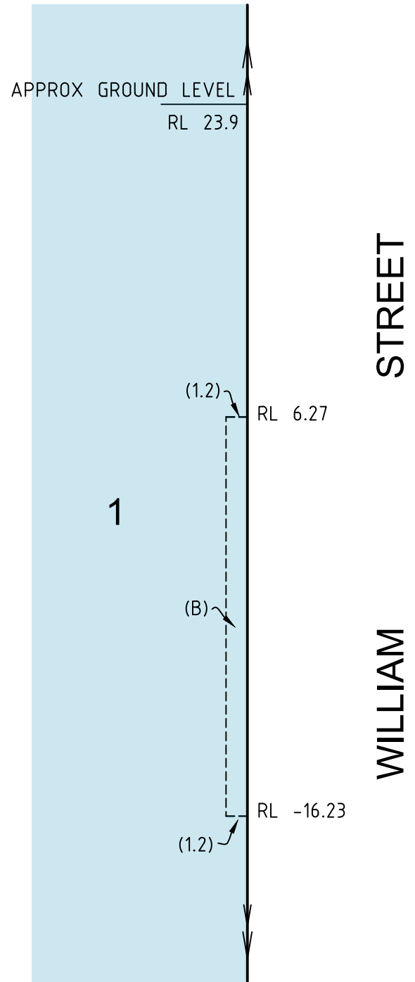
SECTION D-D 1:300
