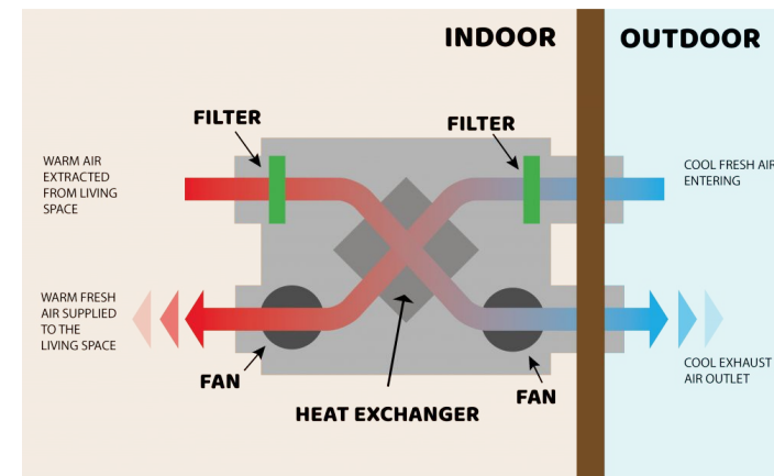
Image of a perroom mini HRV unit
