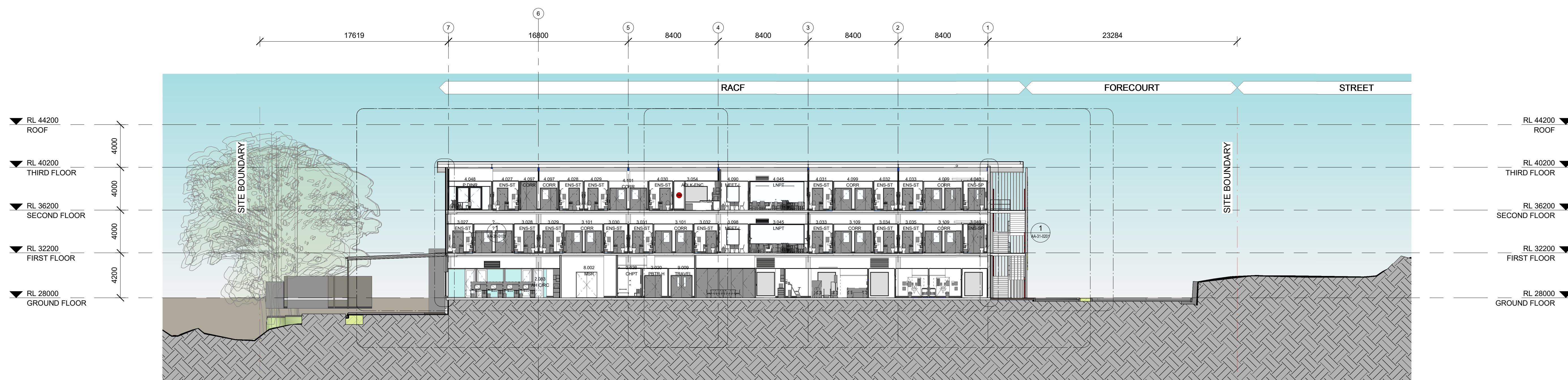
1 DA SECTION - BB 1 : 200
