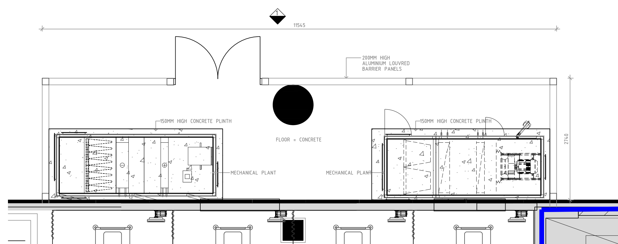
PLAN SCALE 1:50 @A1
