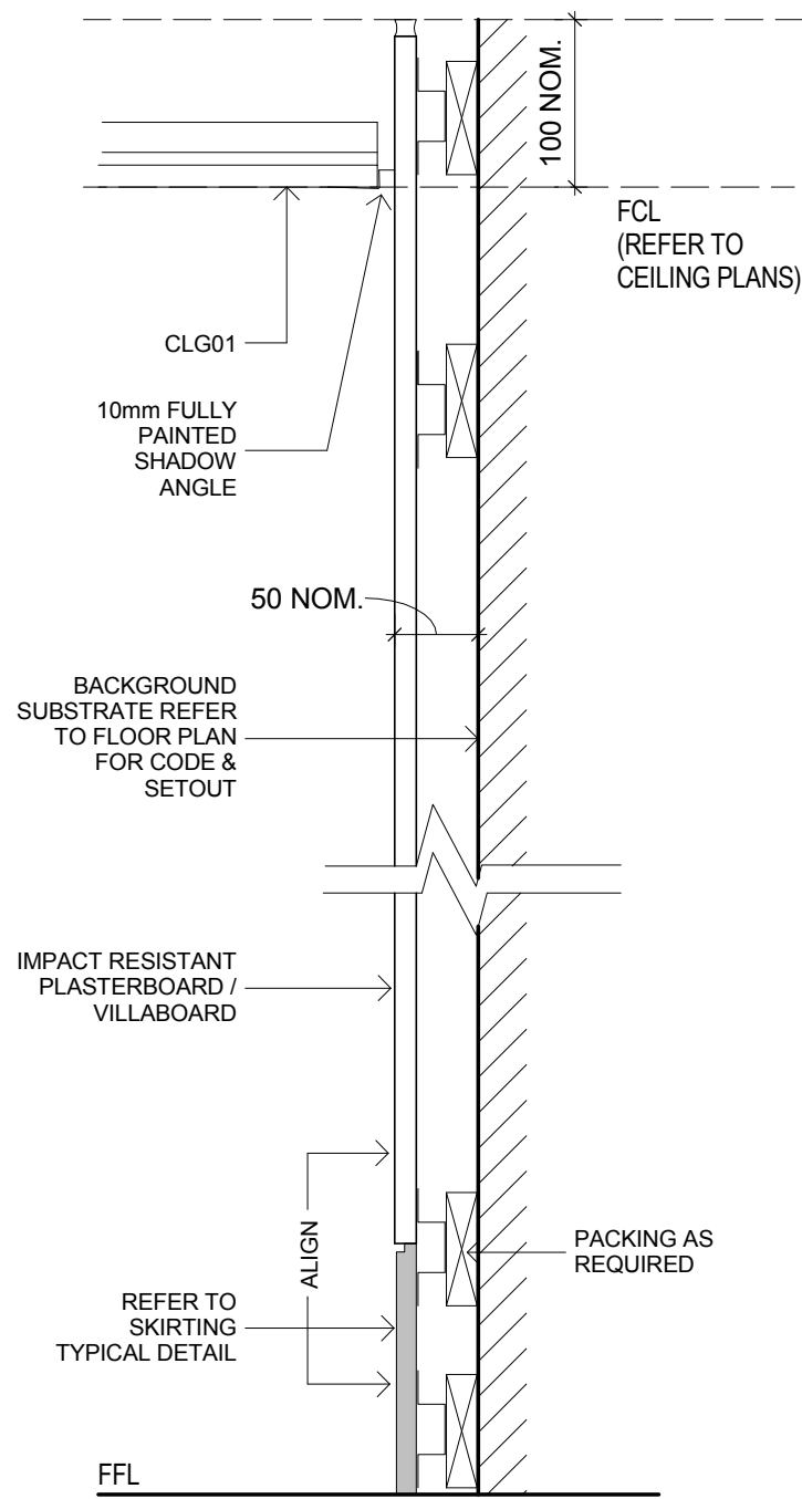
1 PT01-DETAIL SECTION 1:5
