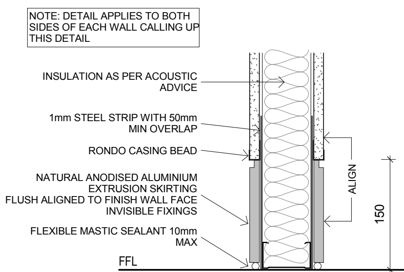
1 PT01-DETAIL SECTION 1:5
