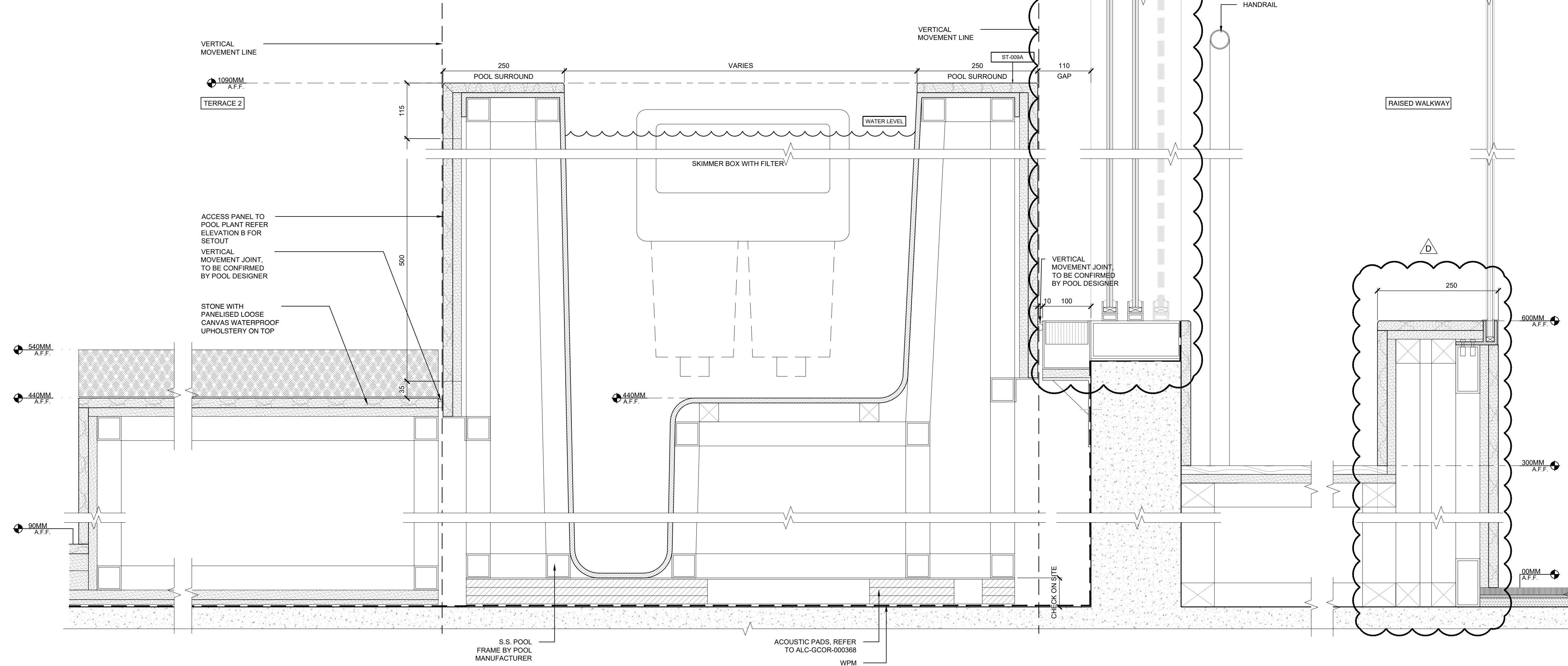
1 SECTION A-A SCALE:1:5
