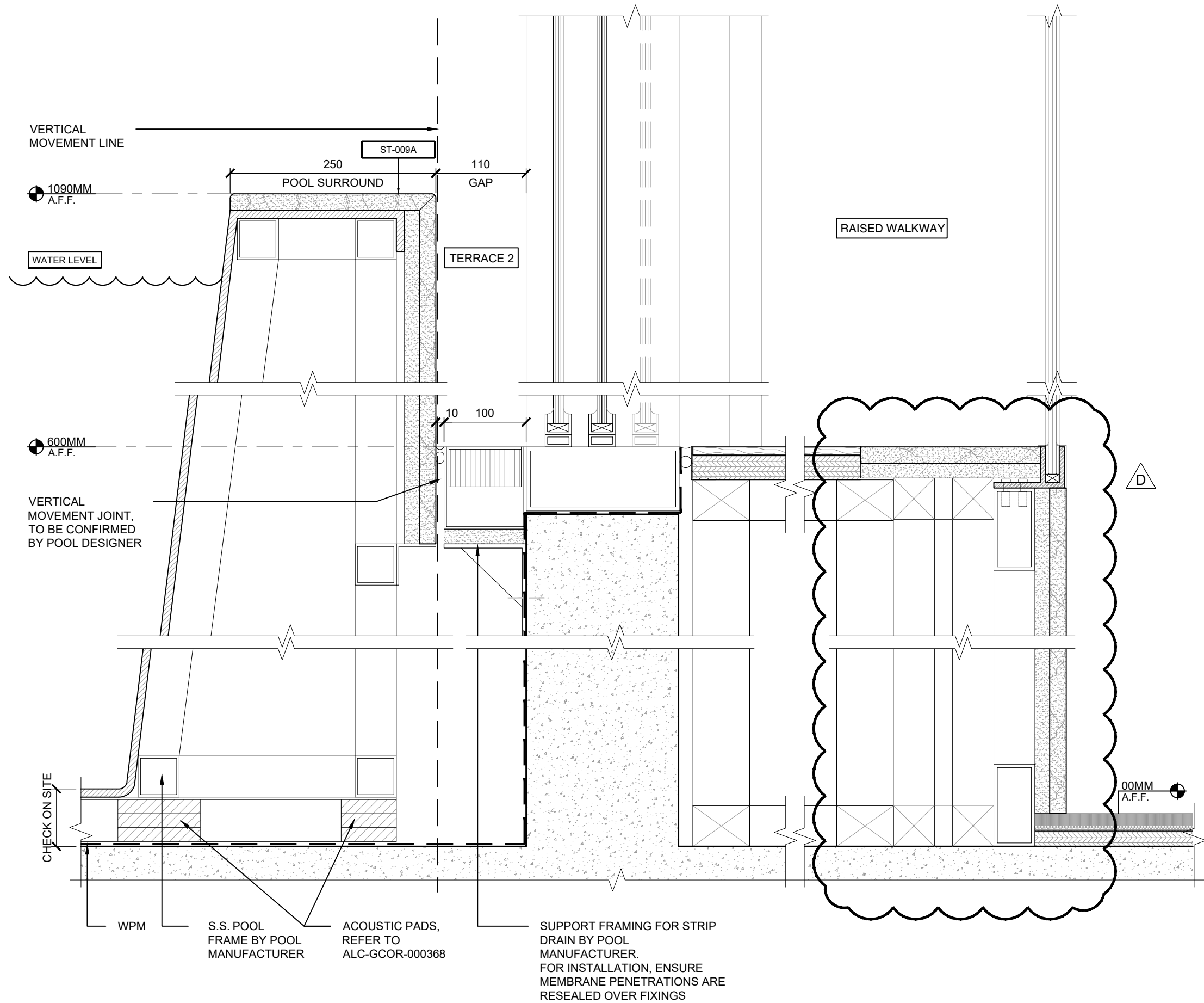
1 SECTION A-A SCALE:1:5
