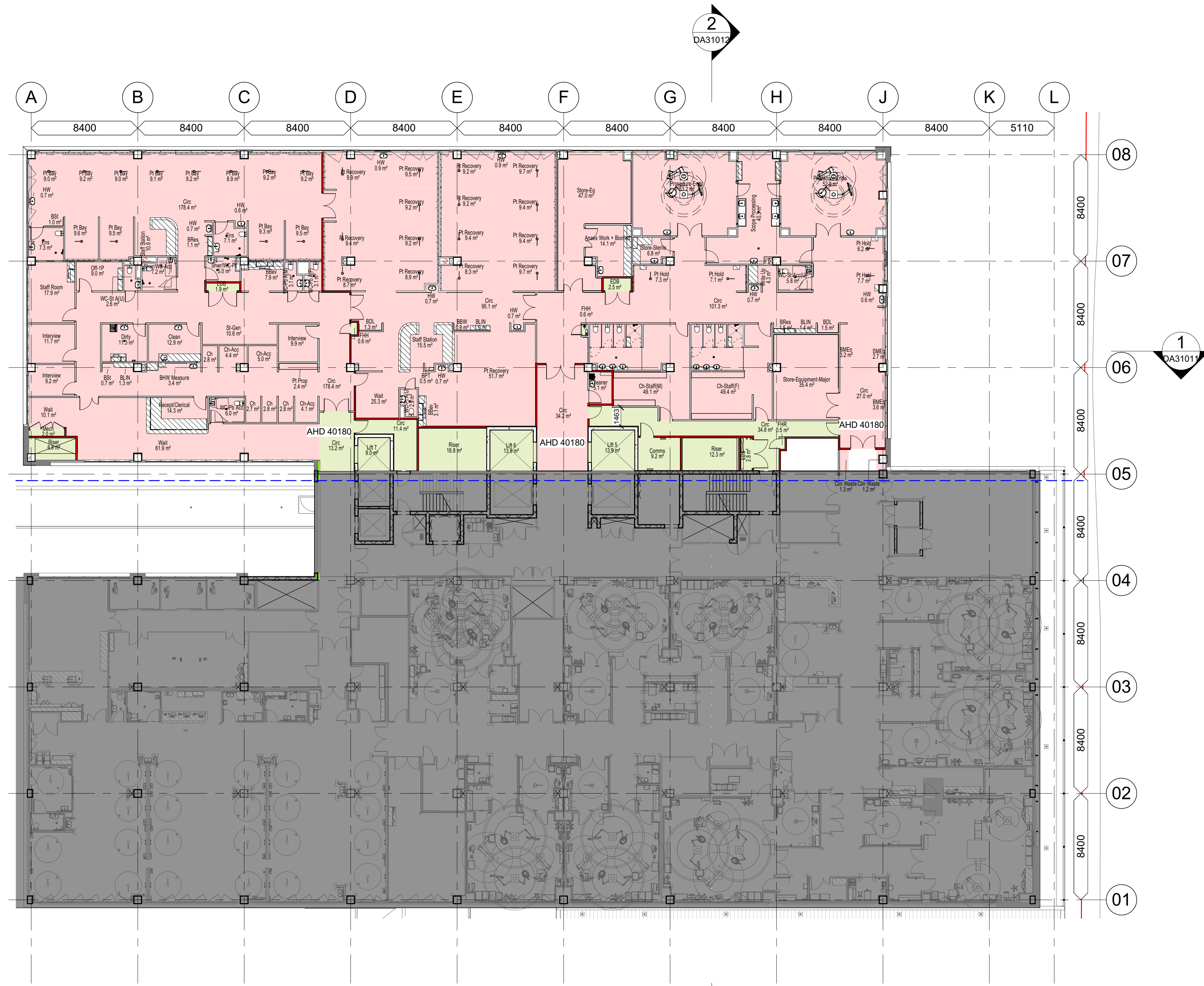
1 GA - Level 06 3B2 A30001 1 : 200
