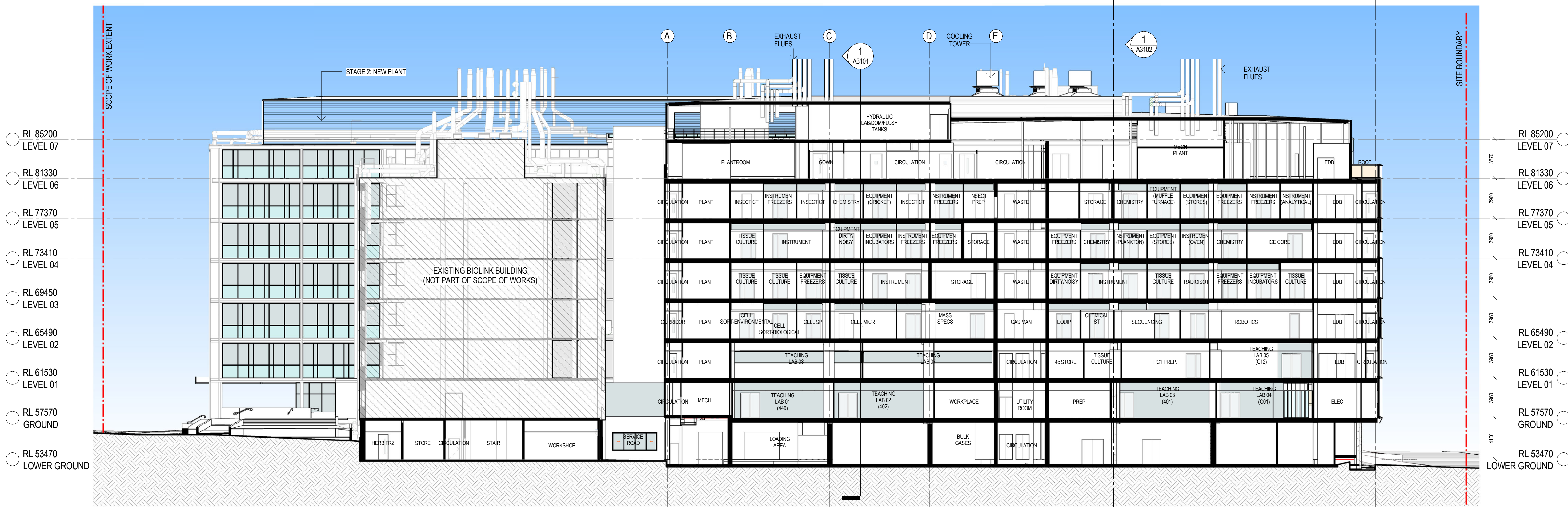
2 SECTION B (SSD) SCALE 1 : 200
