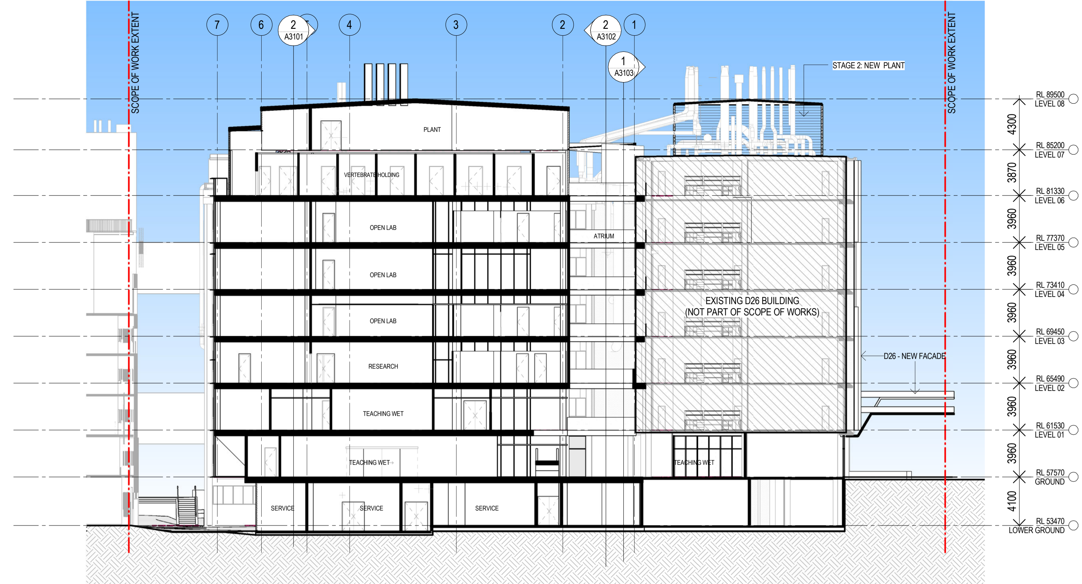
1 SECTION A SCALE 1 : 200
