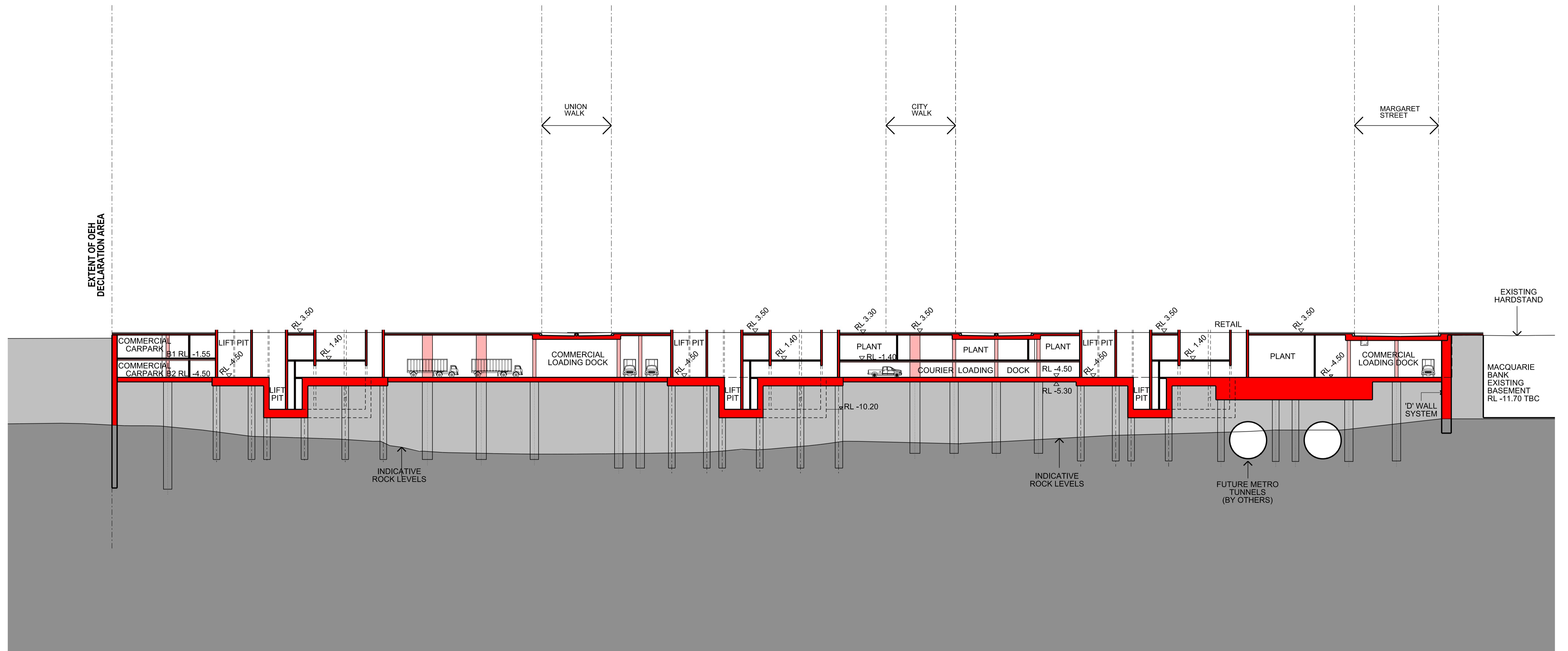
LONGITUDINAL SECTION 2-2
