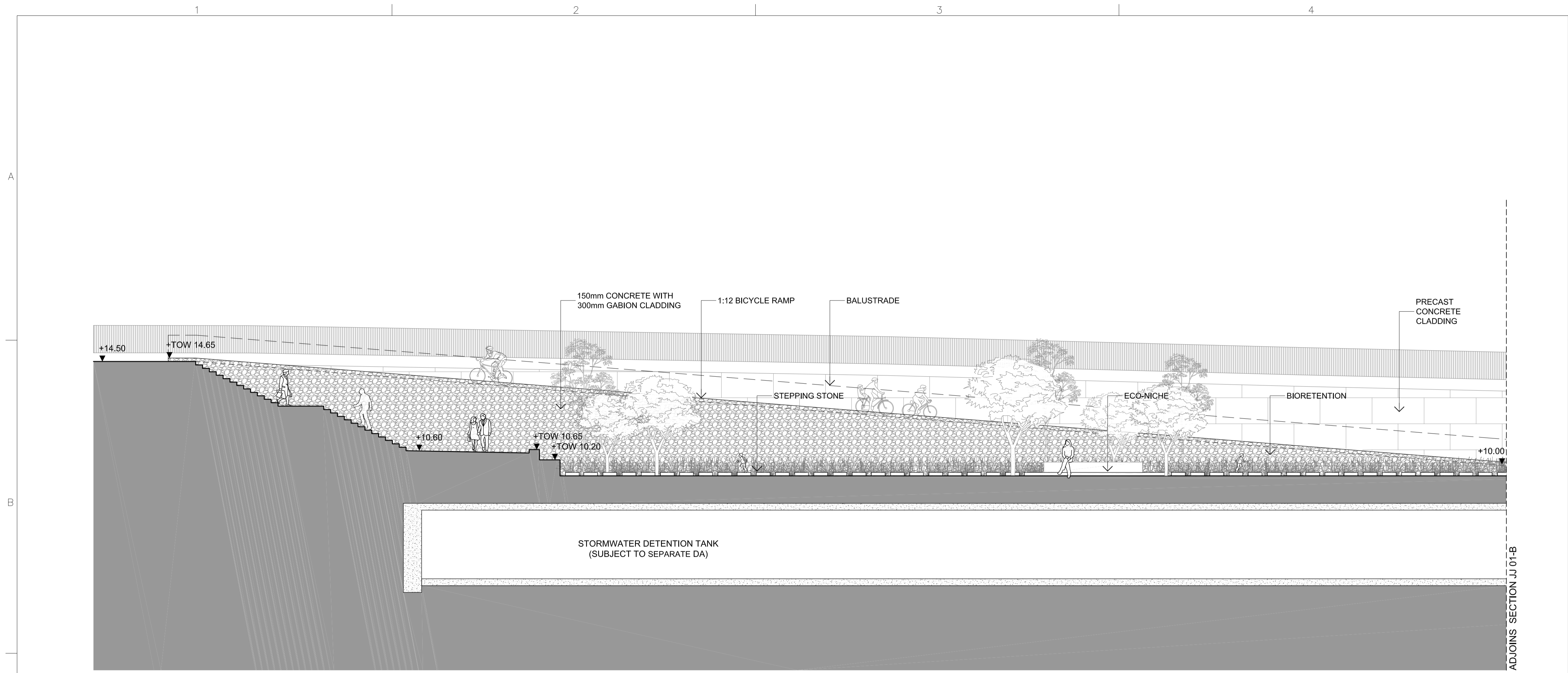
1 SECTION JJ 01-A SCALE - 1:100 @ A1 1:200 @A3
