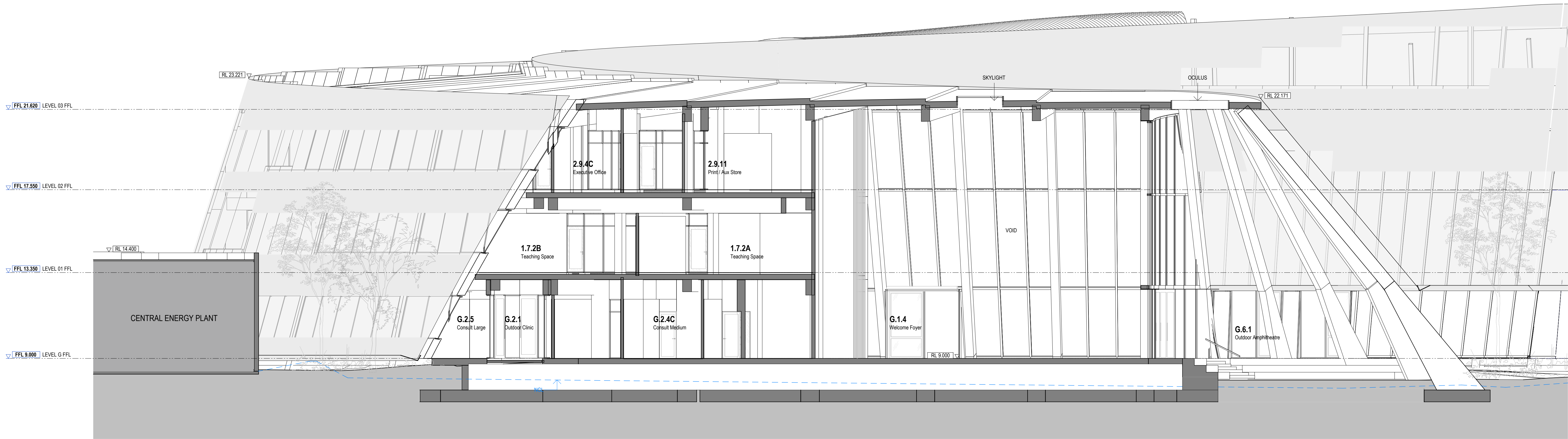
1 DA SECTION 7 1 : 100
