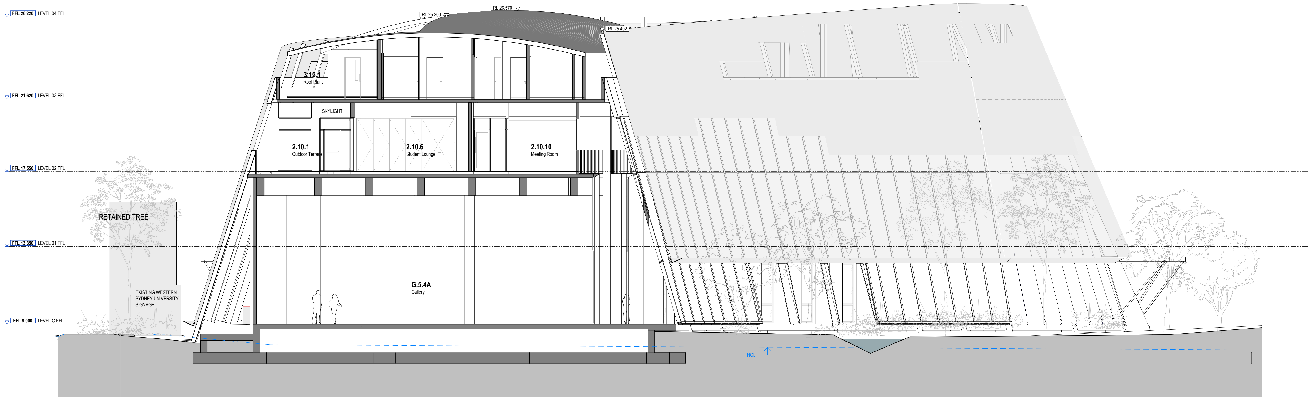
1 DA SECTION 5 1 : 100
