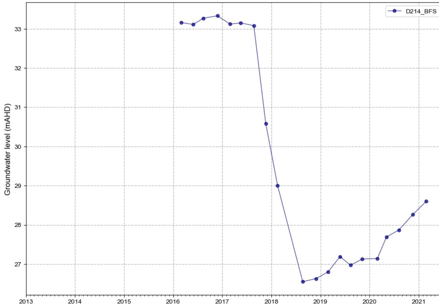
Figure A 26 D214_BFS
