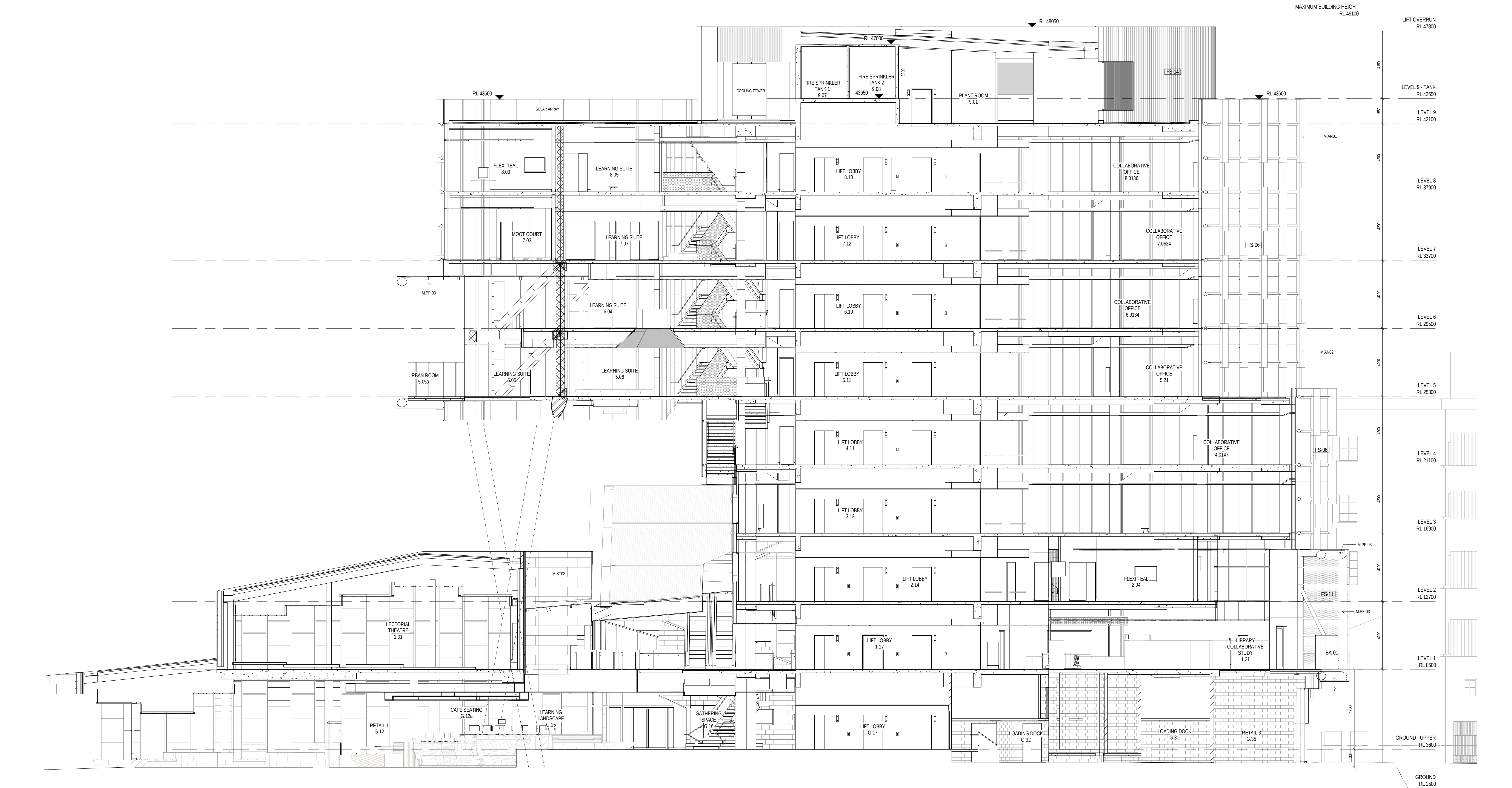
A SECTION AA Scale 1 : 100
