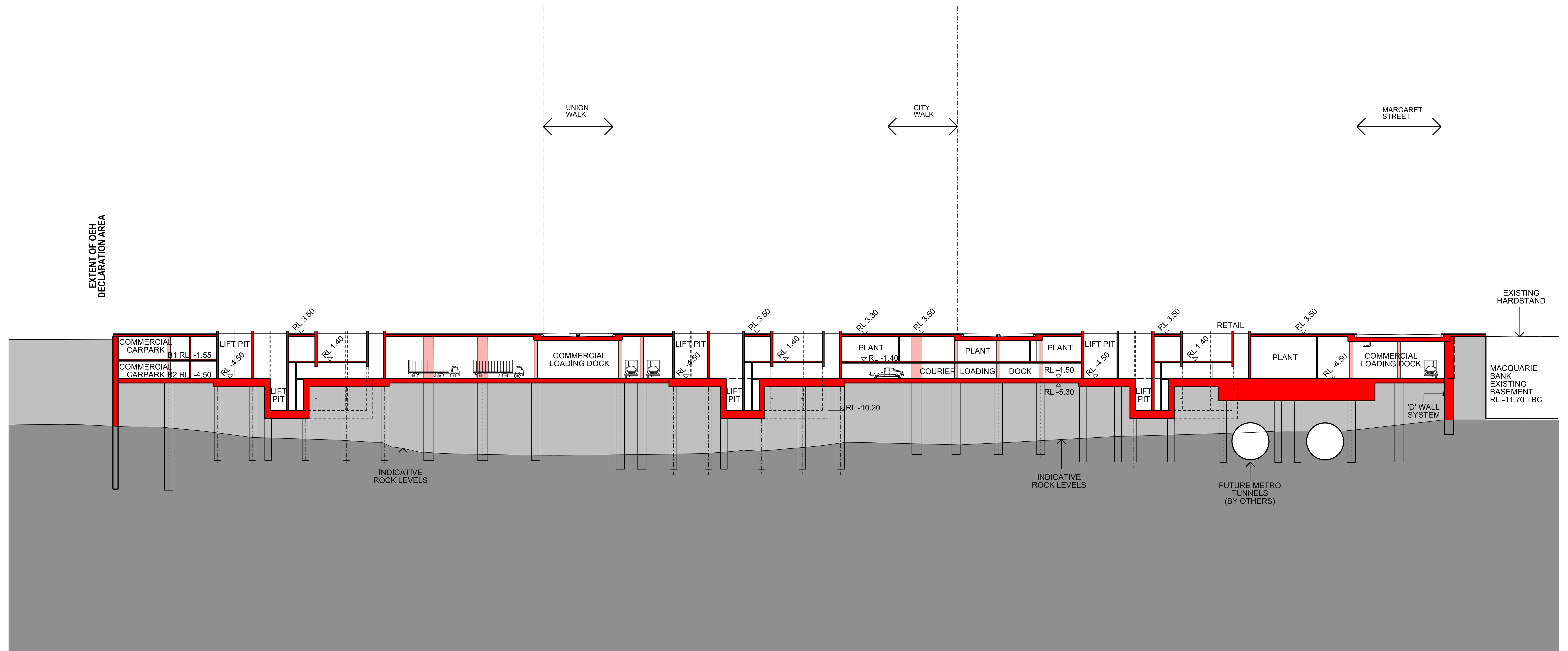
LONGITUDINAL SECTION 2-2
