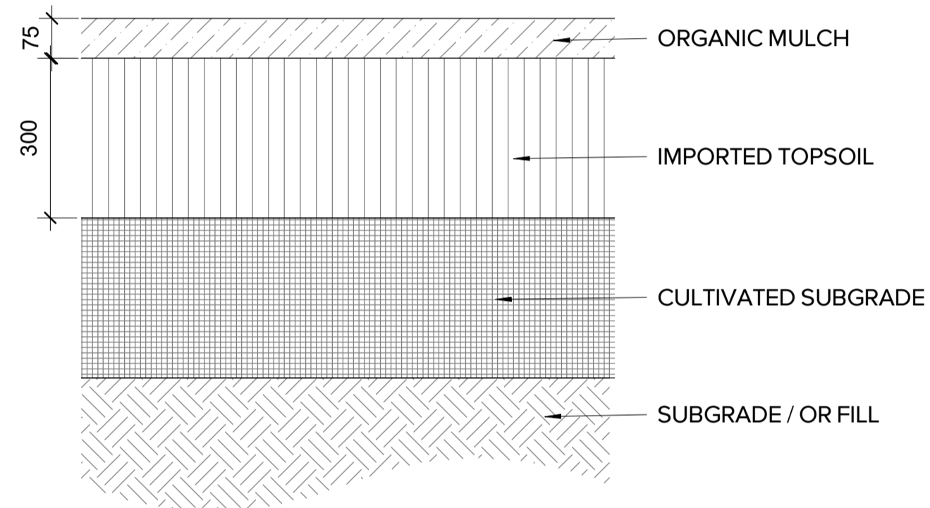
2 PLANTIG - ON GRADE 1 : 10
