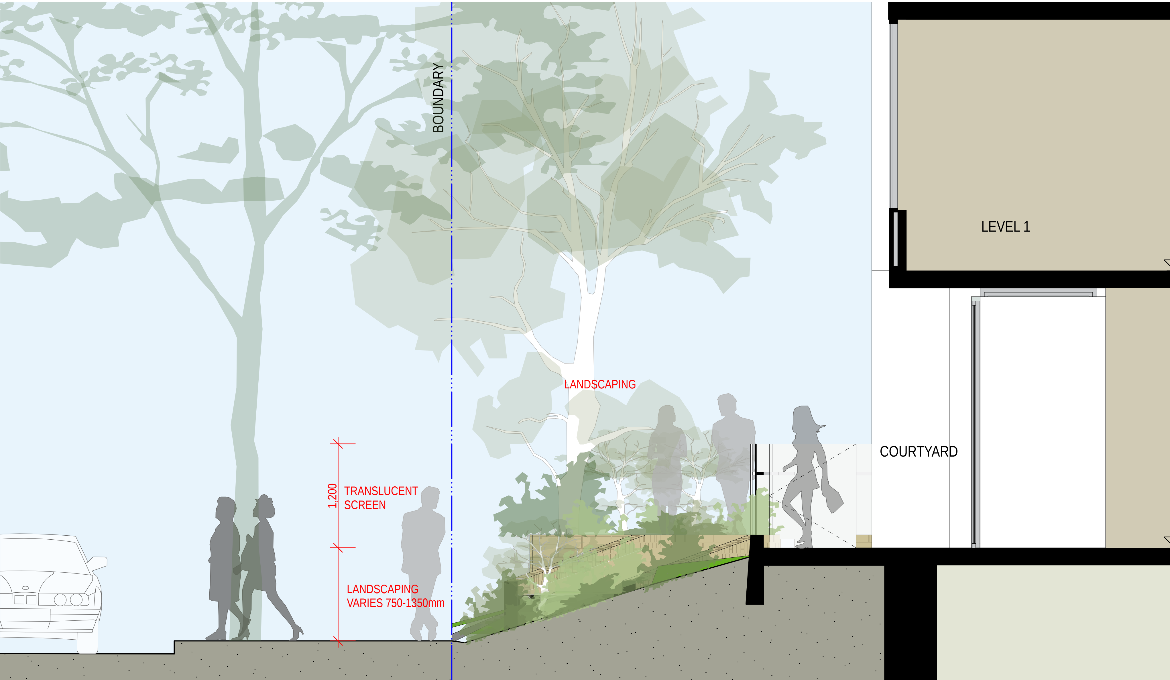
2 Section D_ 1:25
