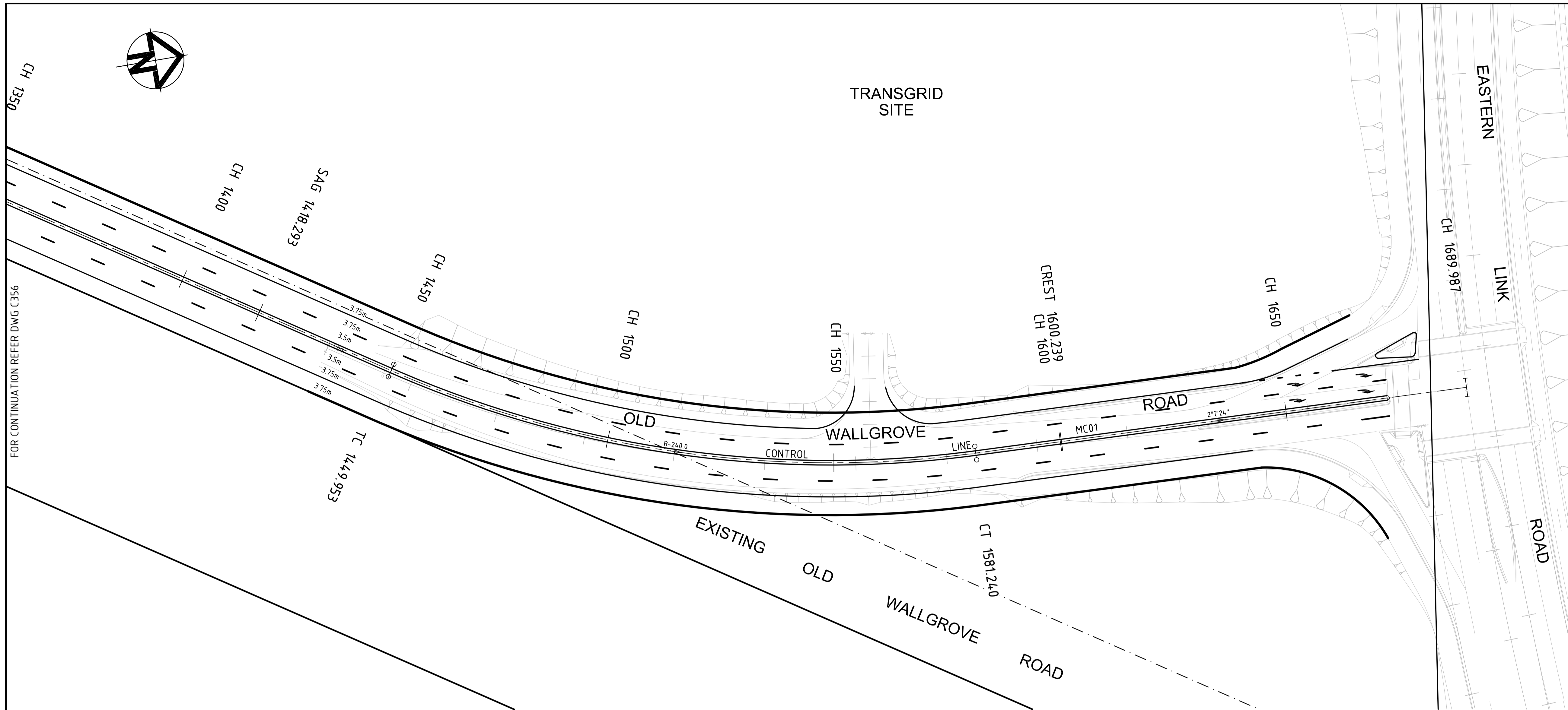
PLAN SCALE 1 : 500
