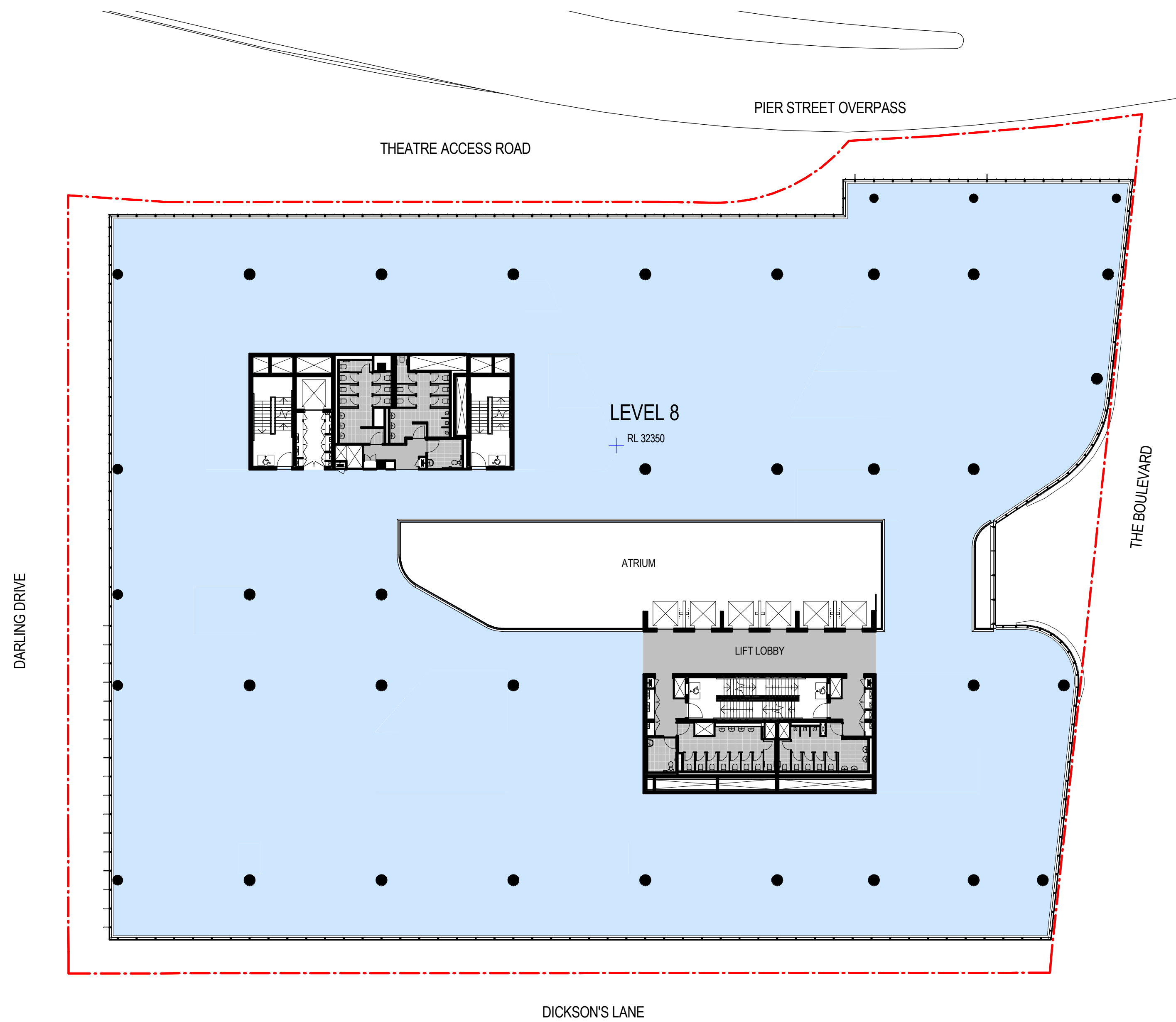
2 Level 8 - Section 96 SCALE 1 : 250
