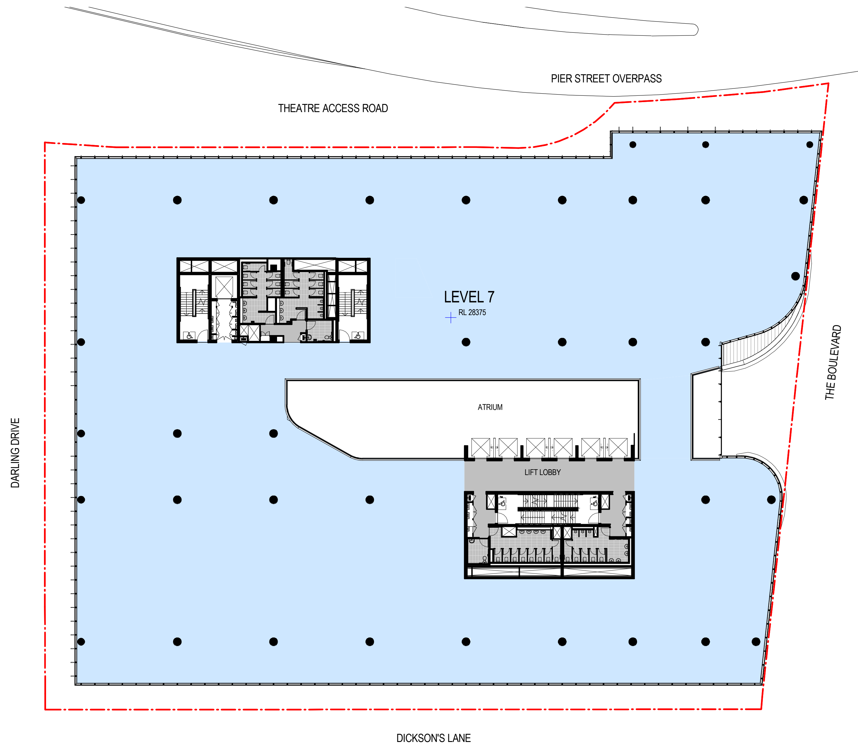
2 Level 7 - Section 96 SCALE 1 : 250
