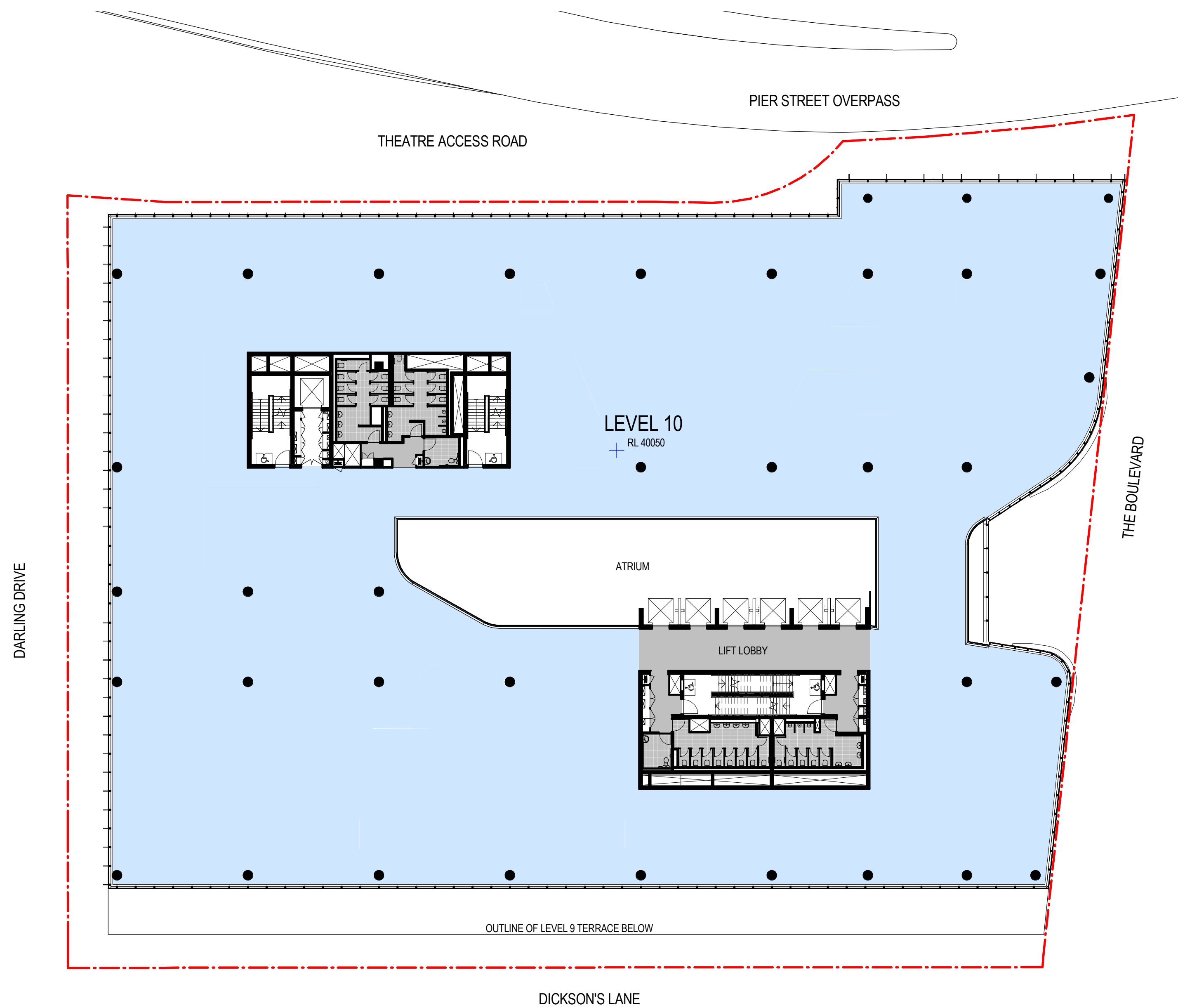
2 Level 10 - Section 96 SCALE 1 : 250
