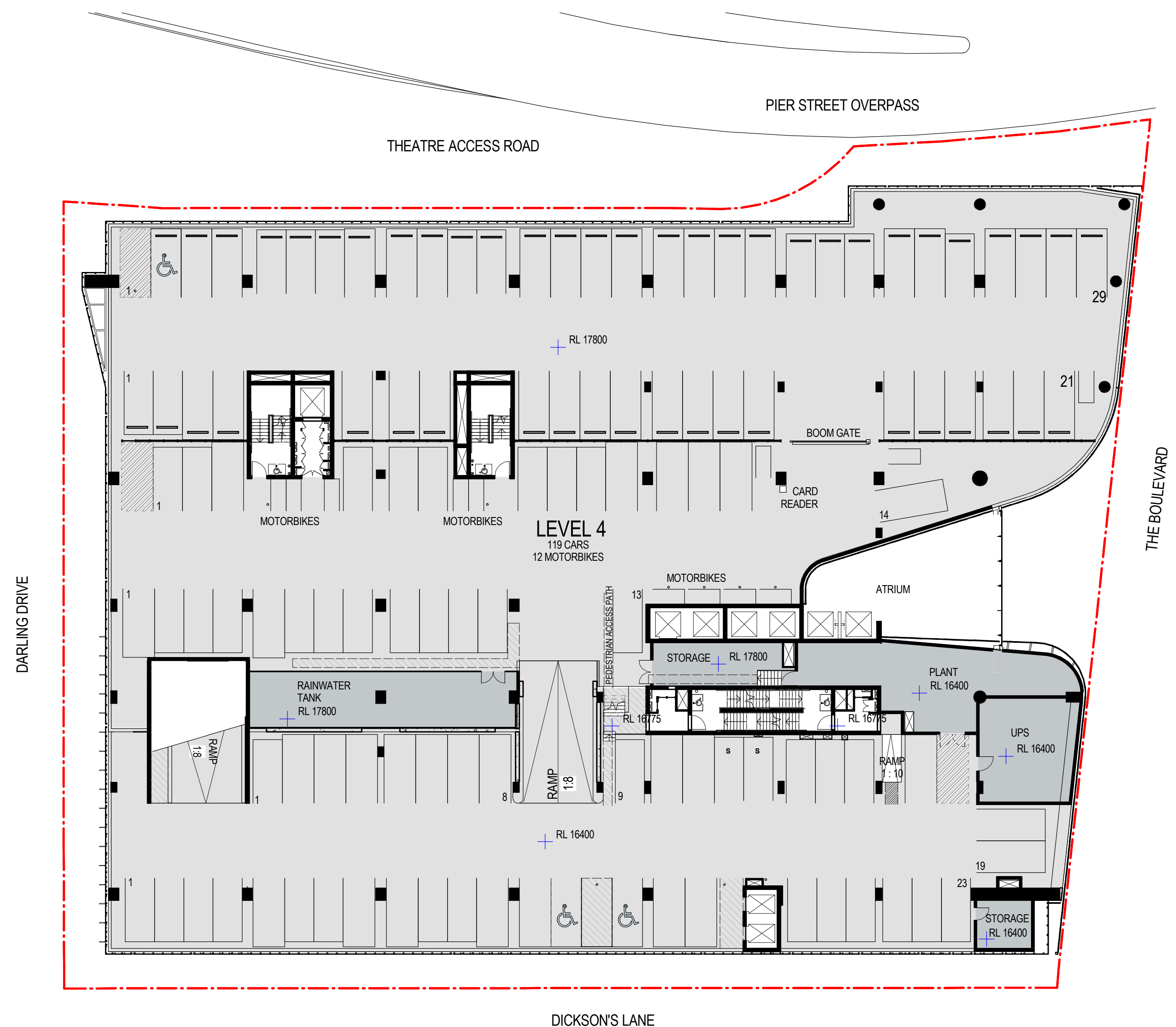
2 Level 4 - Section 96 SCALE 1 : 250
