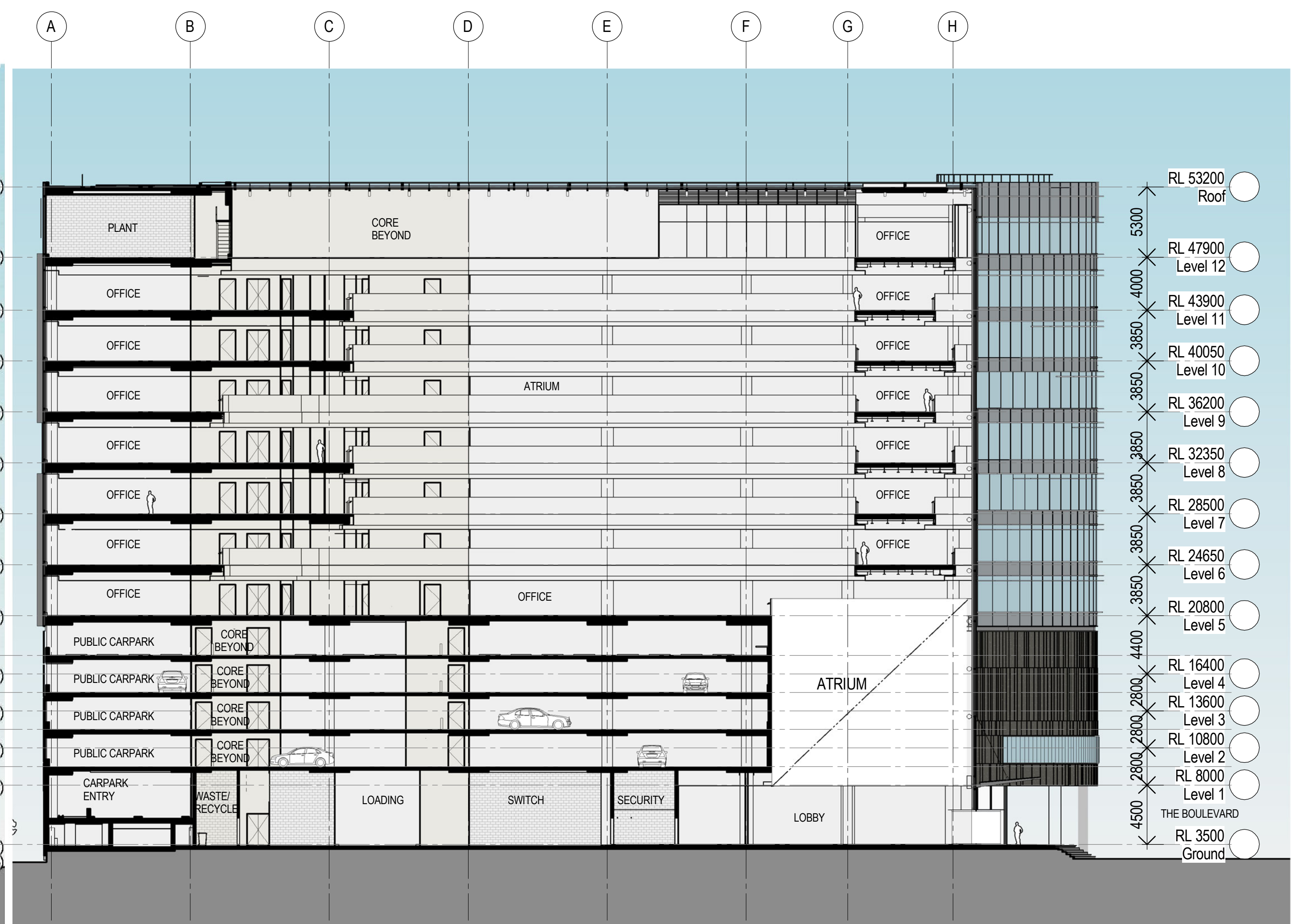
1 Section AA - Section 96 SCALE 1 : 250
