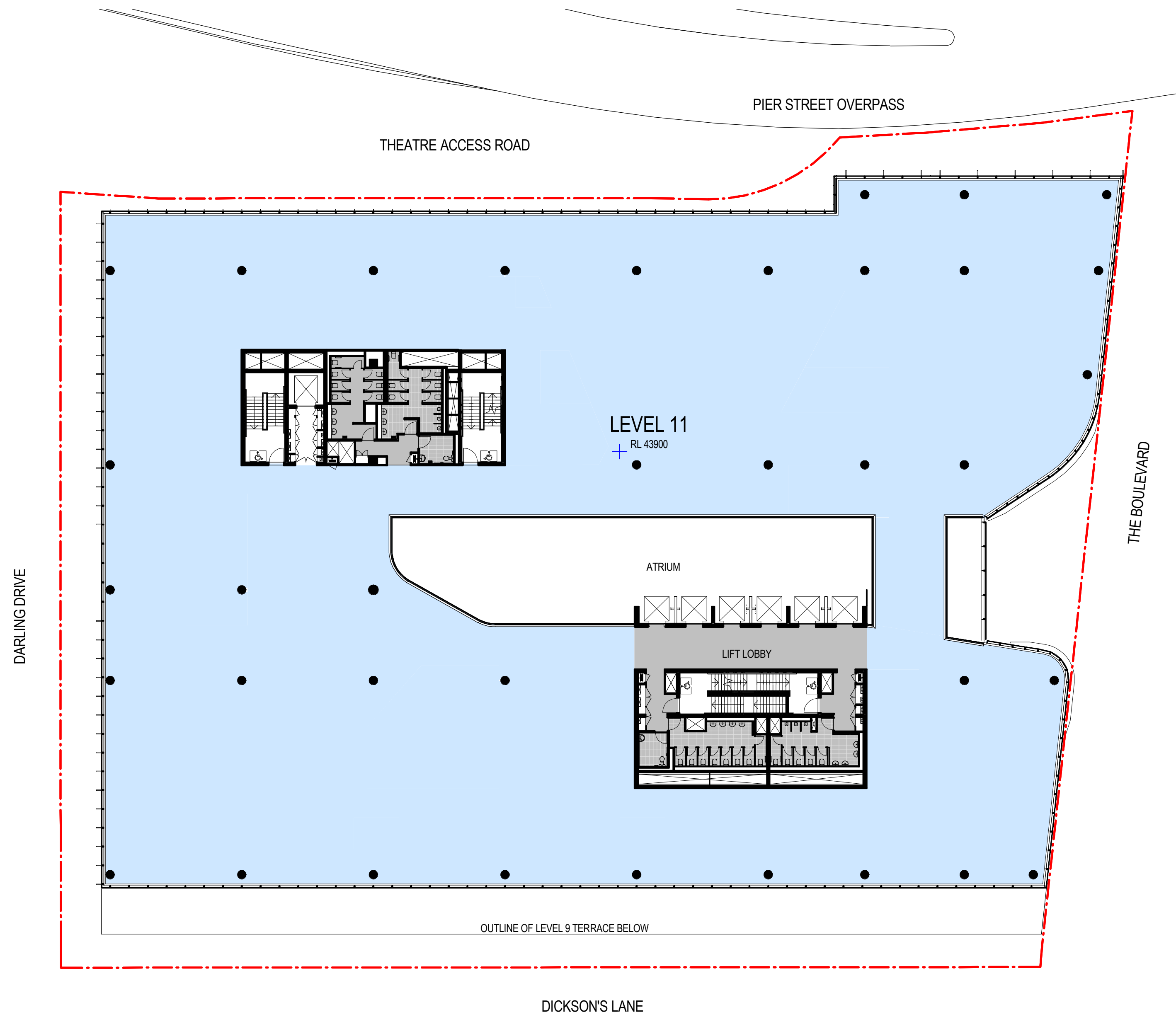
2 Level 11 - Section 96 SCALE 1 : 250
