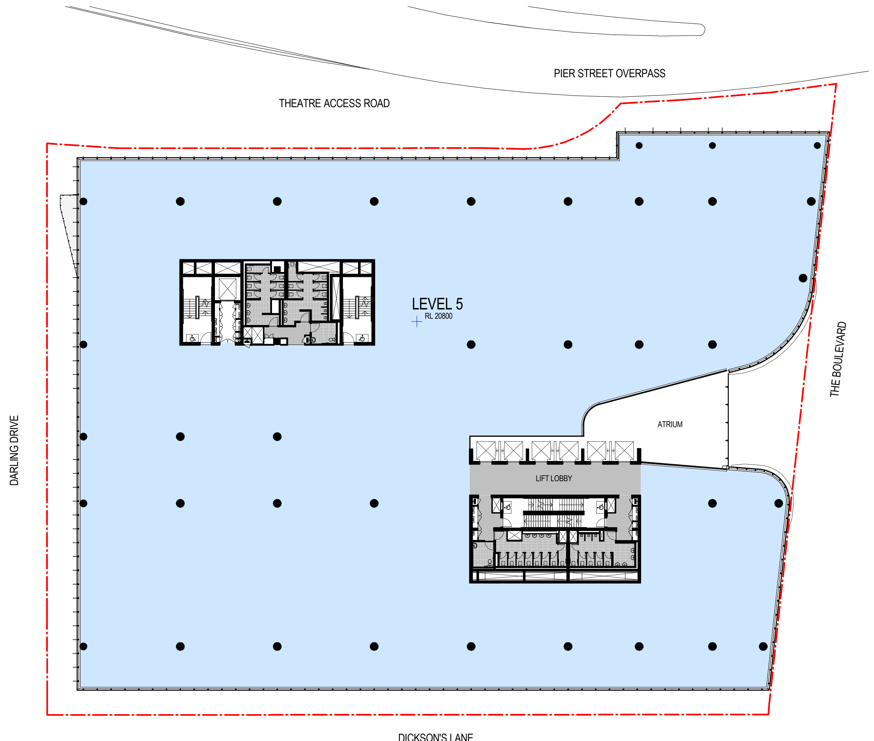
2 Level 5 - Section 96 SCALE 1 : 250
