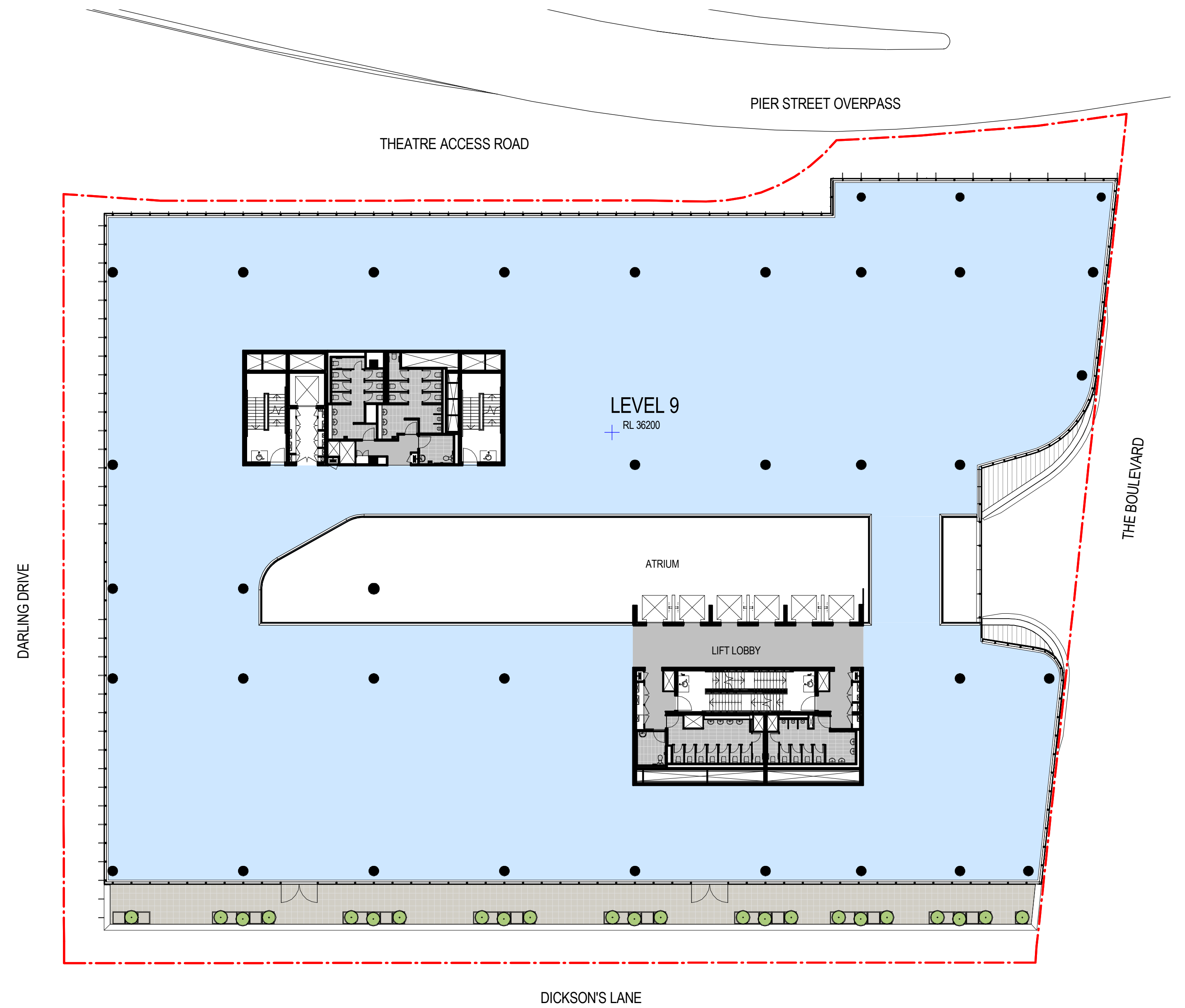
2 Level 9 - Section 96 SCALE 1 : 250
