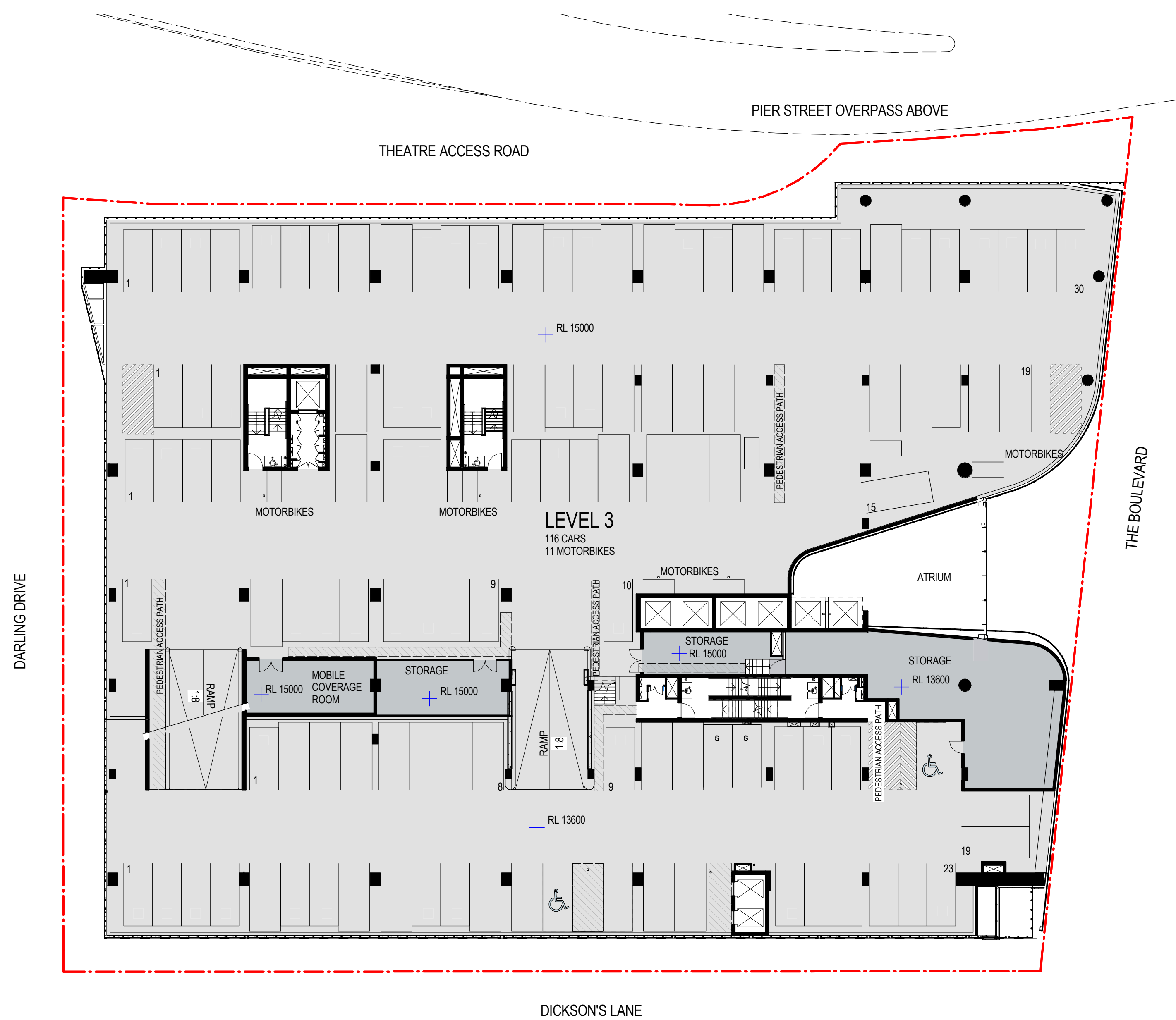
2 Level 3 - Section 96 SCALE 1 : 250
