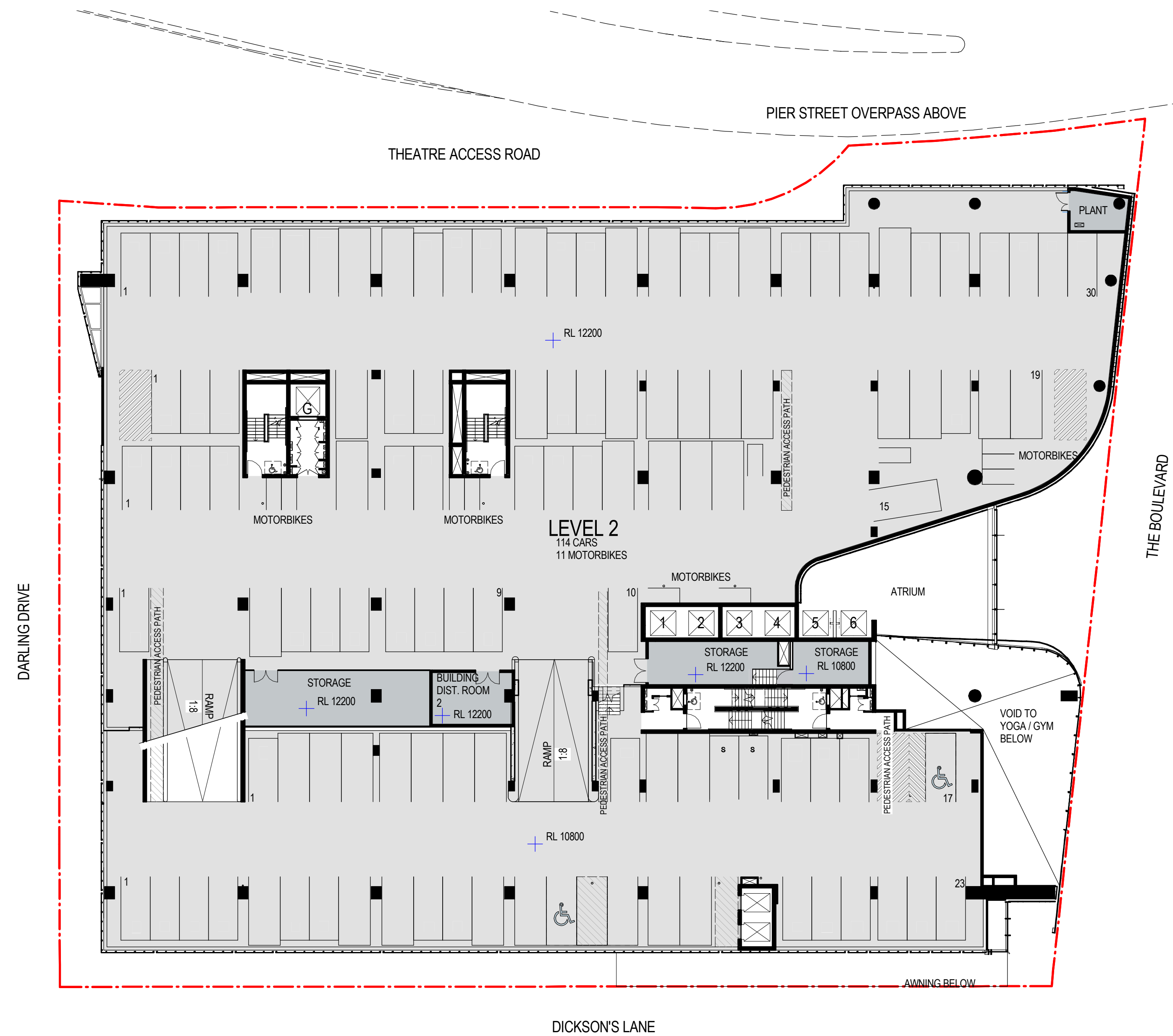
1 Level 2 - Section 96 SCALE 1 : 250
