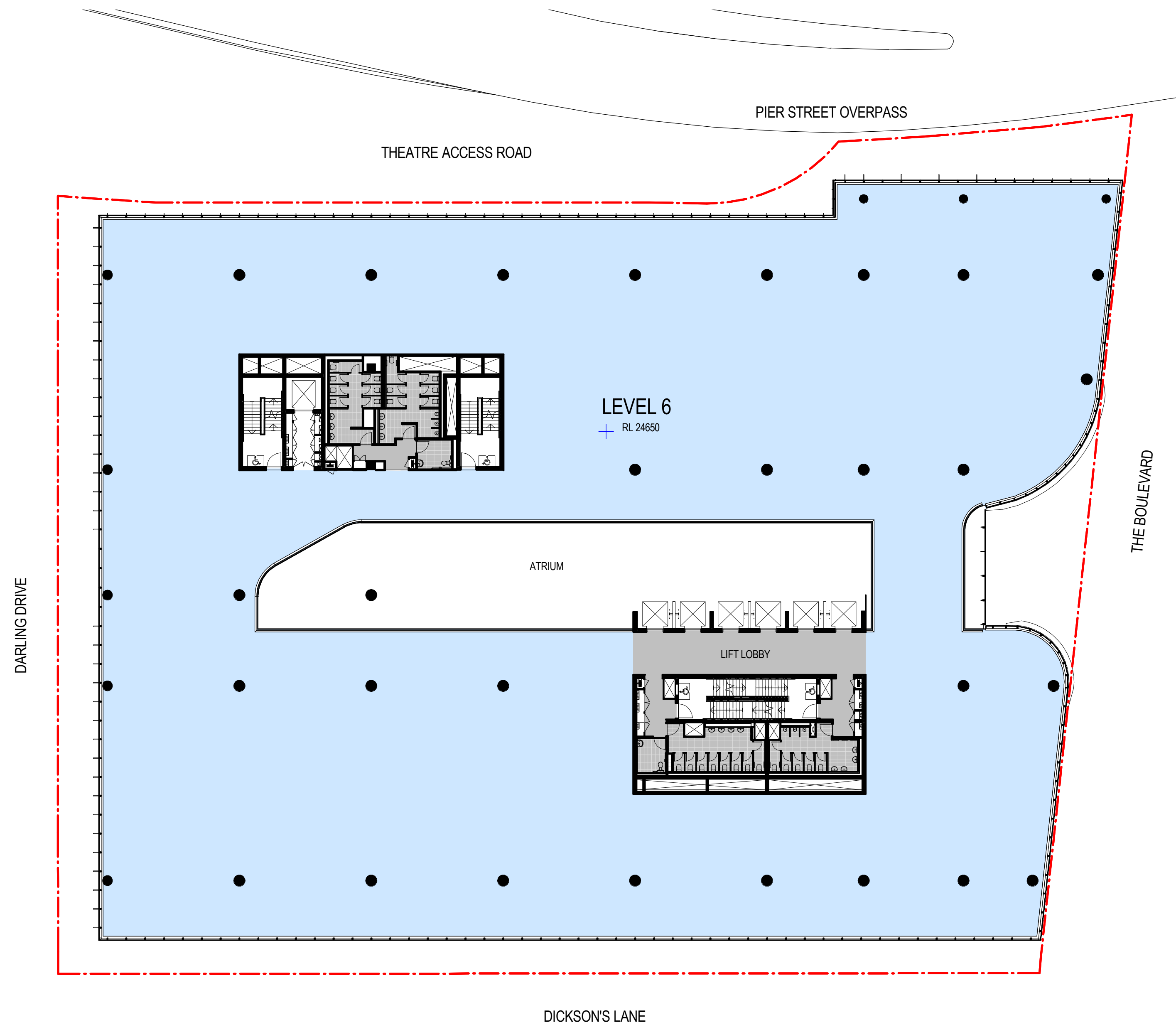
2 Level 6 - Section 96 SCALE 1 : 250
