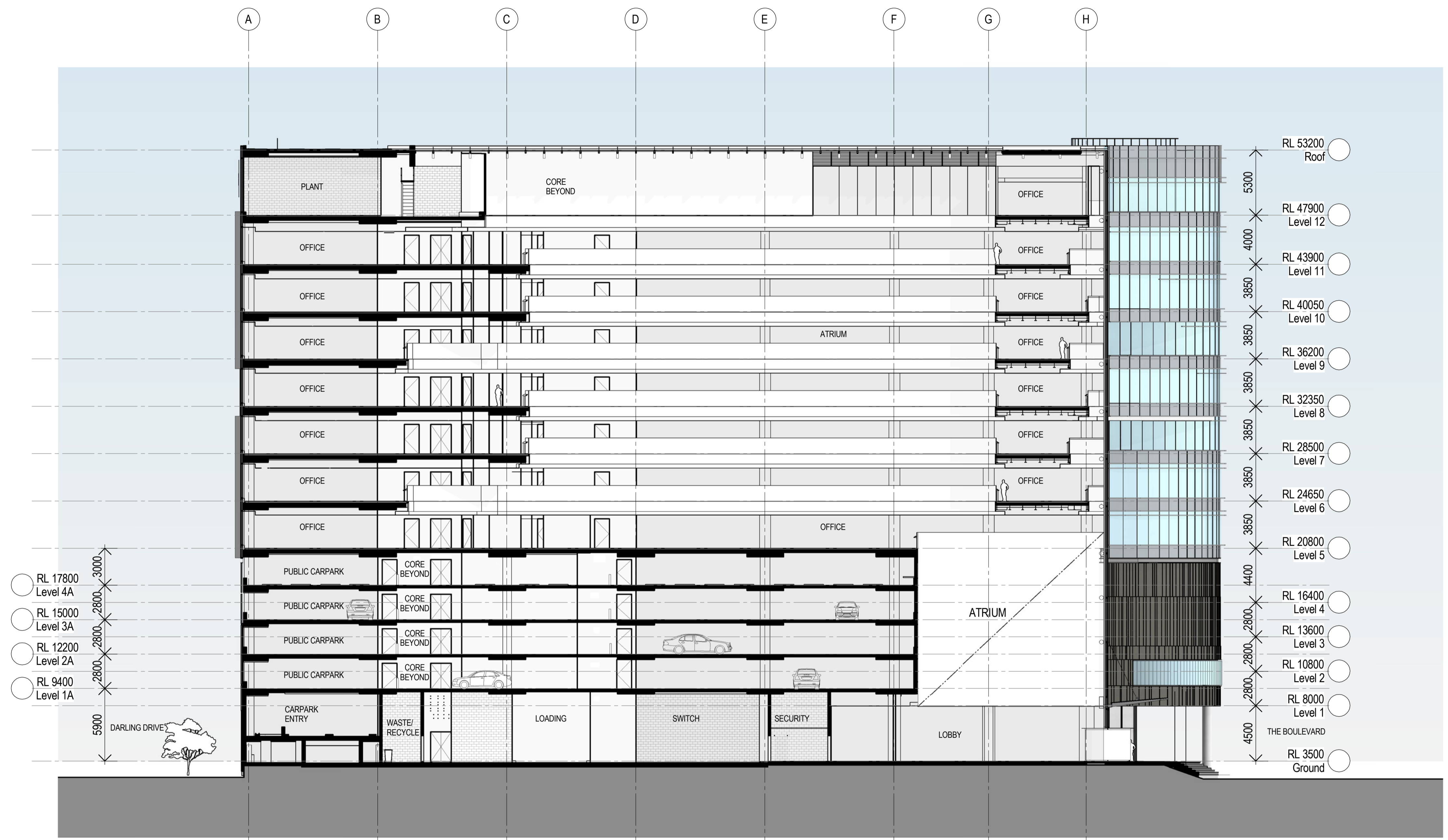
1 SECTION AA SCALE 1 : 200
