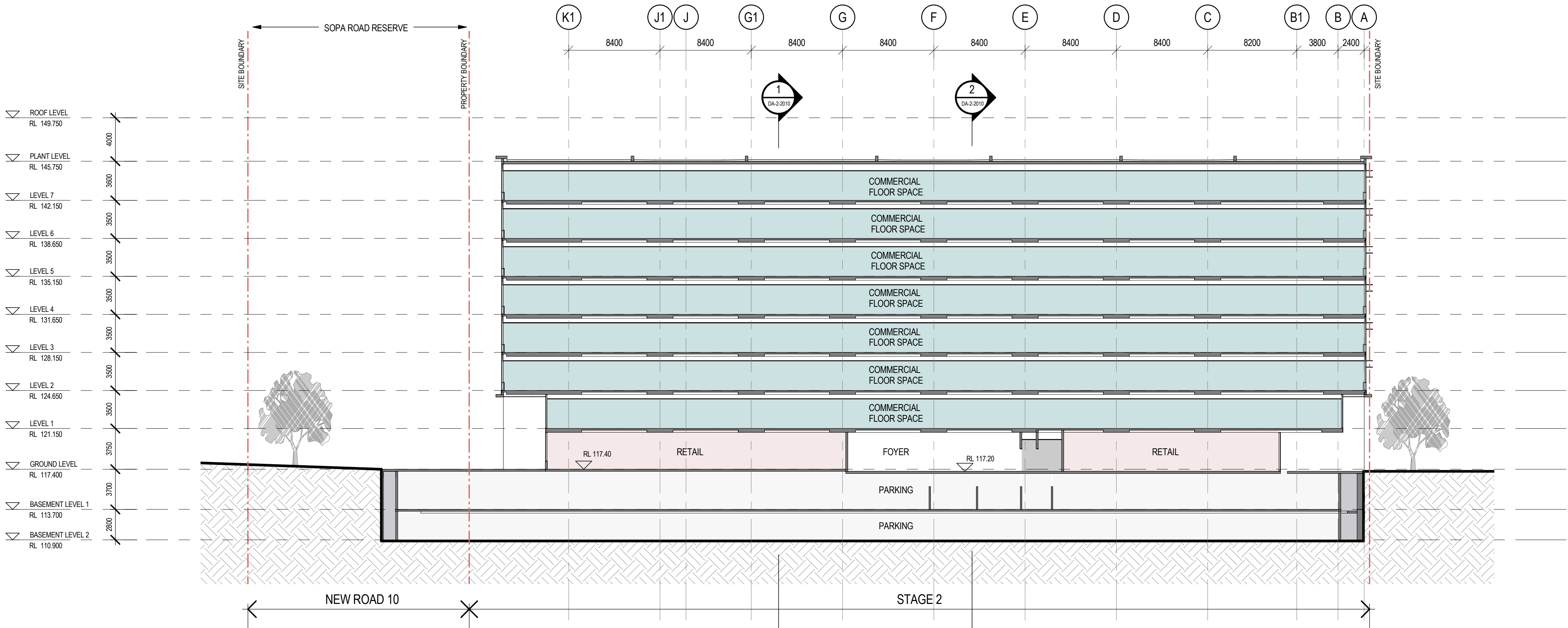
4 Section 4 1 : 250
