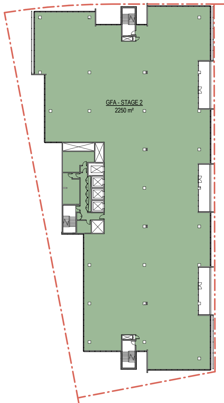
9 Level 6 1 : 500
