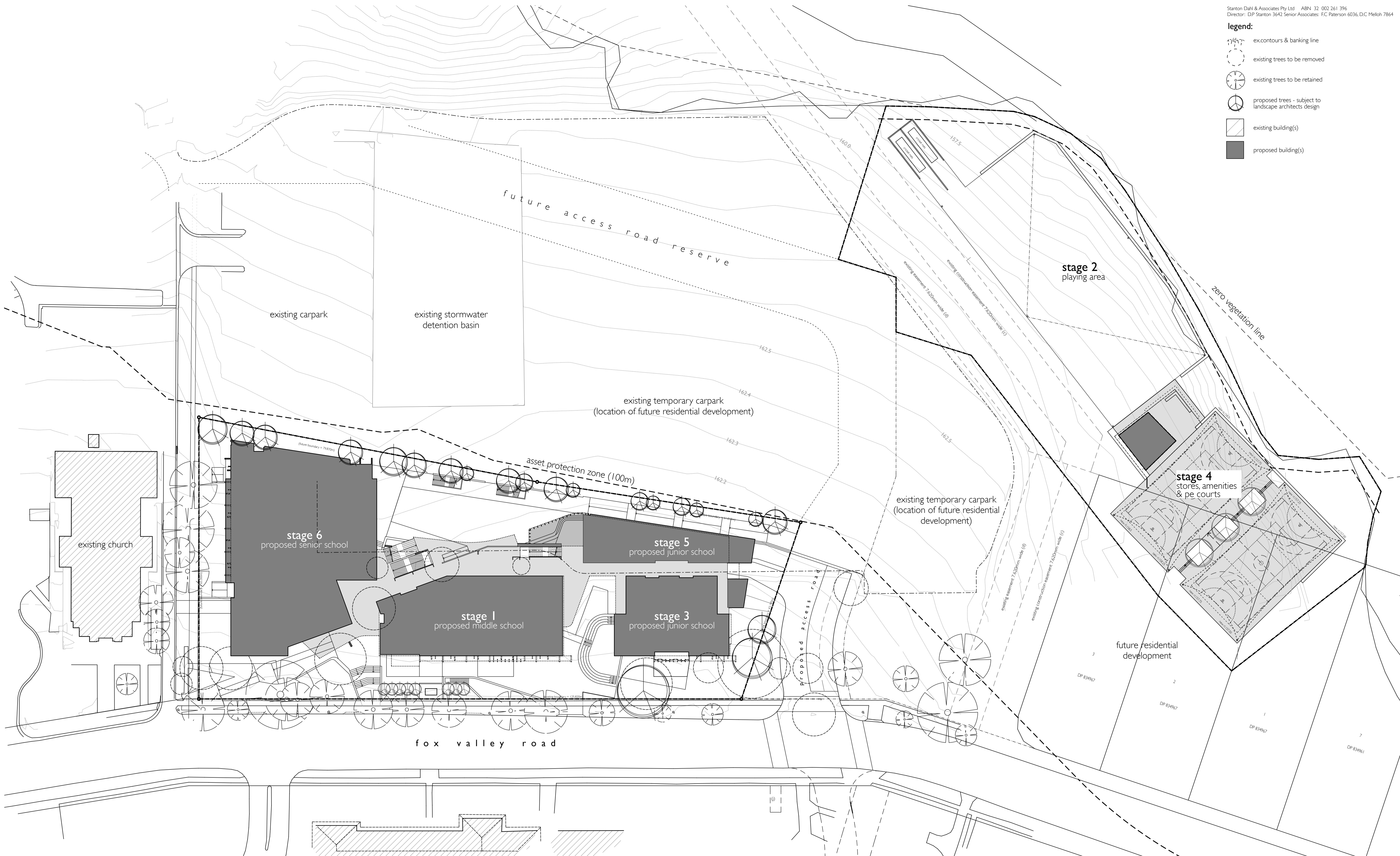
01 precinct plan 1:400
