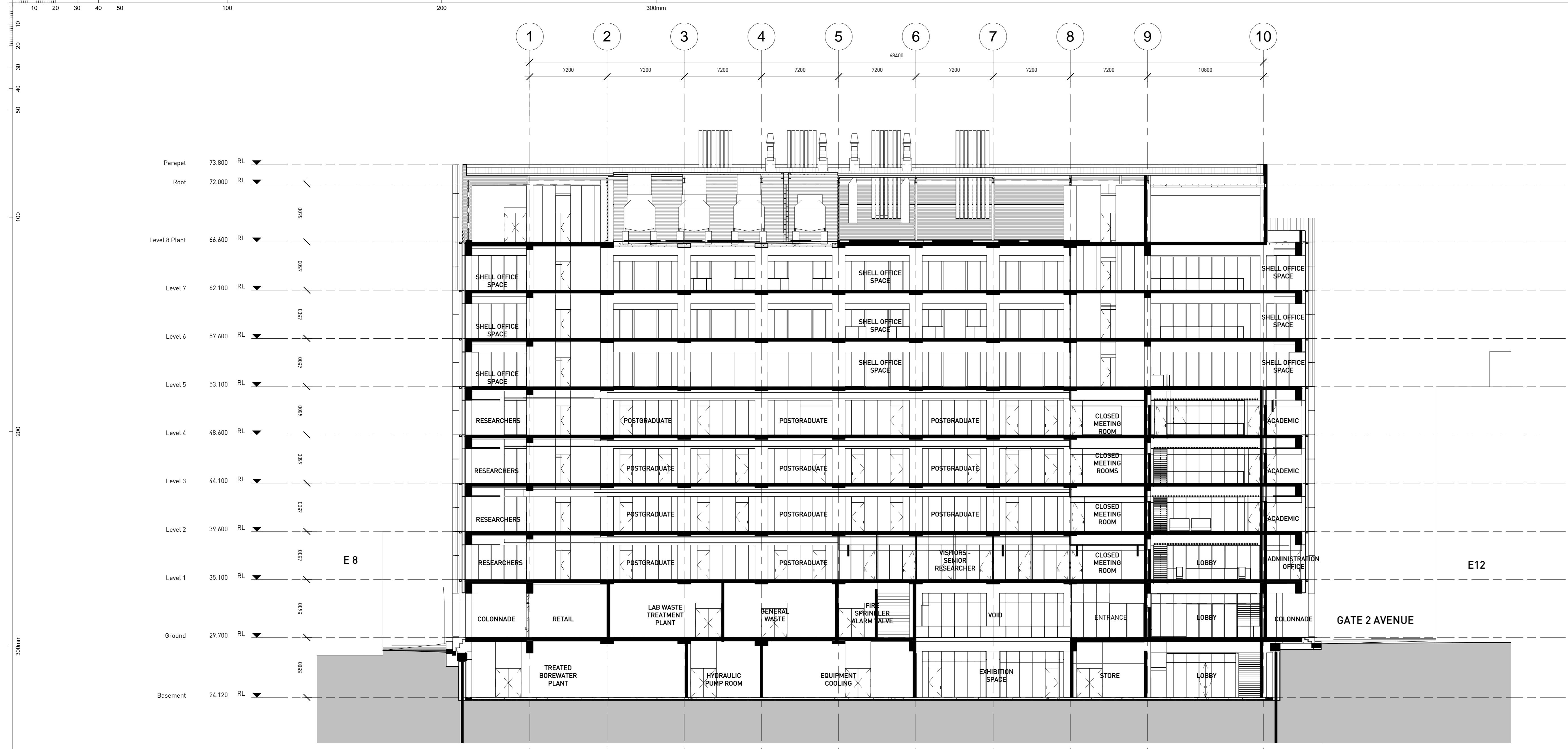
SECTION 4 SCALE: 1:200
