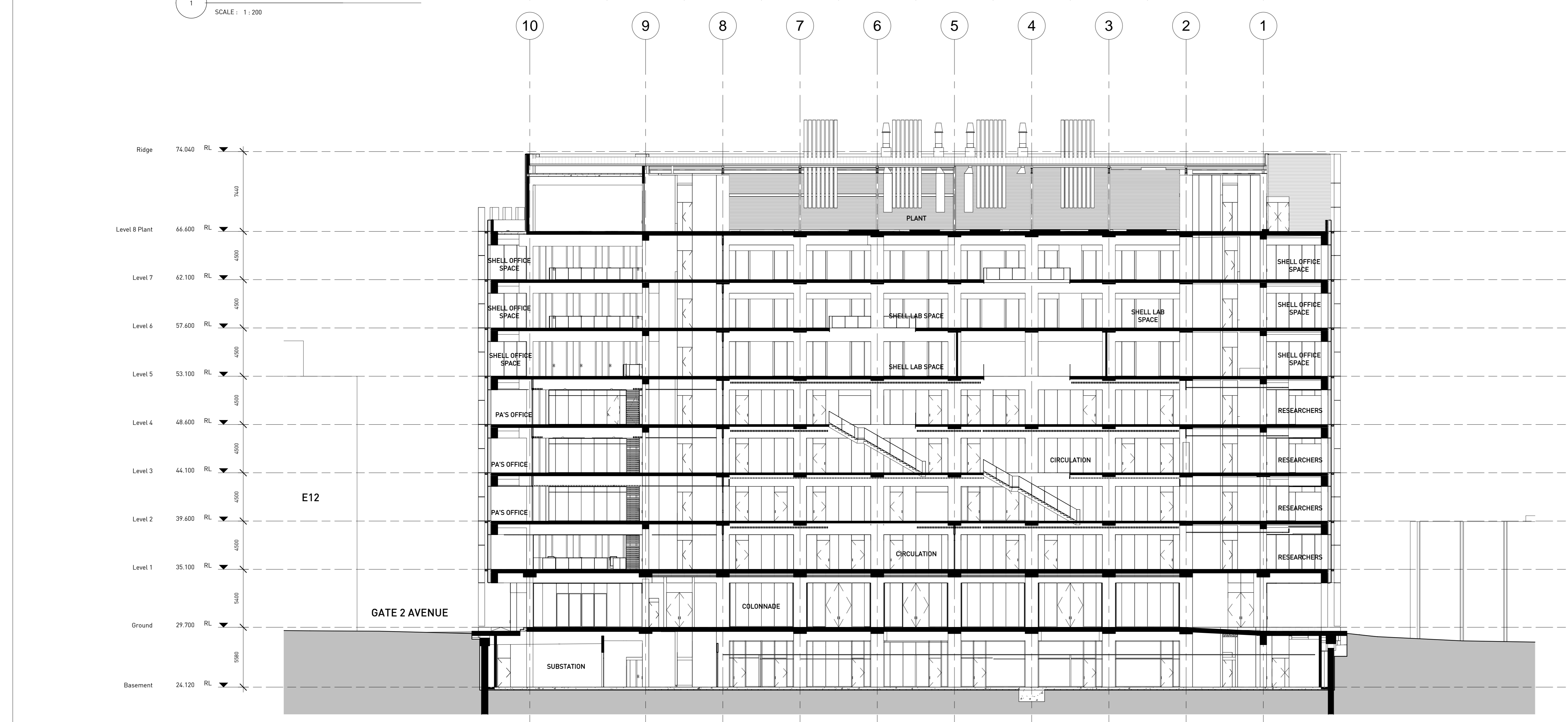
SECTION 5 SCALE: 1:200
