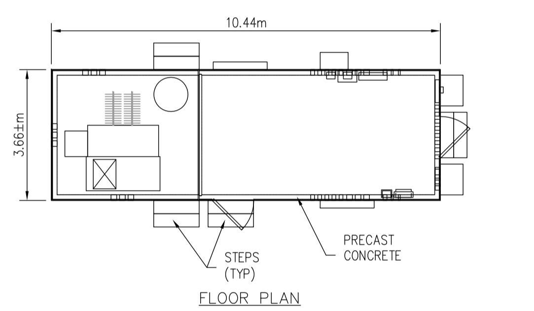
1 PRELIMINARY STAGING LAYOUT Scale: NONE
