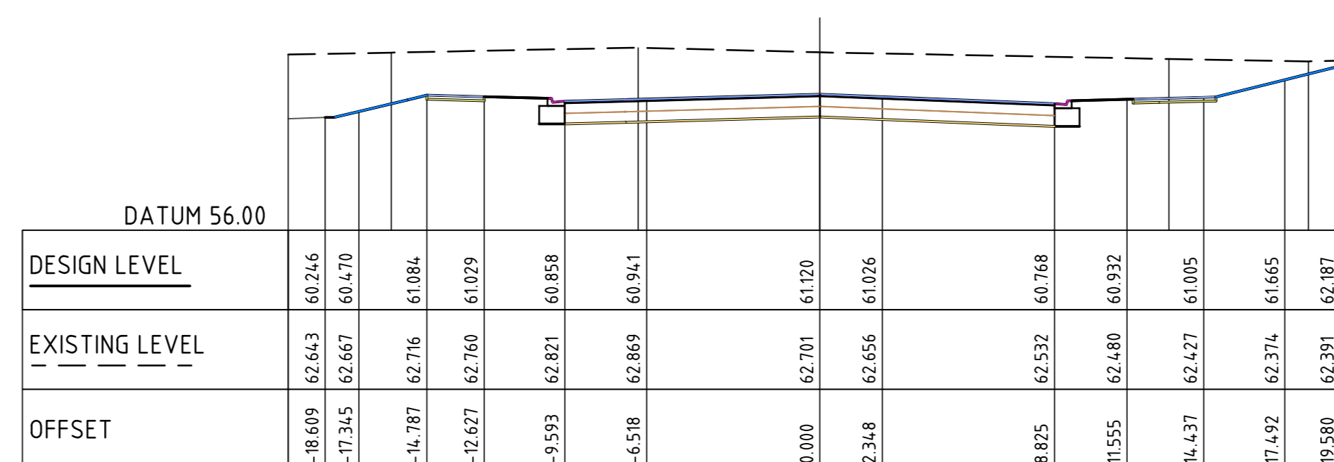
CL DIST RD 1 CH 520.000
