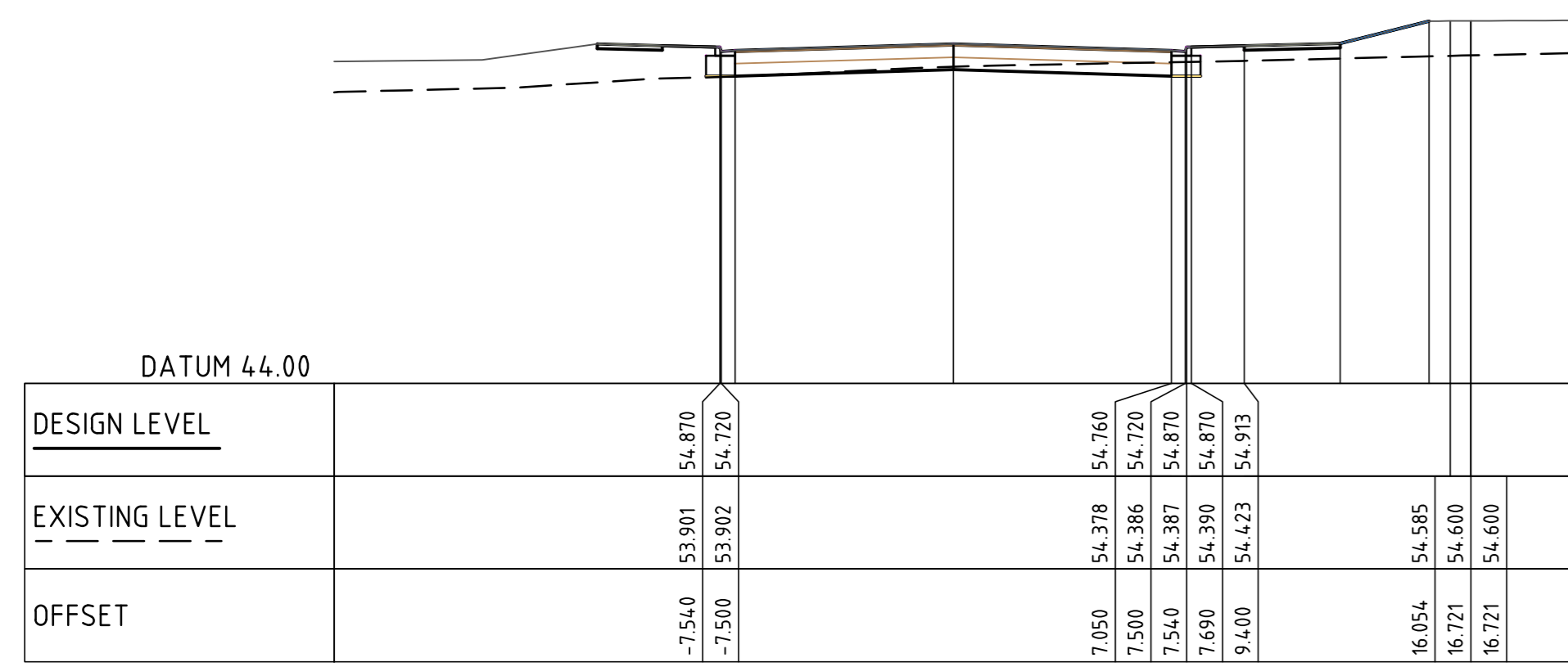
CL IND RD 1 CH 80.000 SCALE 1:200
