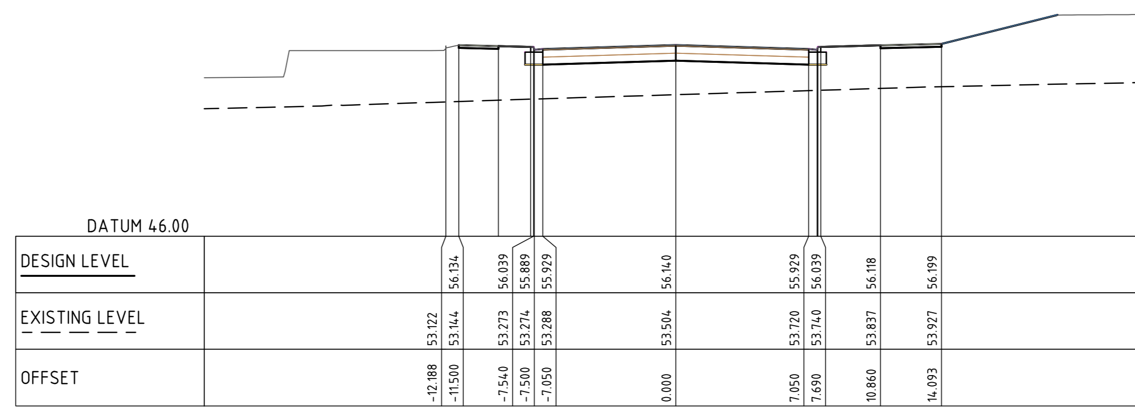
CL IND RD 1 CH 180.000 SCALE 1:200
