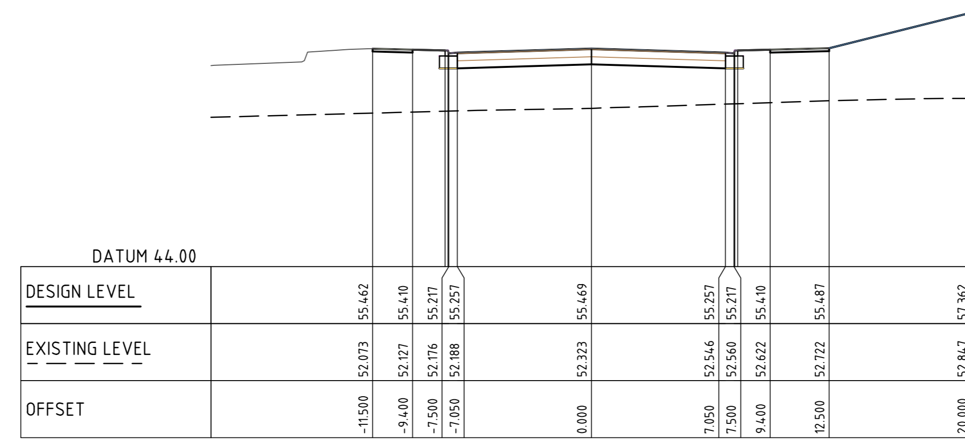
CL IND RD 1 CH 140.000 SCALE 1:200
