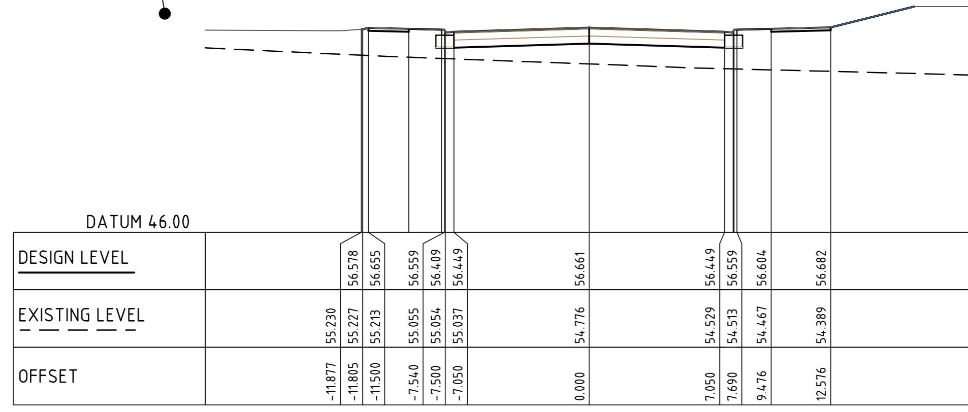
CL IND RD 1 CH 220.000 SCALE 1:200
