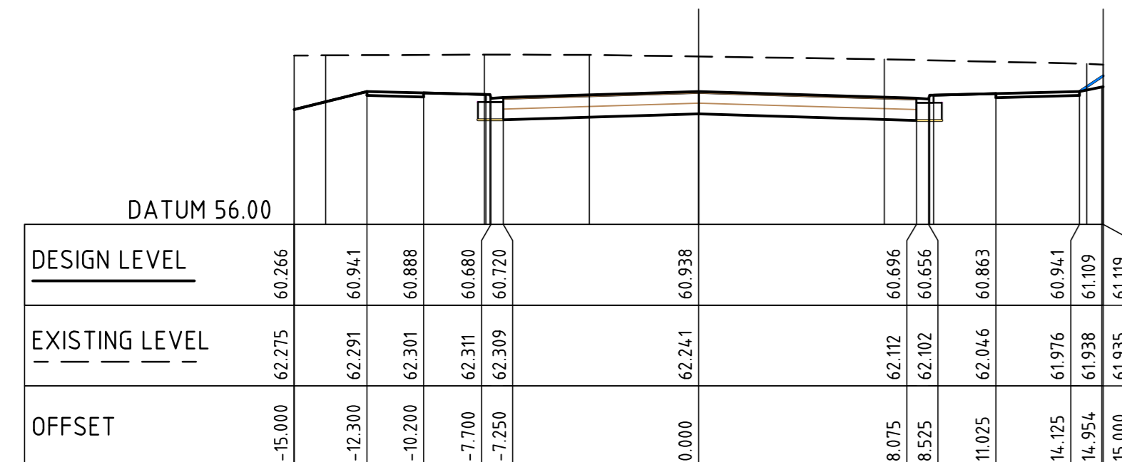
CL DIST RD 1 CH 500.000
