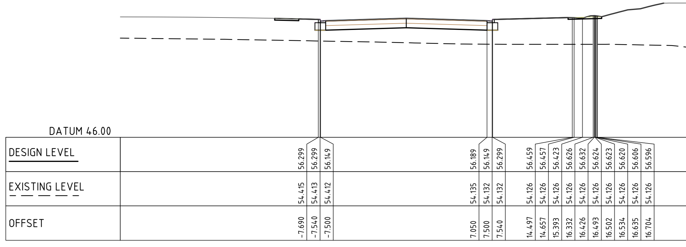
CL IND RD 1 CH 200.000 SCALE 1:200
