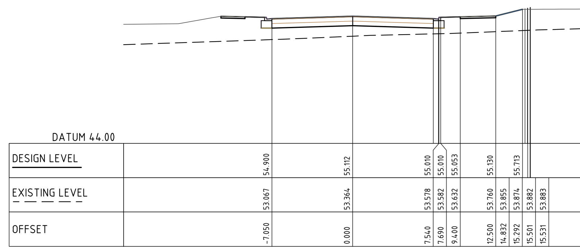
CL IND RD 1 CH 100.000 SCALE 1:200
