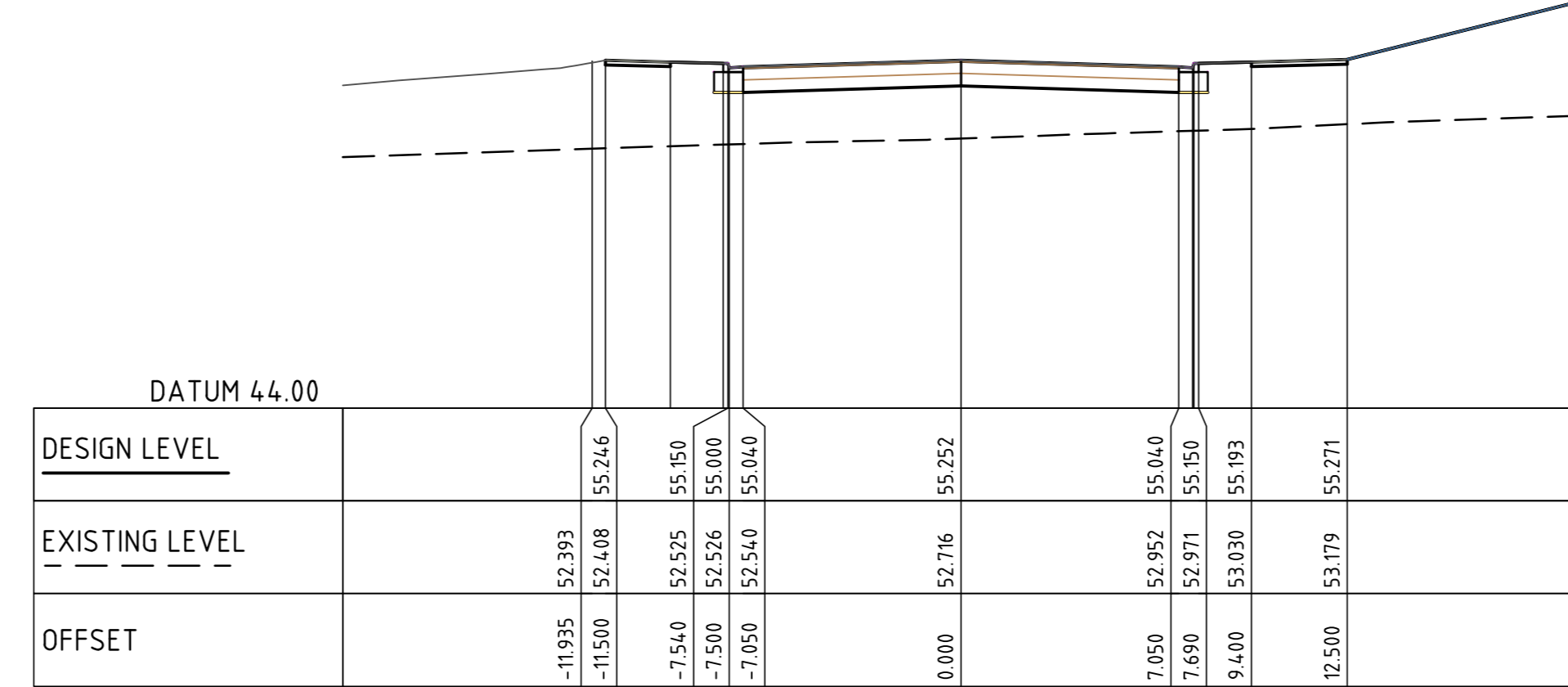
CL IND RD 1 CH 120.000 SCALE 1:200
