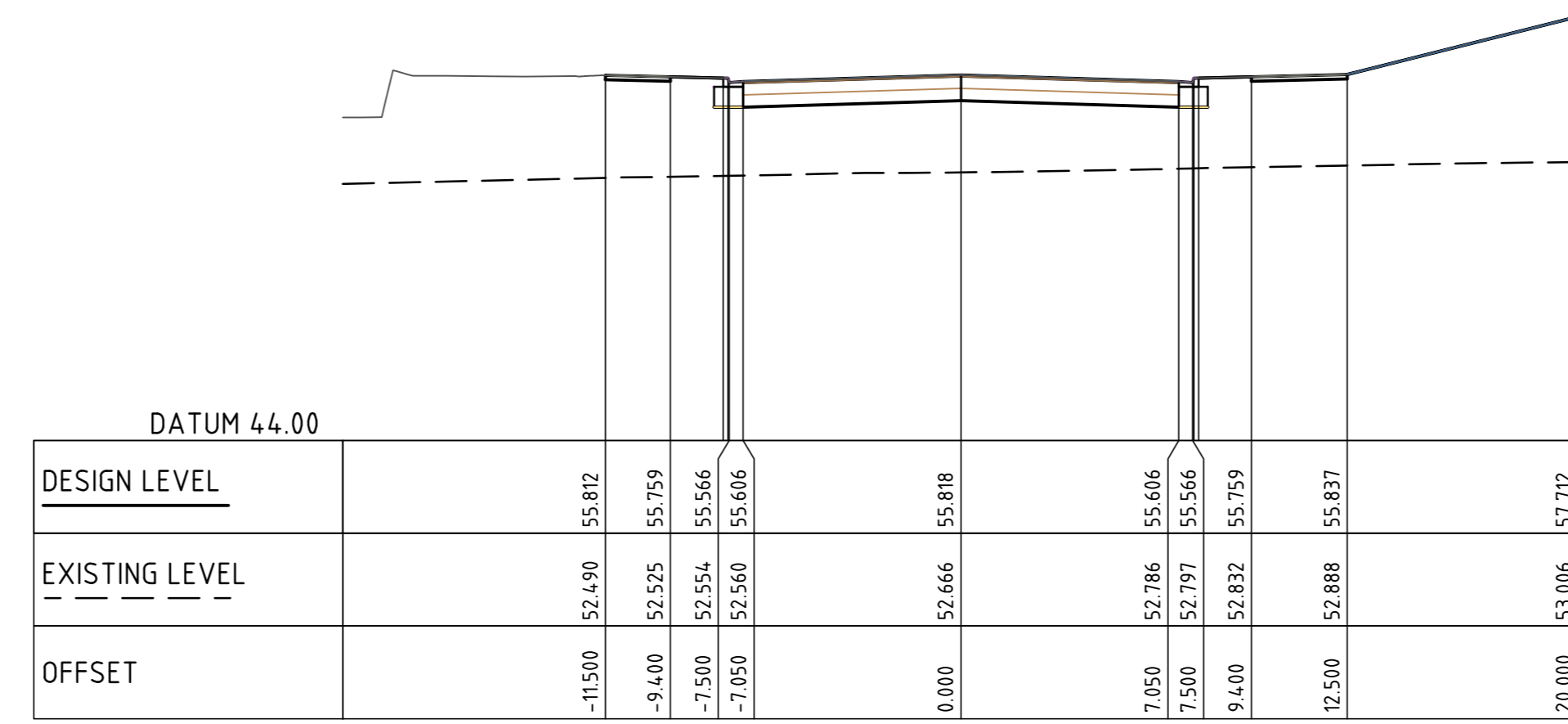
CL IND RD 1 CH 160.000 SCALE 1:200
