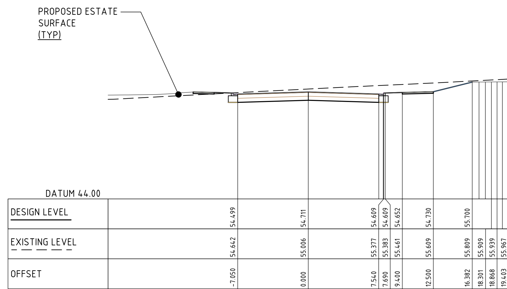
CL IND RD 1 CH 40.000 SCALE 1:200
