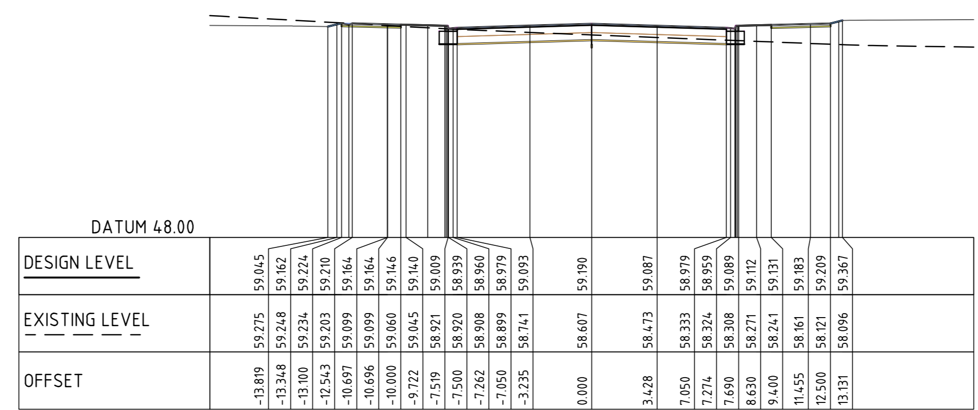
CL IND RD 1 CH 340.000 SCALE 1:200
