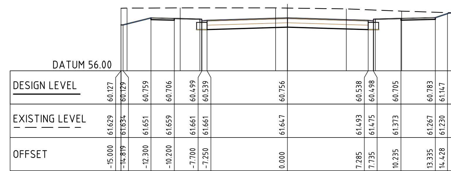
CL DIST RD 1 CH 480.000
