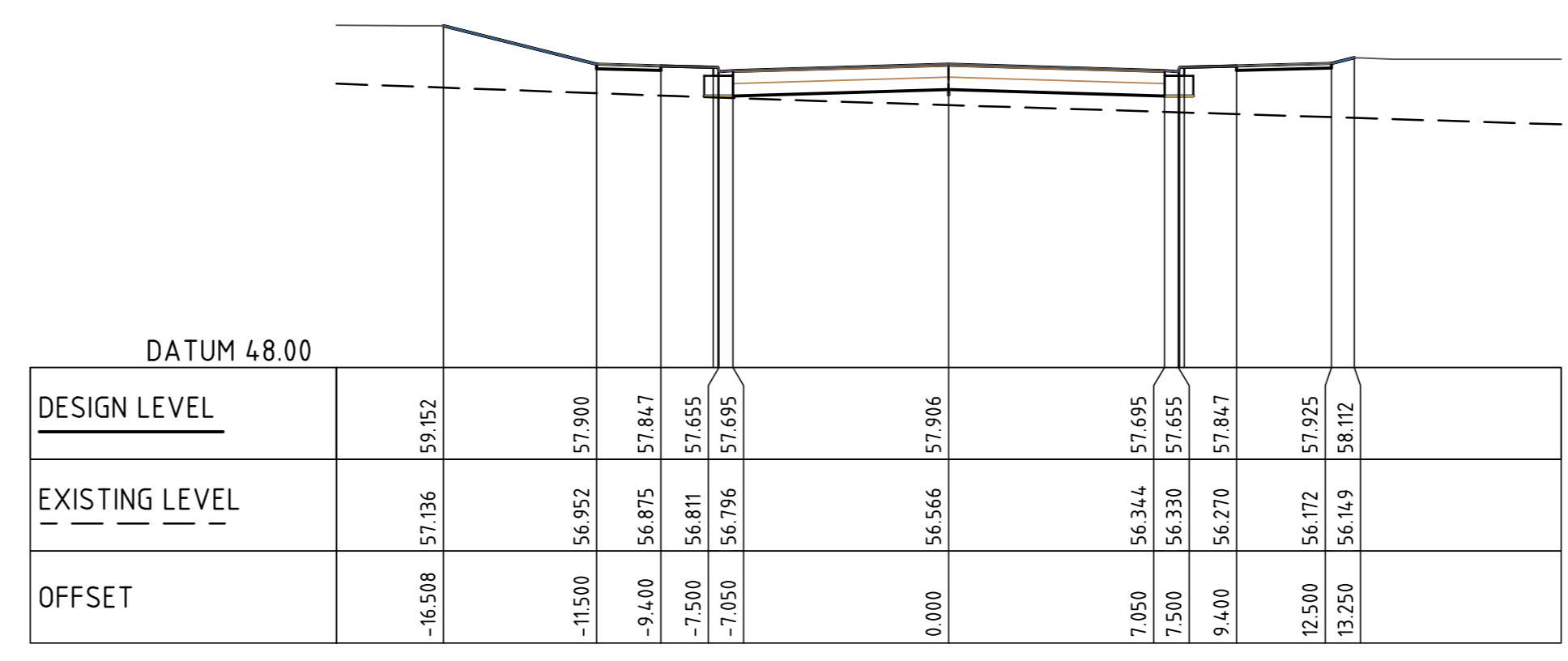
CL IND RD 1 CH 280.000 SCALE 1:200
