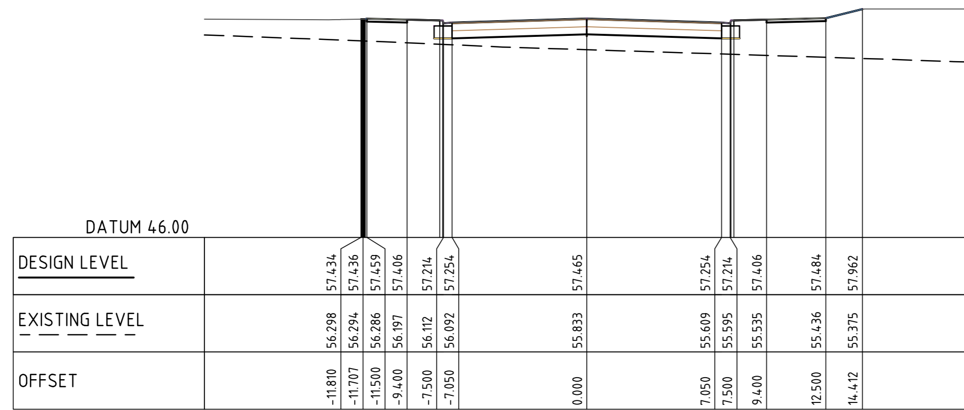
CL IND RD 1 CH 260.000 SCALE 1:200
