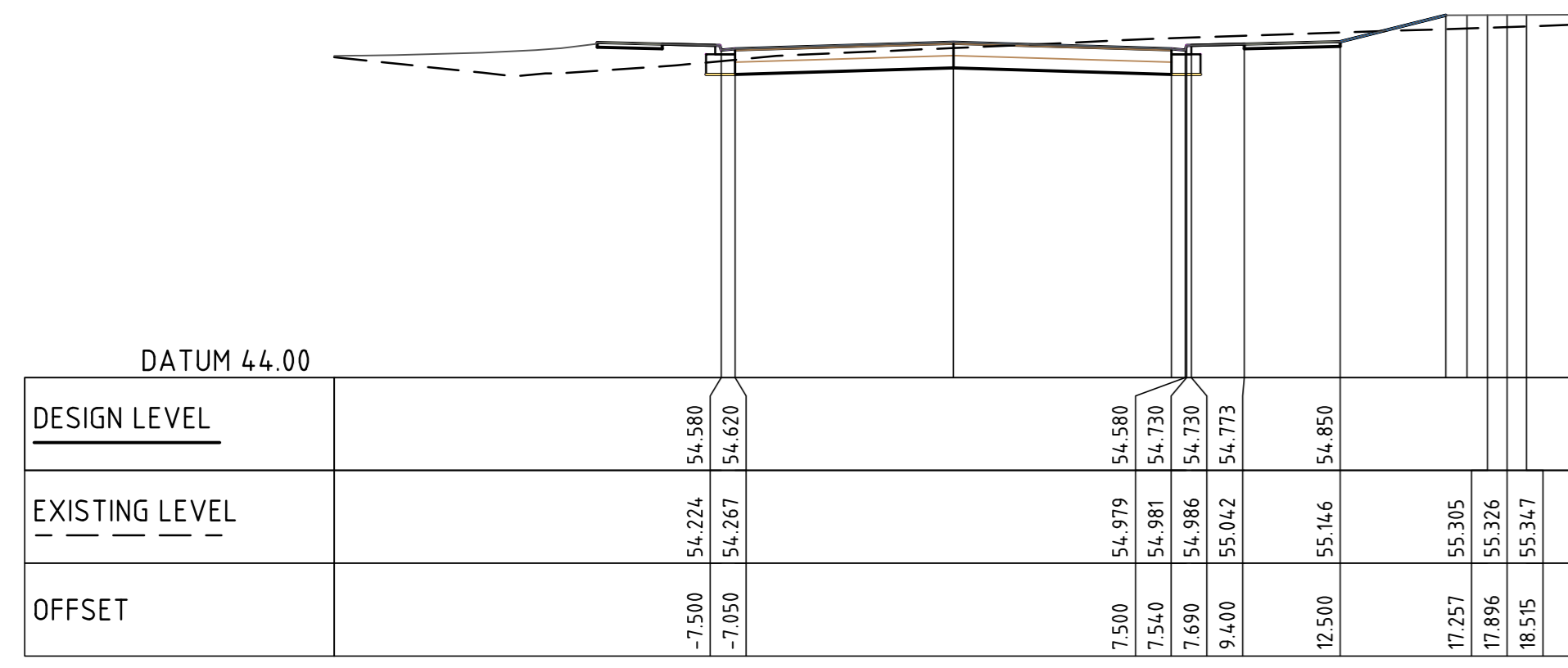
CL IND RD 1 CH 60.000 SCALE 1:200
