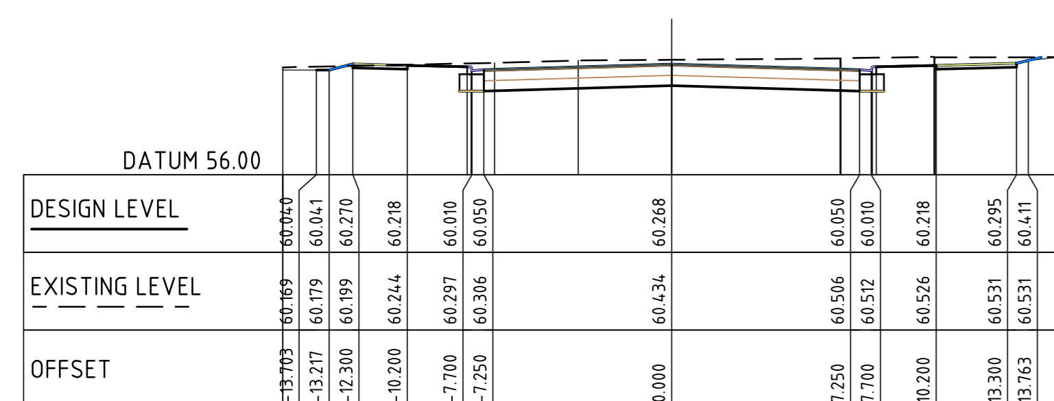
CL DIST RD 1 CH 420.000
