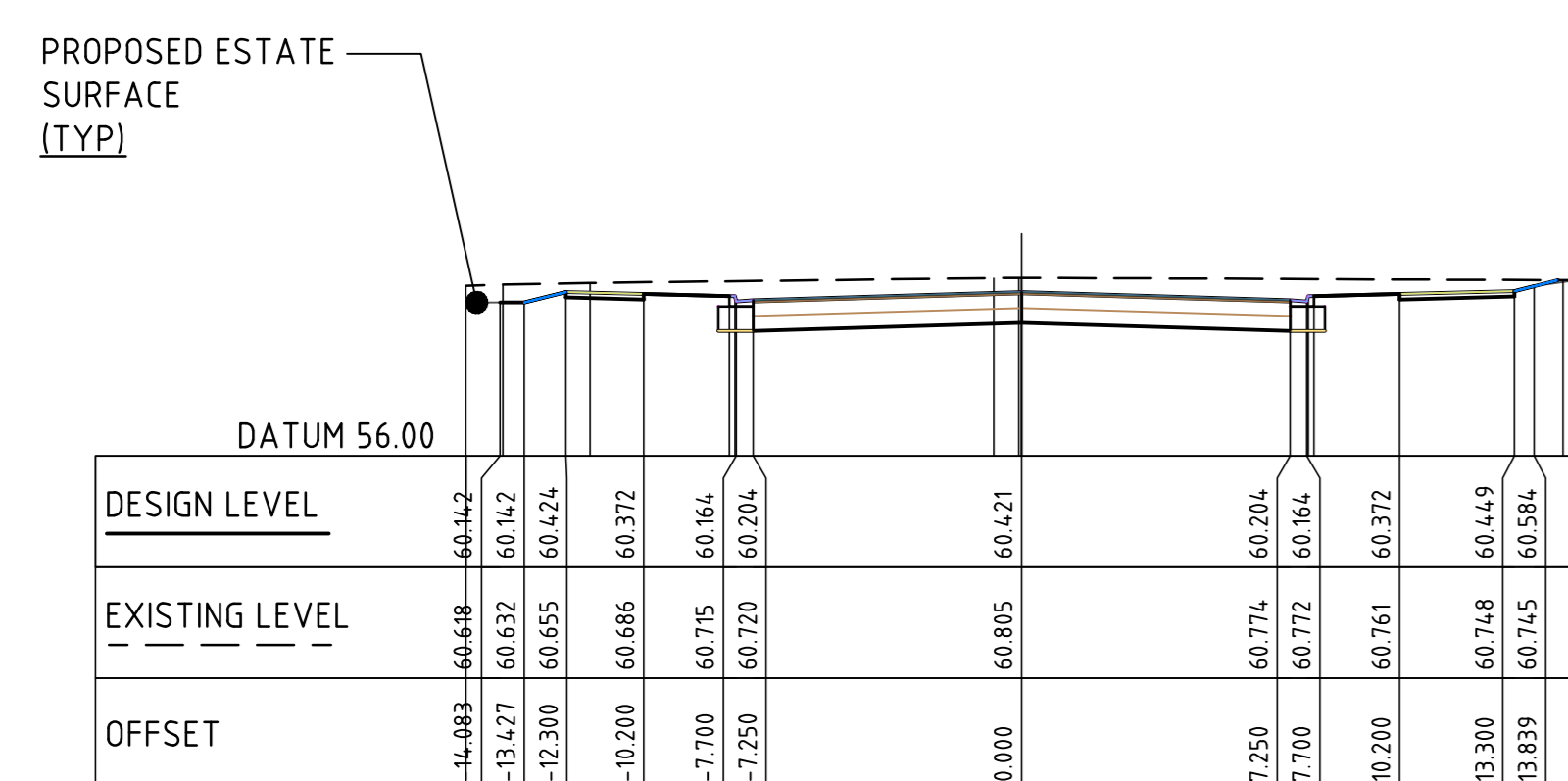
CL DIST RD 1 CH 440.000
