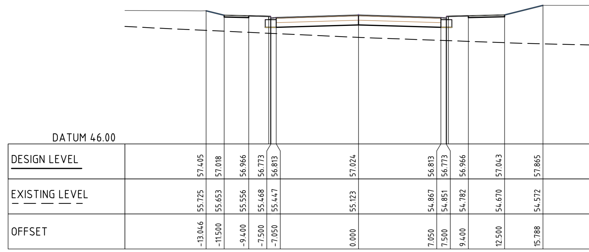
CL IND RD 1 CH 240.000 SCALE 1:200
