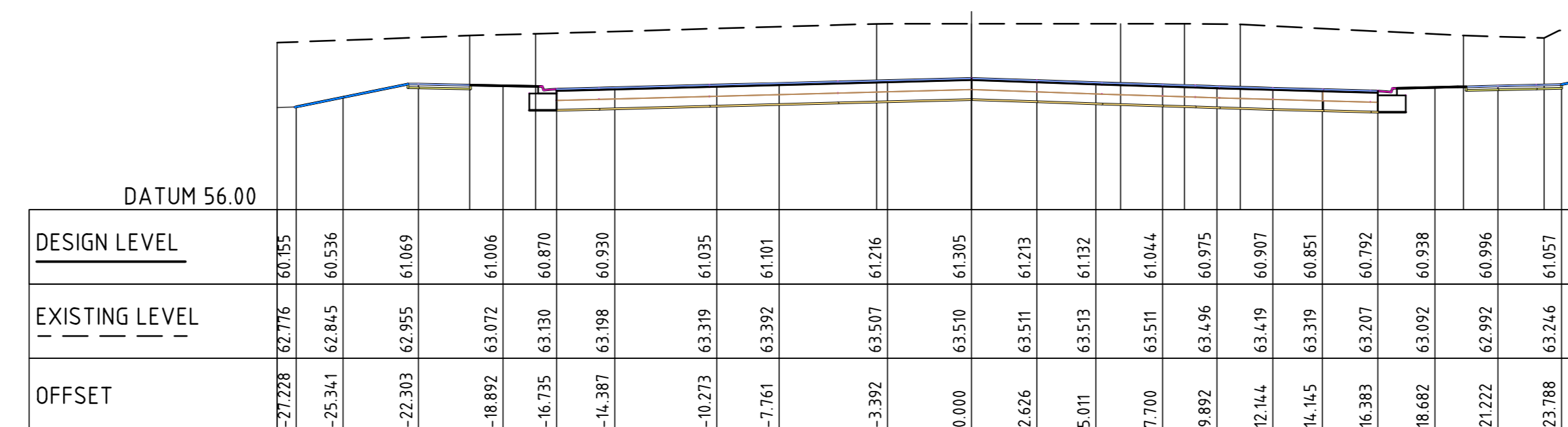
CL DIST RD 1 CH 540.000
