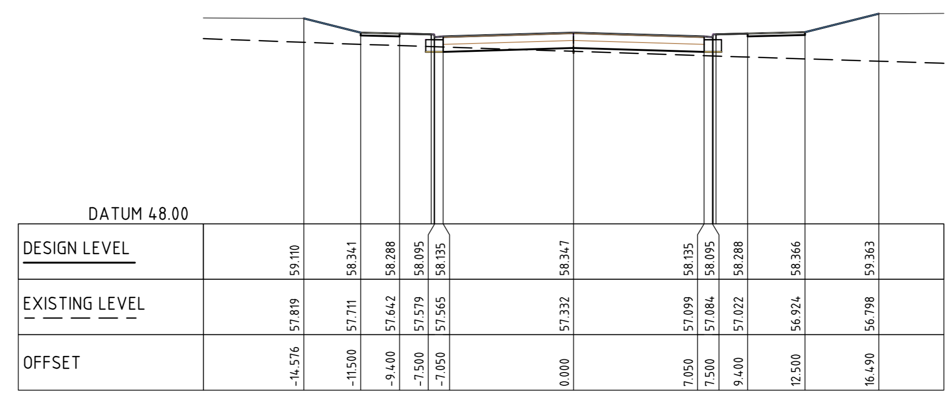
CL IND RD 1 CH 300.000 SCALE 1:200
