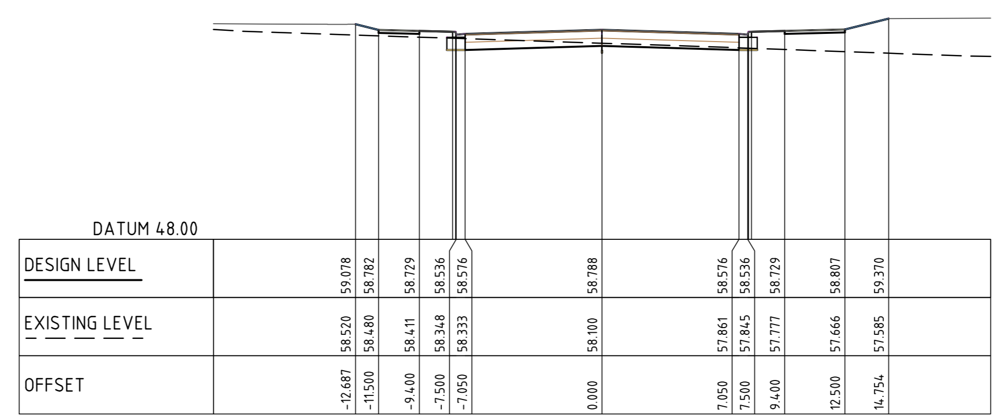
CL IND RD 1 CH 320.000 SCALE 1:200
