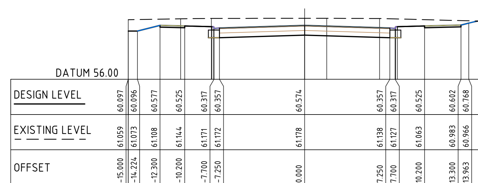
CL DIST RD 1 CH 460.000
