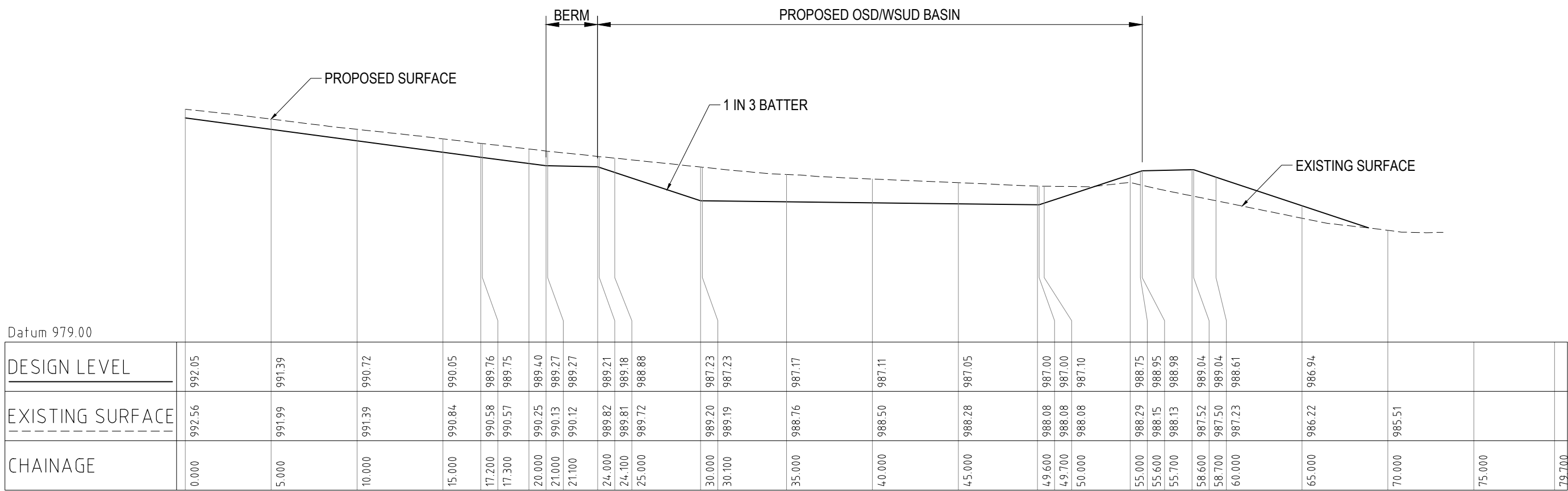
SITE SECTION E 1:250 HORI. 1:250 VERT.
