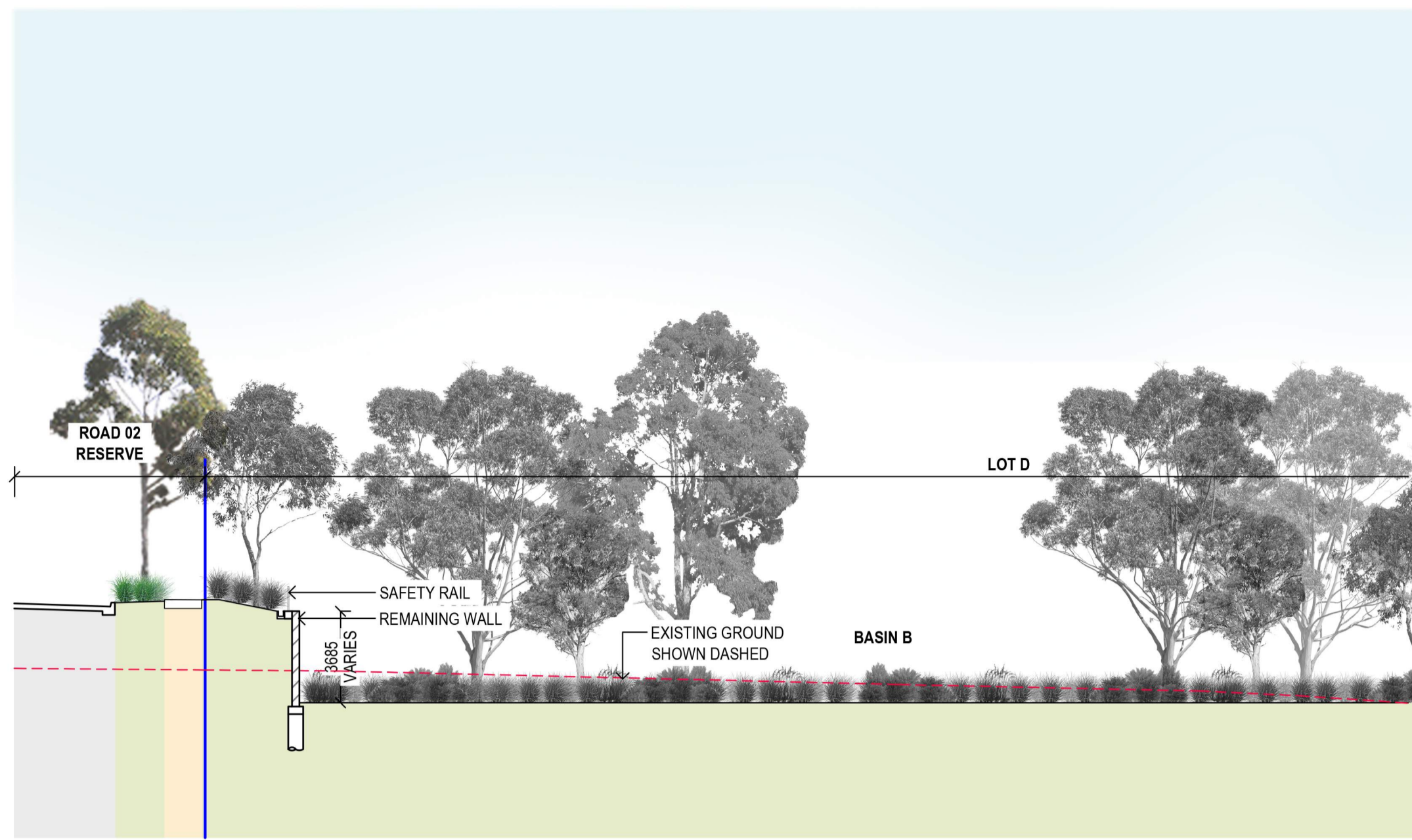
1 SECTION 1 6001 1:200
