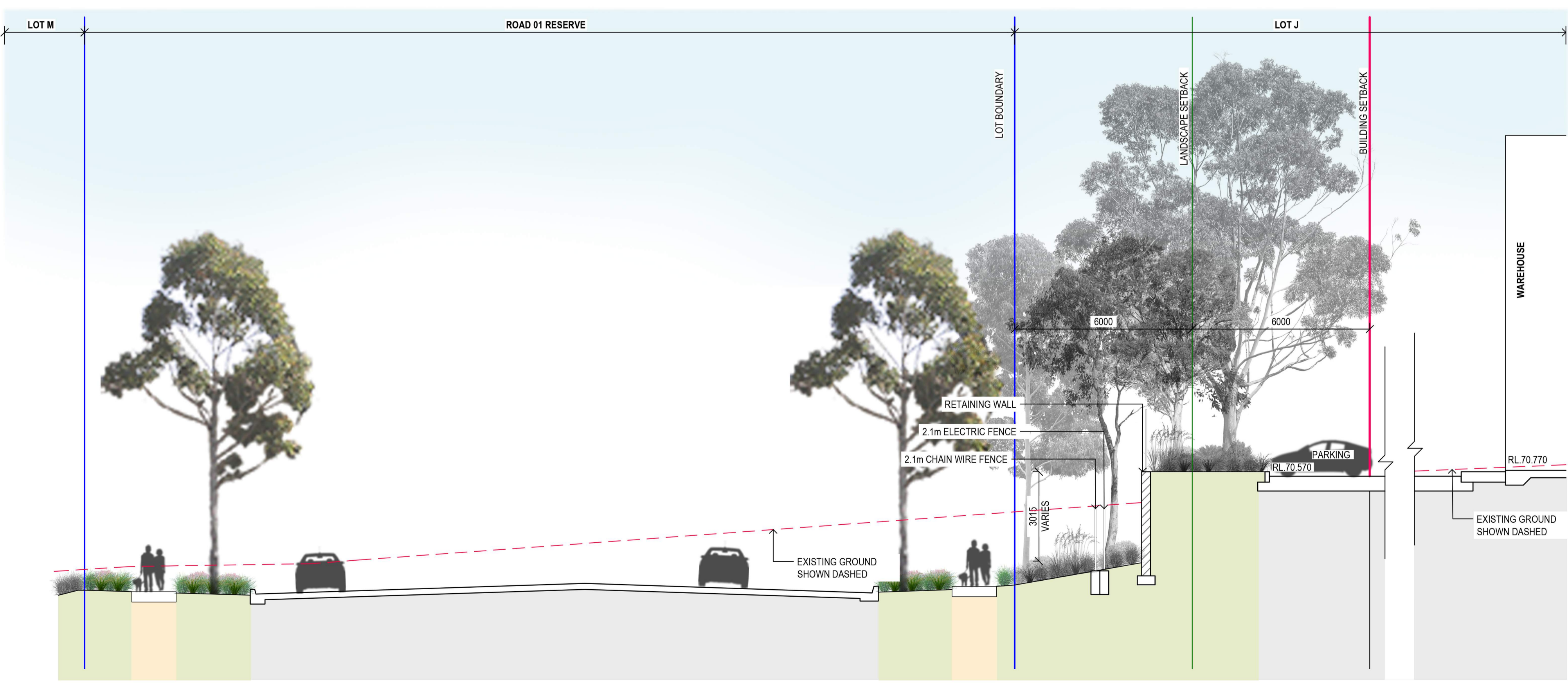
8 SECTION 8 6003 1:100
