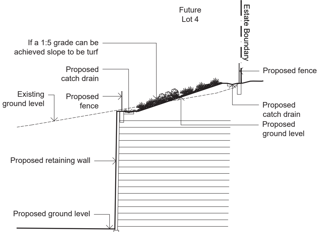
Section E 1:200
