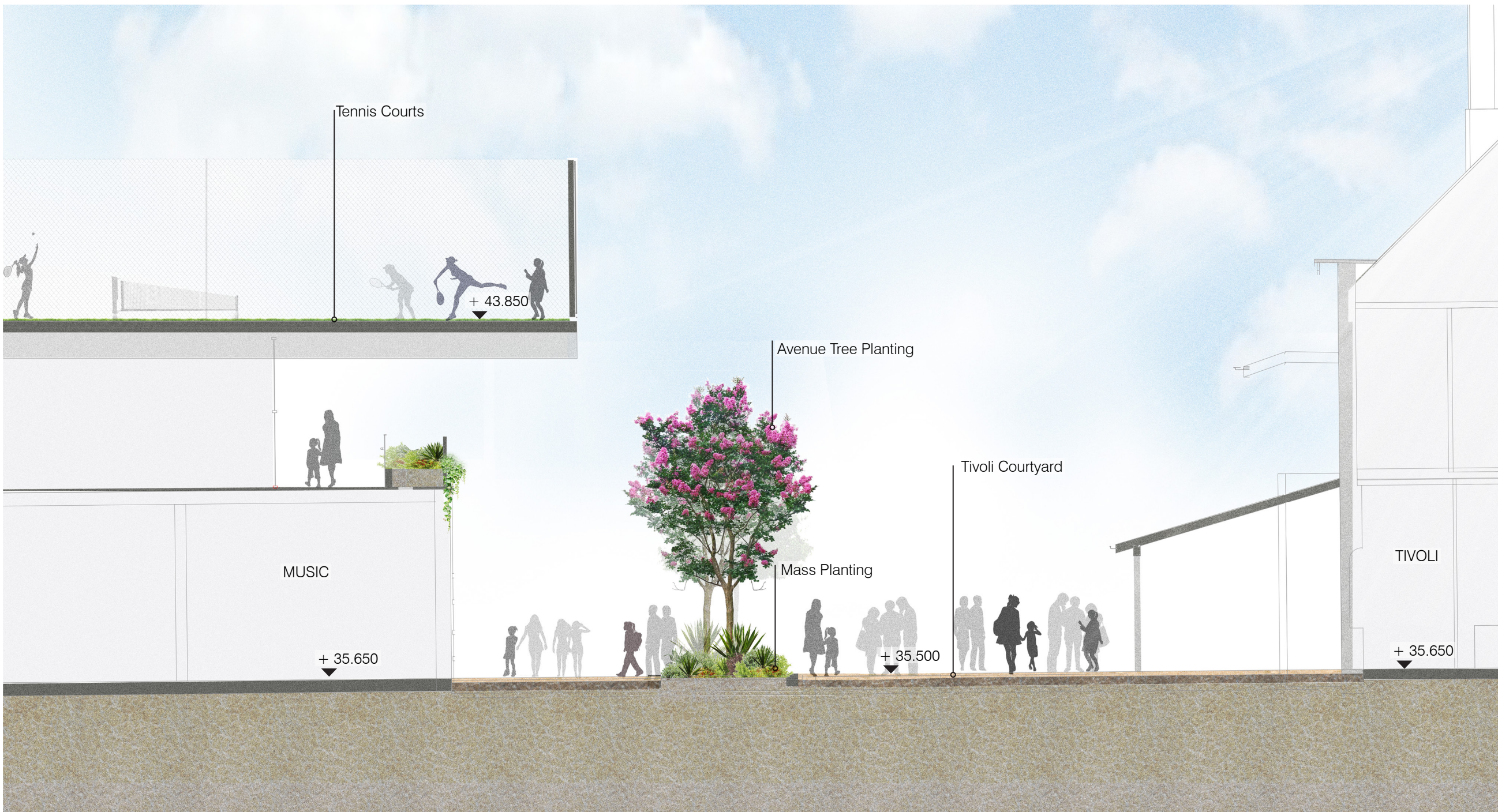
SECTION DD. Tivoli Courtyard SCALE: 1:100
