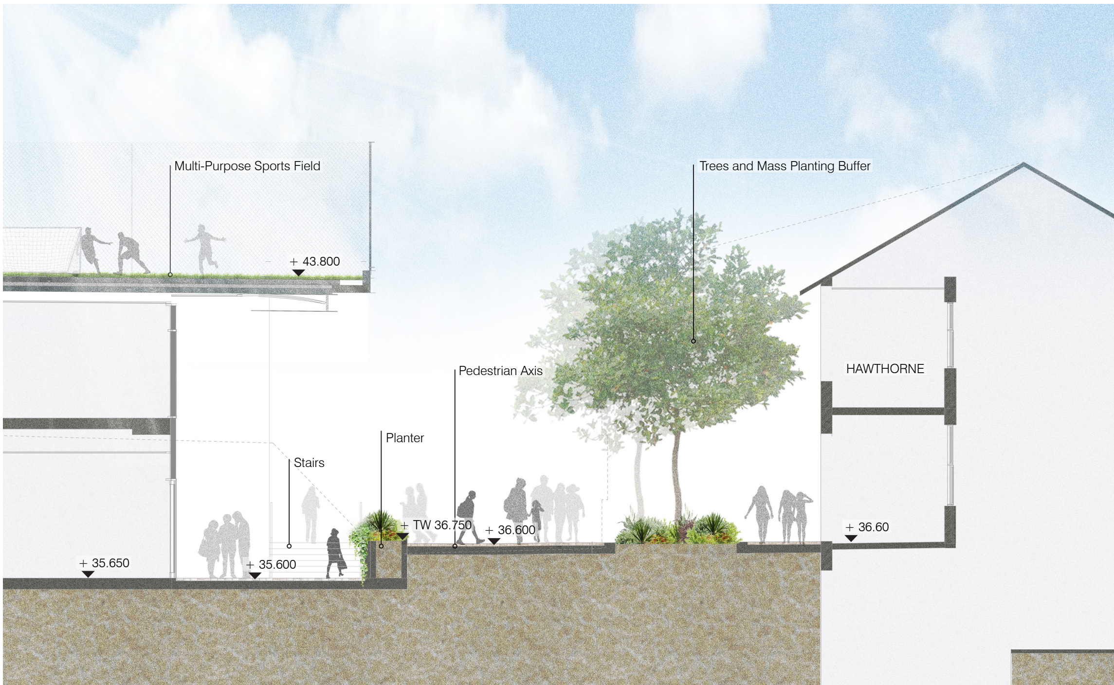
SECTION CC. Pedestrian Axis SCALE: 1:100
