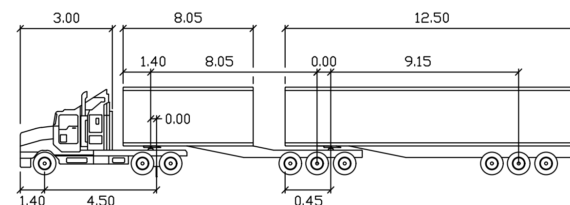
SCALE: 1:500@A1
