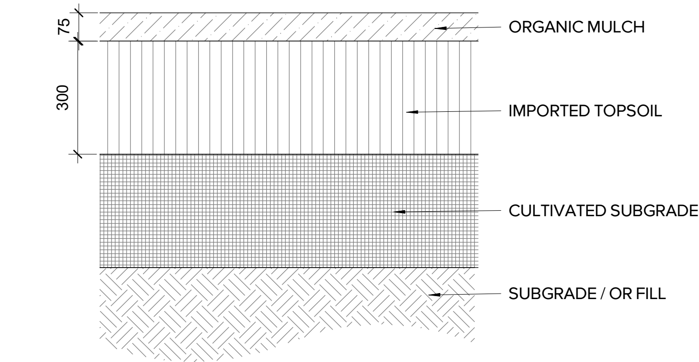
2 PLANTIG - ON GRADE 1 : 10
