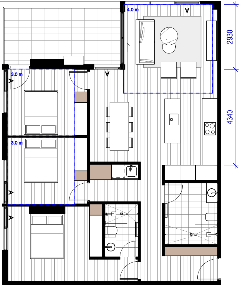
1 3B_6_05_VM SCALE 1 : 100
