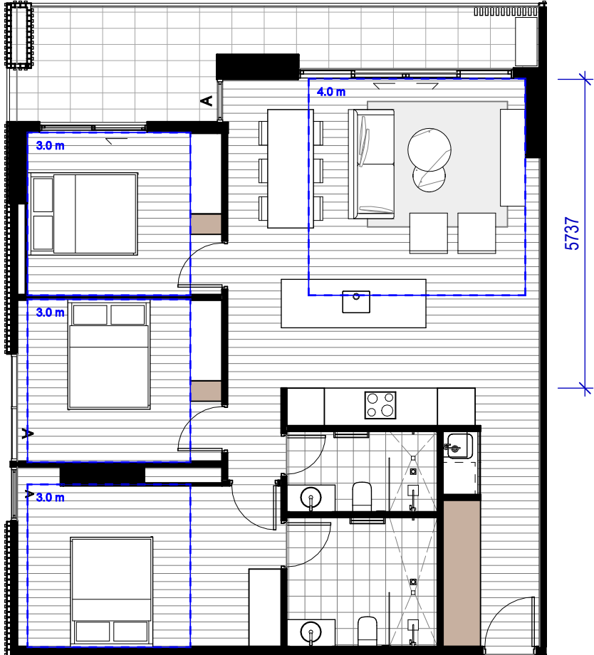
1 3B_7_01_VM SCALE 1 : 100
