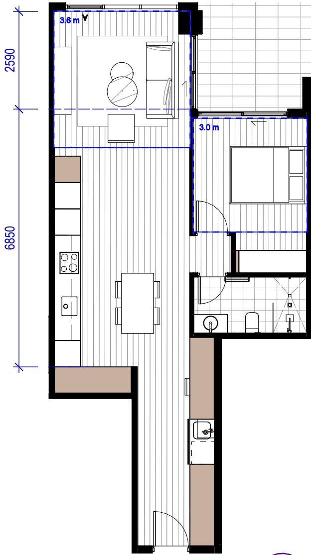
1 1B_2_01_VM SCALE 1 : 100
