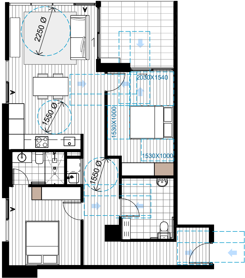
6 2B_4_04_VM Post Adaptable SCALE 1 : 100
