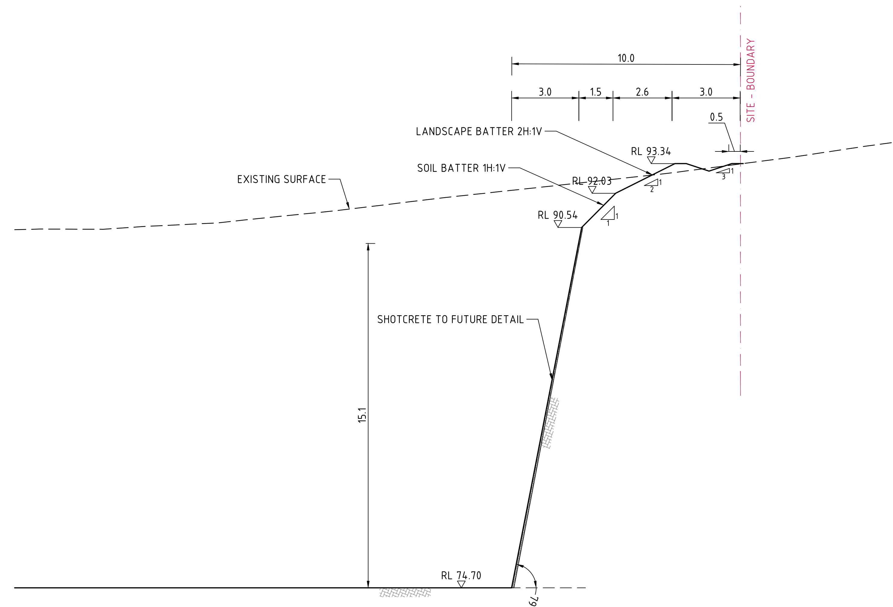
SECTION 1:100 2/600
