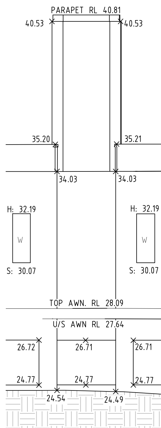
ELEVATION G-G
