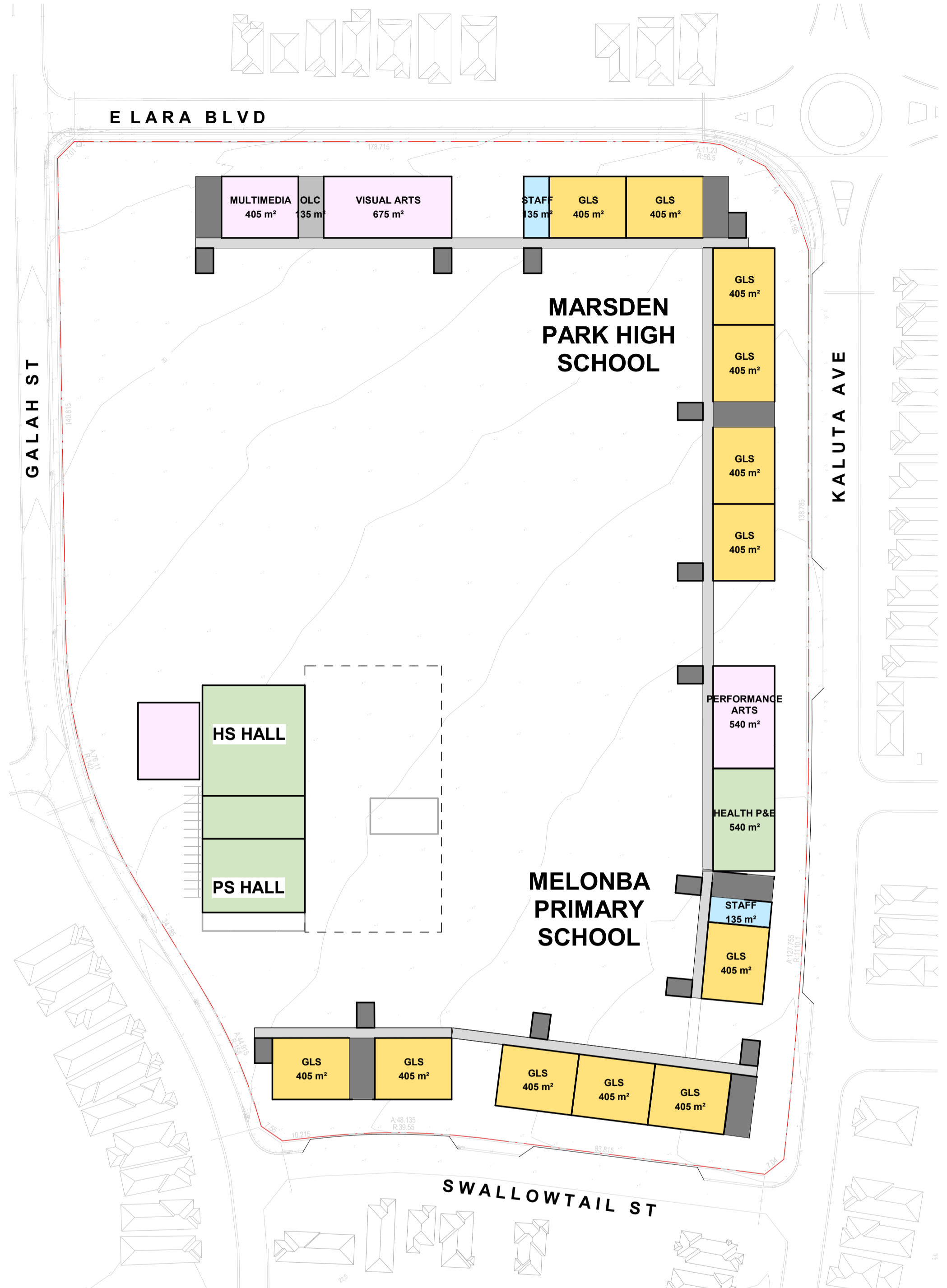
2 LEVEL 1 - OPTION 5 SDRP 1 : 1000
