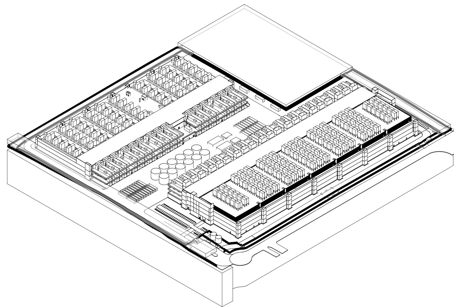
6 SSDA A07 3D - SITE AXONOMETRIC
