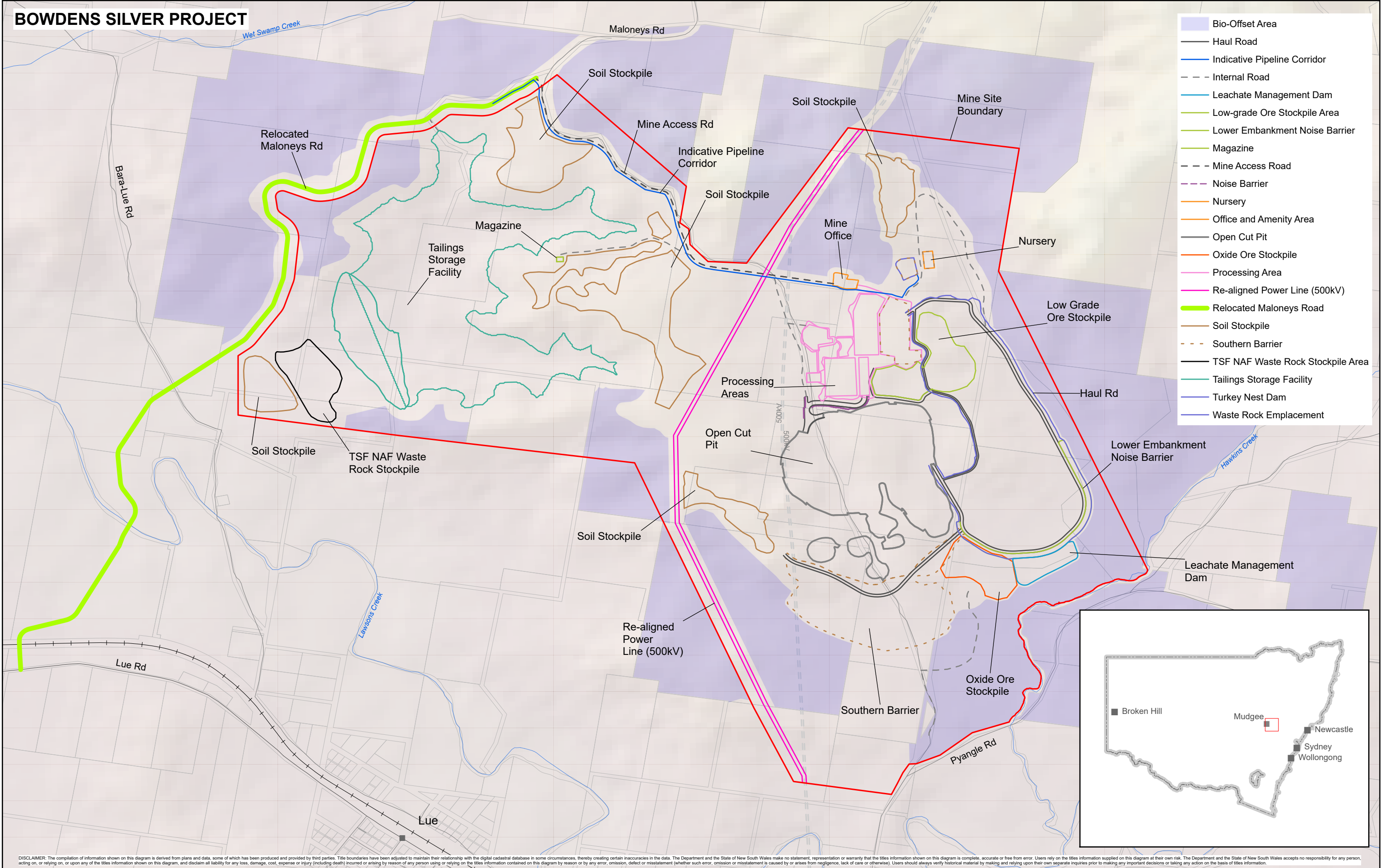
DIAGRAM: SSD 5765 - 1
