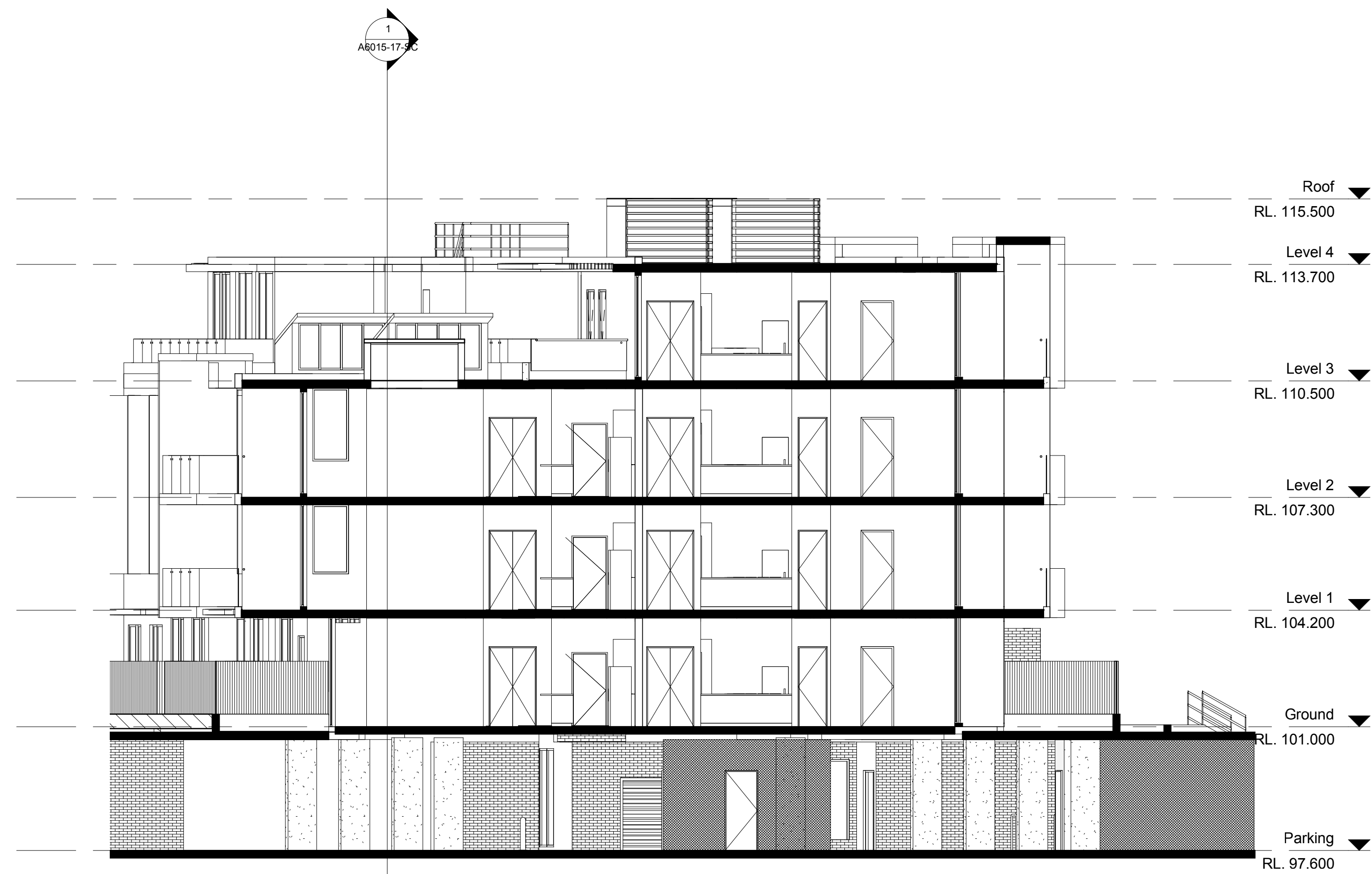
3 Section 2 1 : 100
