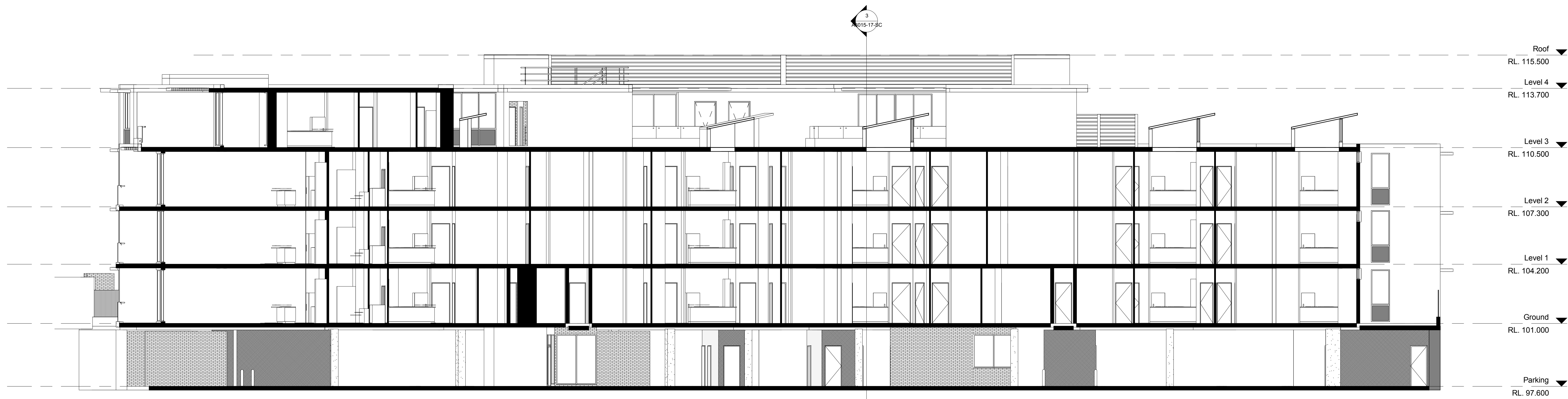
1 Section 3 1 : 100
