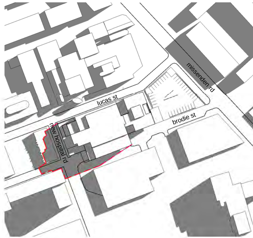
SHADOW STUDY - EQUINOX - 9AM
