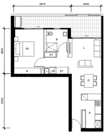
9 DETAIL PLAN BLDG D - Apartment Type 12-A Pre Adaption Layout 1:100 D.1.01 D.7.01 D.10.01 D.13.01 D.16.01 D.2.01 D.7.08 D.10.08 D.13.08 D.16.08 D.3.01 D.8.01 D.11.01 D.14.01 D.17.01 D.4.01 D.8.08 D.11.08 D.14.08 D.17.08 D.5.01 D.9.01 D.12.01 D.15.01 D.18.01 D.6.01 D.9.08 D.12.08 D.15.08 D.18.08
