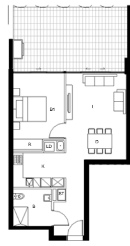
1 DETAIL PLAN BLDG A - Apartment Type 2-A Pre Adaption Layout 1:100 A.1.02 A.4.11 A.08.02 A.11.09 A.1.10 A.5.02 A.08.09 A.12.02 A.2.02 A.5.11 A.09.02 A.12.09 A.2.11 A.6.02 A.09.09 A.13.09 A.3.02 A.6.11 A.10.02 A.14.09 A.3.11 A.7.02 A.10.09 A.15.09 A.4.02 A.7.09 A.11.02
