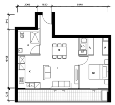
1 DETAIL PLAN BLDG A - Apartment Type 2-A Pre Adaption Layout 1:100 A.1.02 A.4.11 A.08.02 A.11.09 A.1.10 A.5.02 A.08.09 A.12.02 A.2.02 A.5.11 A.09.02 A.12.09 A.2.11 A.6.02 A.09.09 A.13.09 A.3.02 A.6.11 A.10.02 A.14.09 A.3.11 A.7.02 A.10.09 A.15.09 A.4.02 A.7.09 A.11.02
