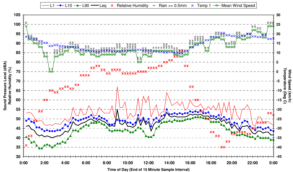
Statistical Ambient Noise Levels 135 Croatia Av Edmonson Park - Monday 24 April 2006
