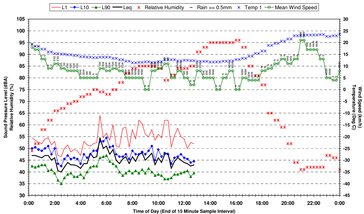
Statistical Ambient Noise Levels 135 Croatia Av Edmonson Park - Saturday 29 April 2006
