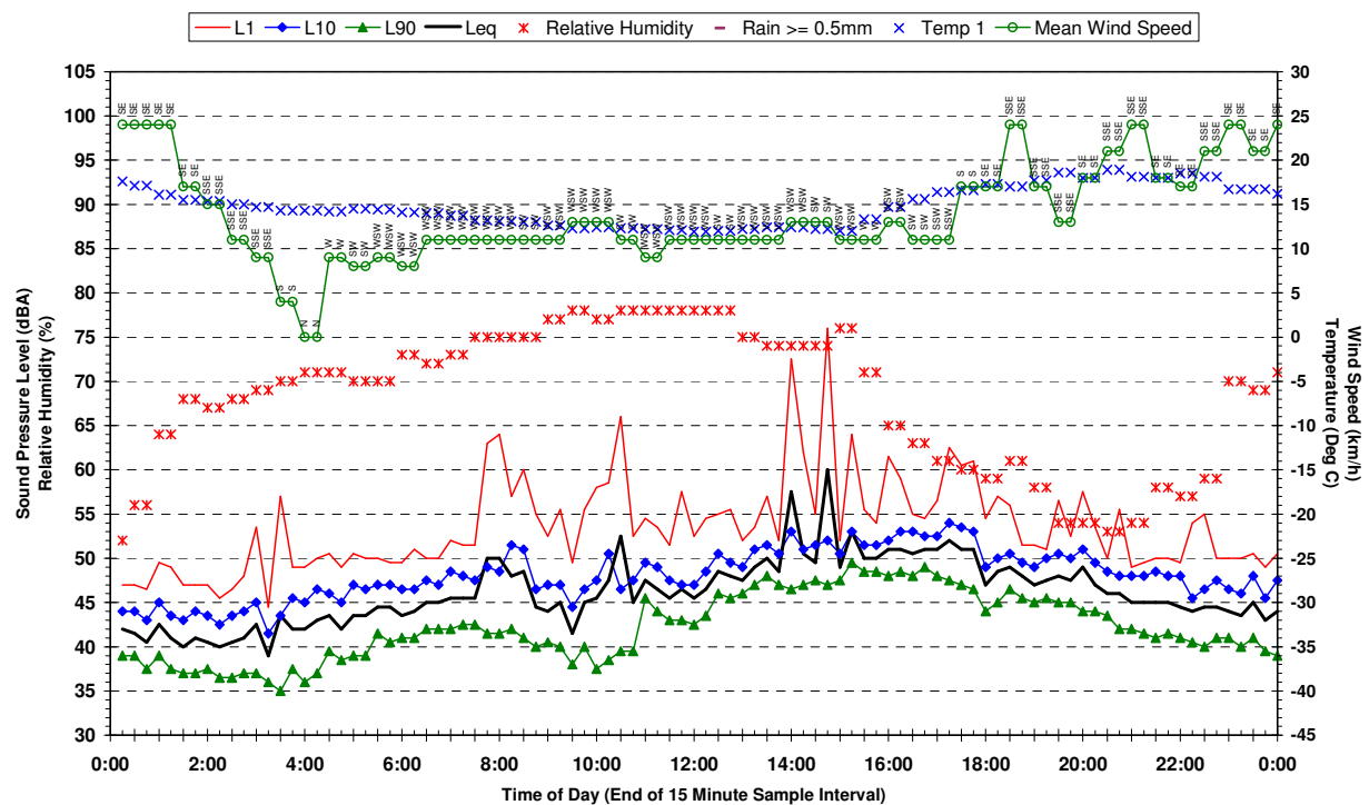
Statistical Ambient Noise Levels 135 Croatia Av Edmonson Park - Tuesday 25 April 2006
