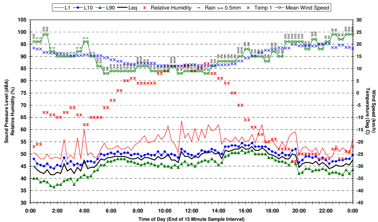
Statistical Ambient Noise Levels 135 Croatia Av Edmonson Park - Thursday 27 April 2006
