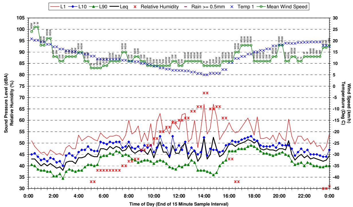
Statistical Ambient Noise Levels 135 Croatia Av Edmonson Park - Saturday 22 April 2006
