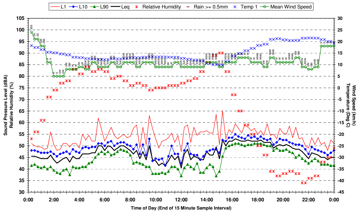
Statistical Ambient Noise Levels 135 Croatia Av Edmonson Park - Friday 28 April 2006
