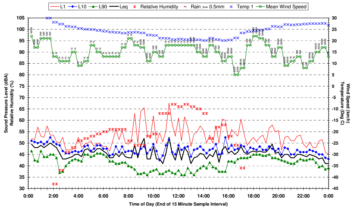
Statistical Ambient Noise Levels 135 Croatia Av Edmonson Park - Thursday 20 April 2006
