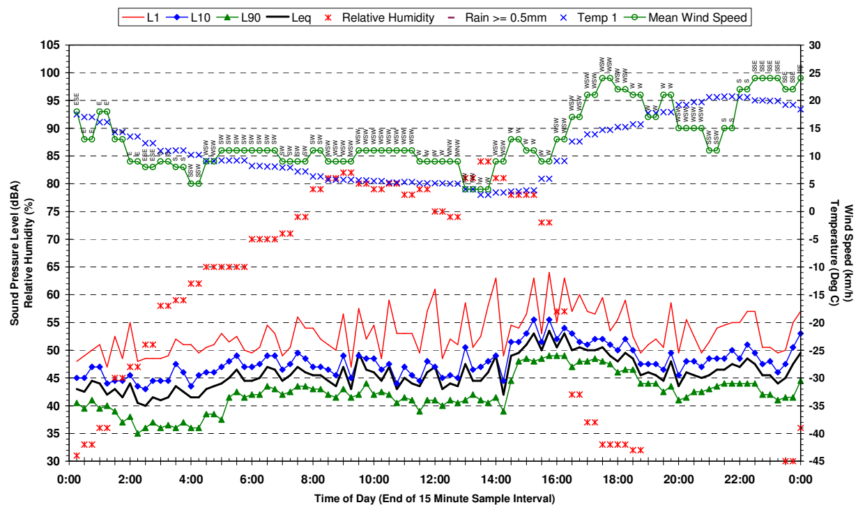
Statistical Ambient Noise Levels 135 Croatia Av Edmonson Park - Sunday 23 April 2006
