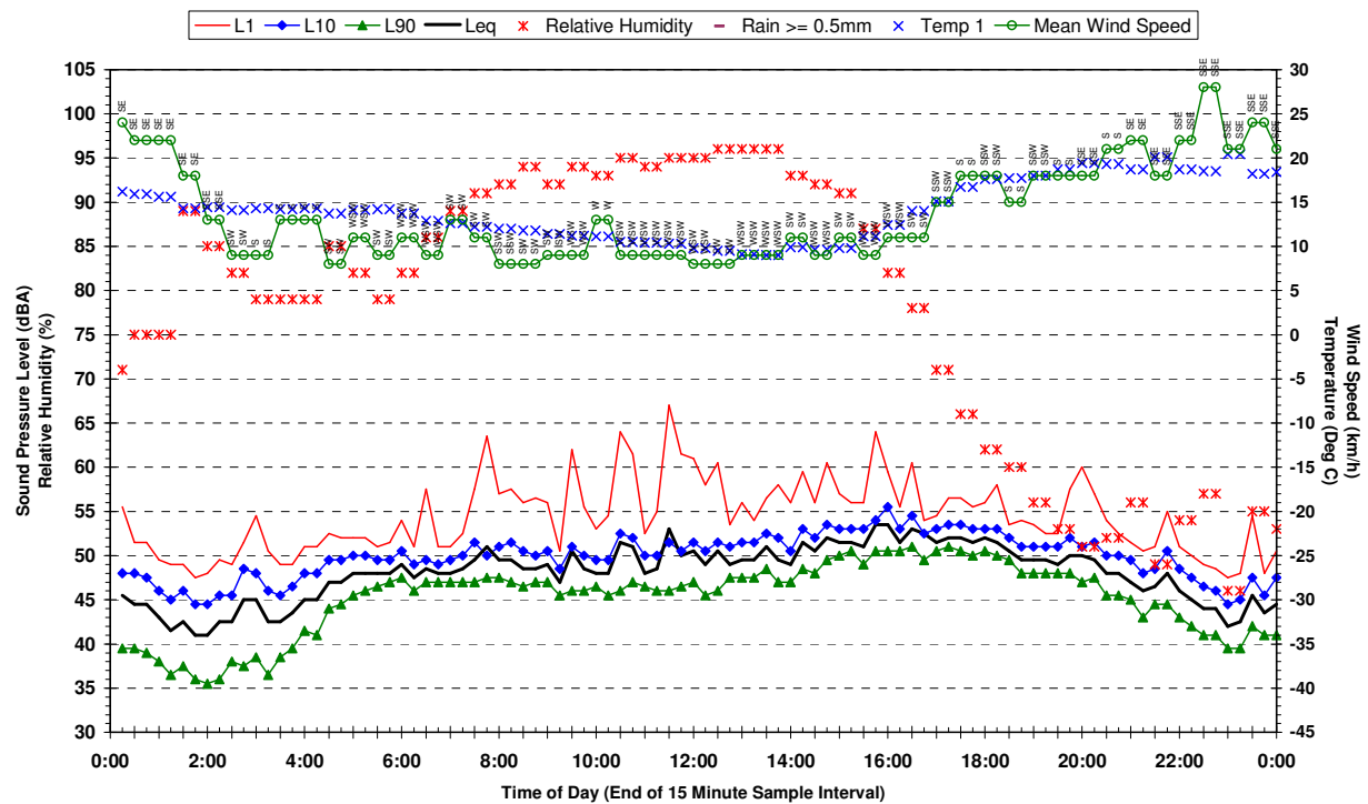
Statistical Ambient Noise Levels 135 Croatia Av Edmonson Park - Wednesday 26 April 2006
