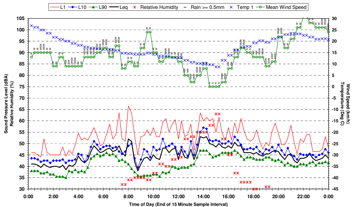
Statistical Ambient Noise Levels 135 Croatia Av Edmonson Park - Friday 21 April 2006
