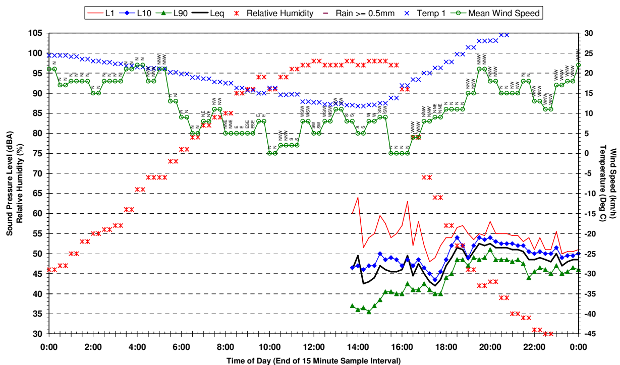
Statistical Ambient Noise Levels 135 Croatia Av Edmonson Park - Wednesday 19 April 2006
