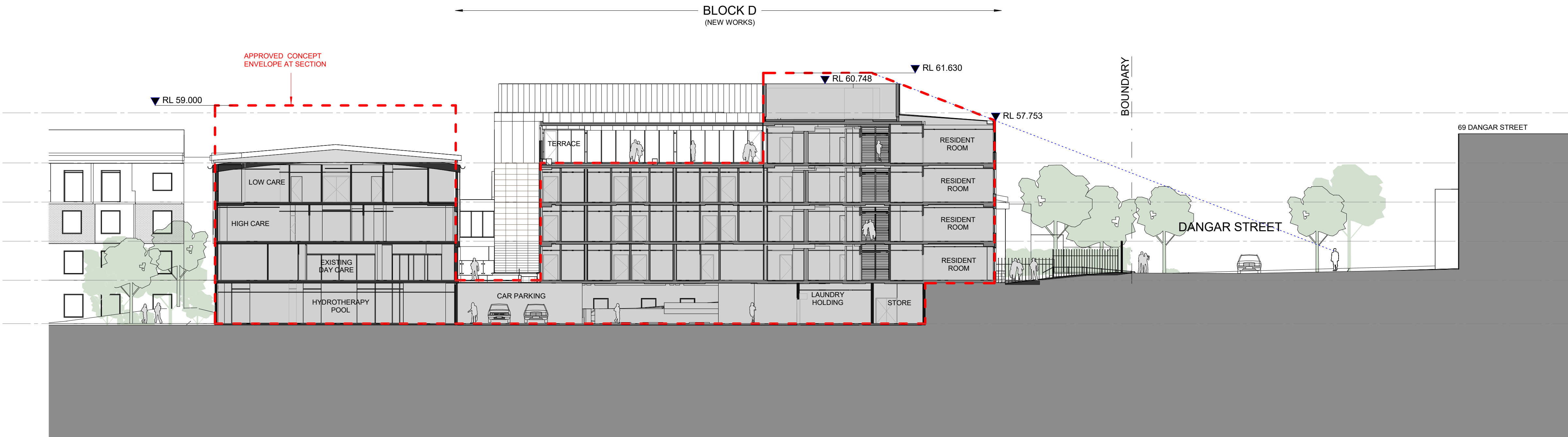
1 SECTION 1 : 200
