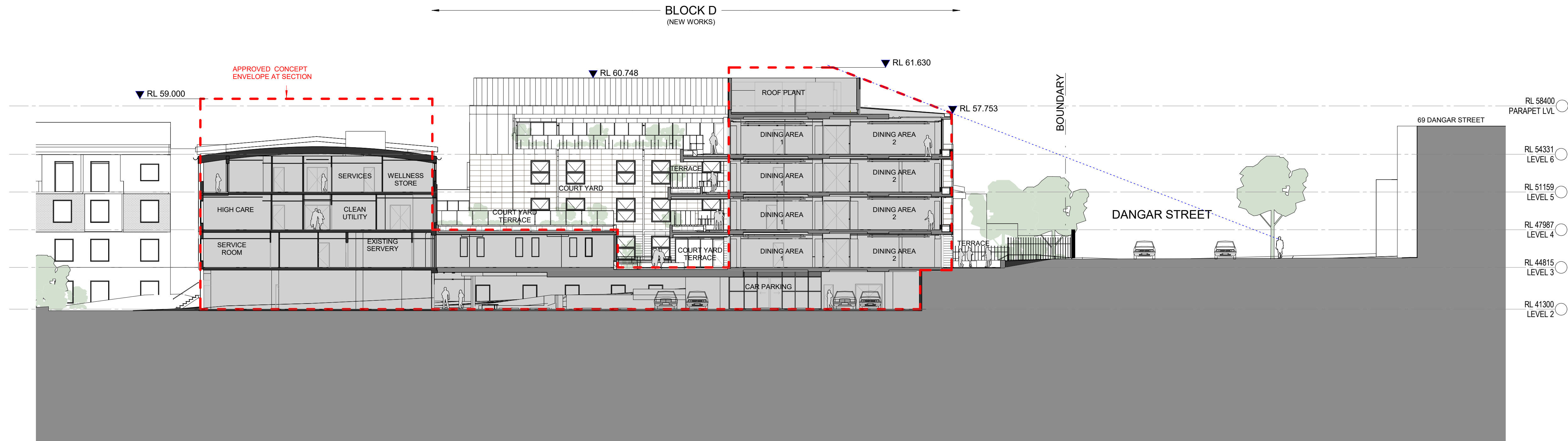
2 SECTION 1 : 200
