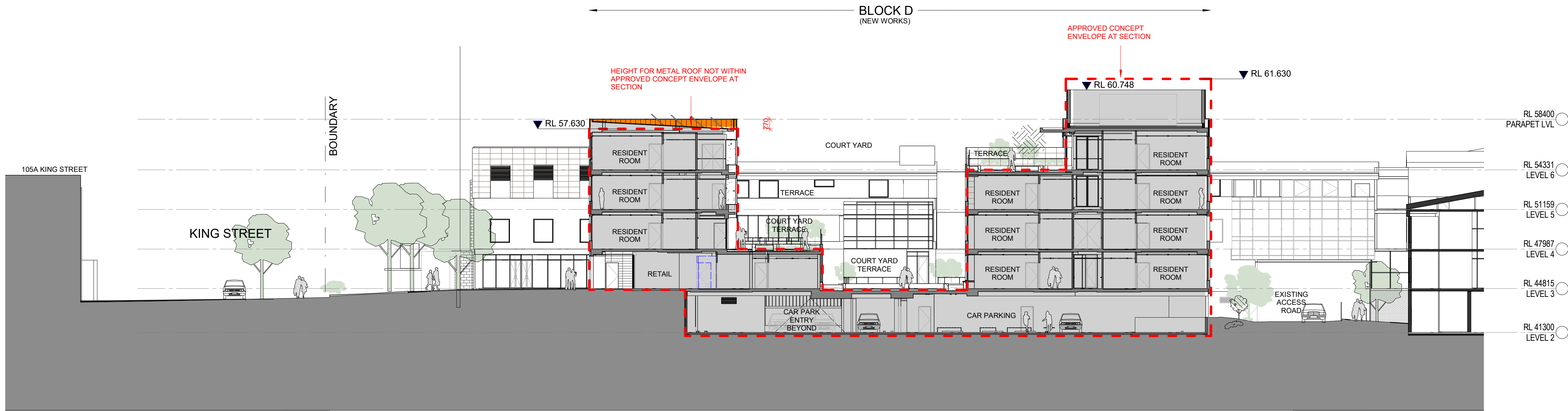
1 SECTION 1 : 200
