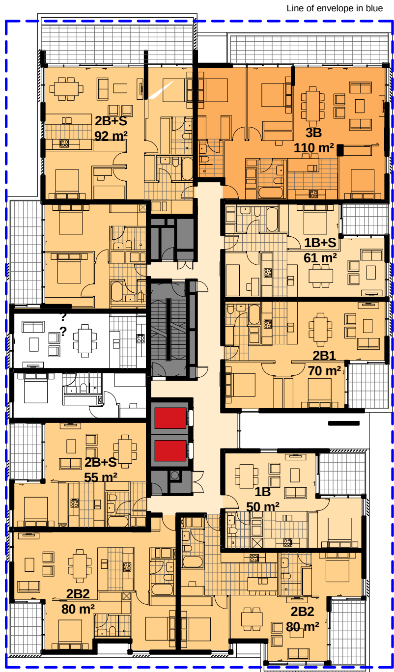
3 Level 07 - 08 DA2.203 1 : 250
