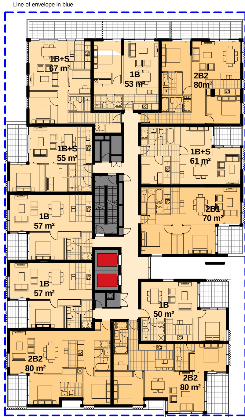
2 Level 05 - 06 DA2.203 1 : 250
