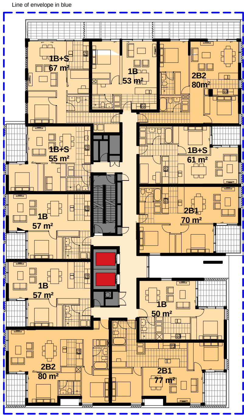
1 Level 03 - 04 DA2.203 1 : 250
