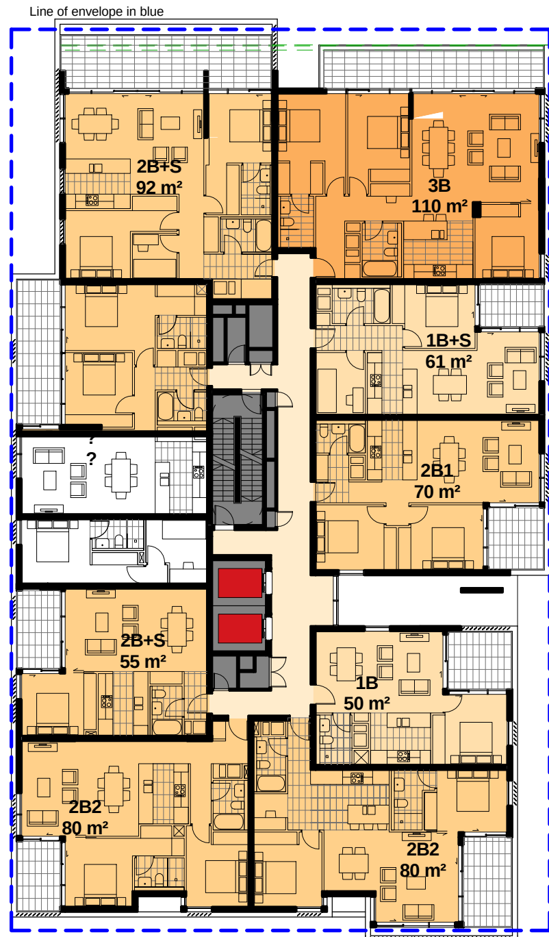
4 Level 09 - 10 DA2.203 1 : 250
