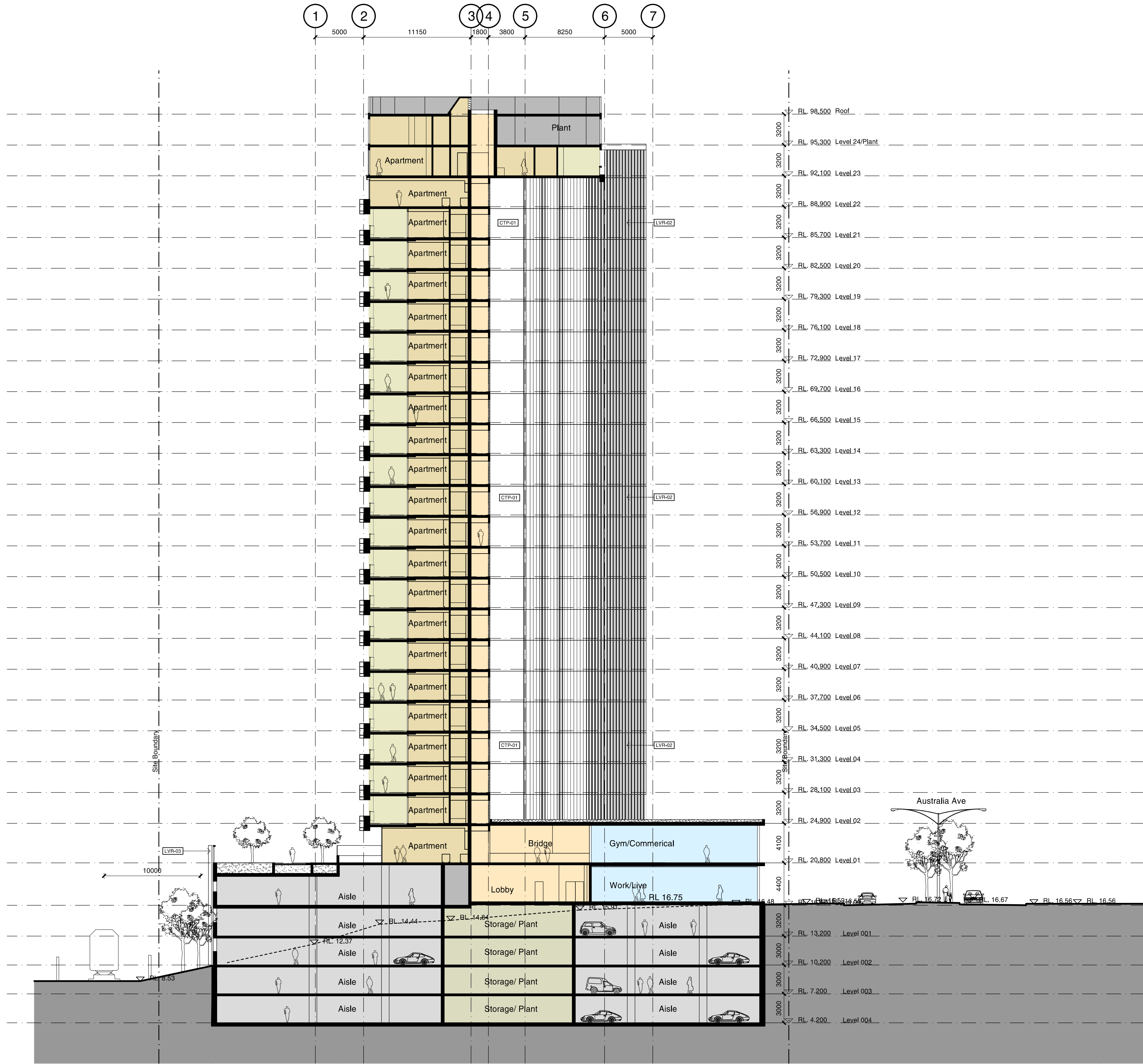
1 Section BB 1:250
