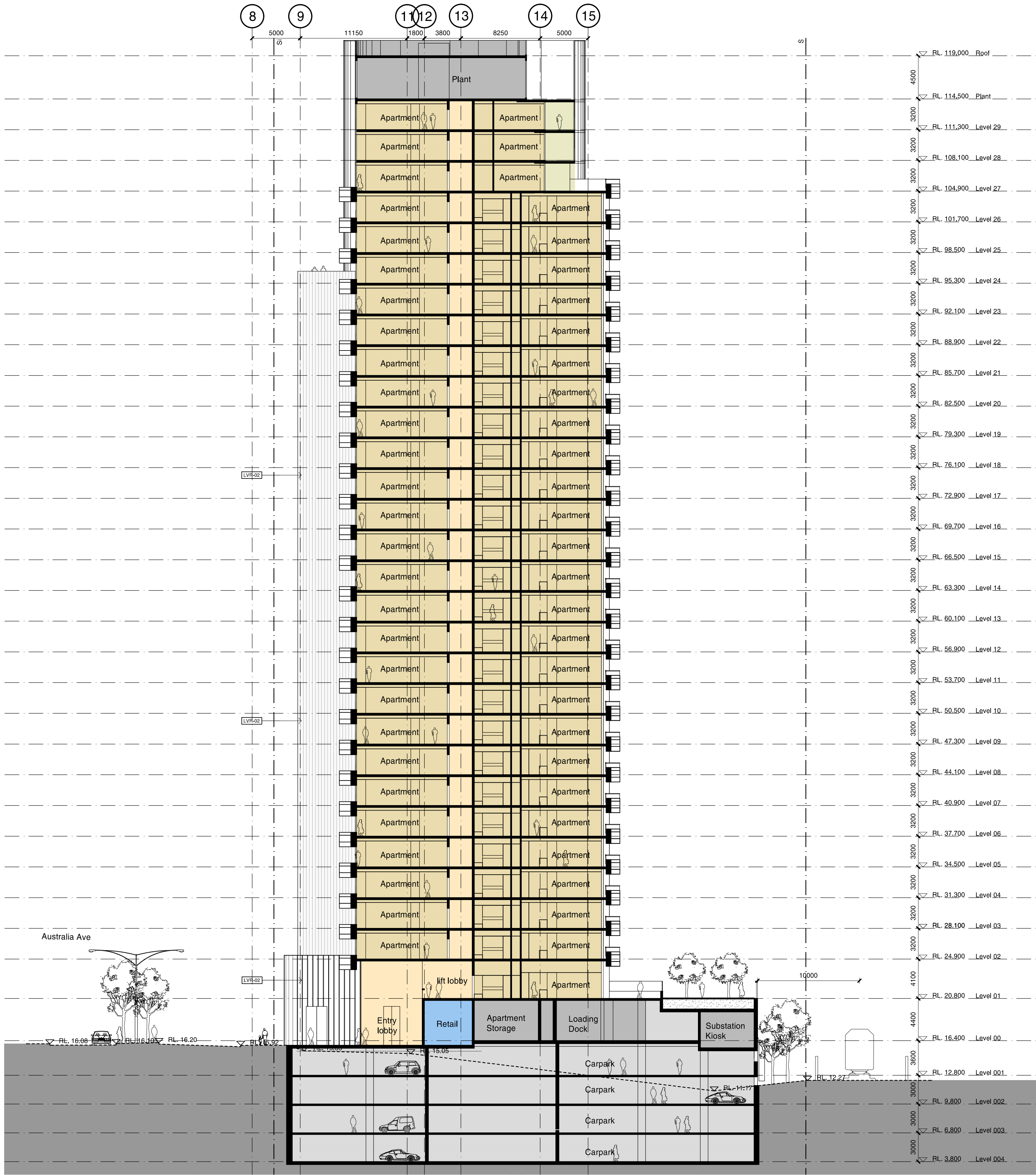
1 Section DD 1:250
