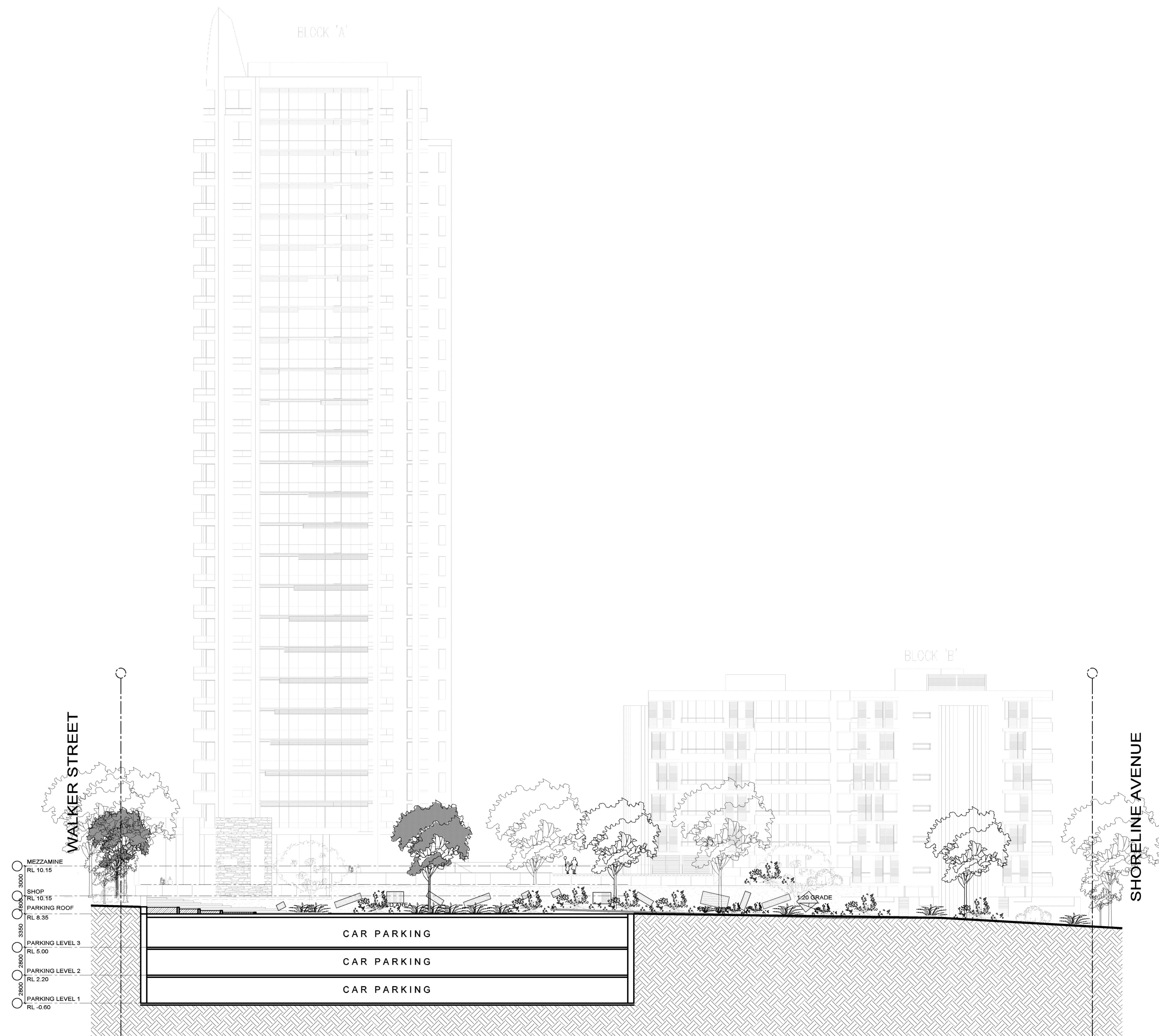
SITE SECTION D-D SCALE 1:200
